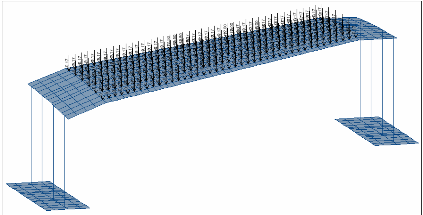
Figura 3.10 Fuerzas variables debidas a la carga viva IMT 66.5 en los carriles de circulación del tramo central (VI C )
