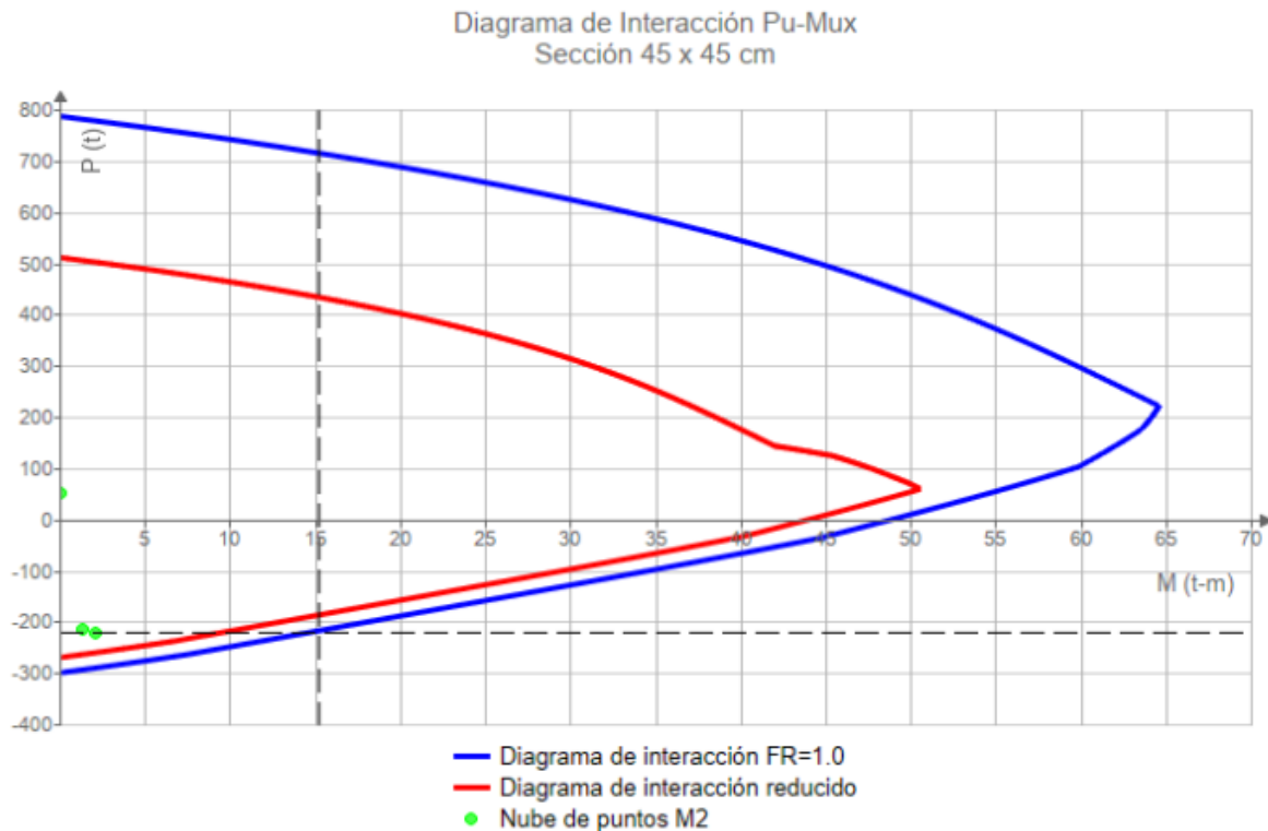
Imagen 6.3.6 Resistencia nominal a flexión de la sección de columna. Fuente: elaboración propia.
