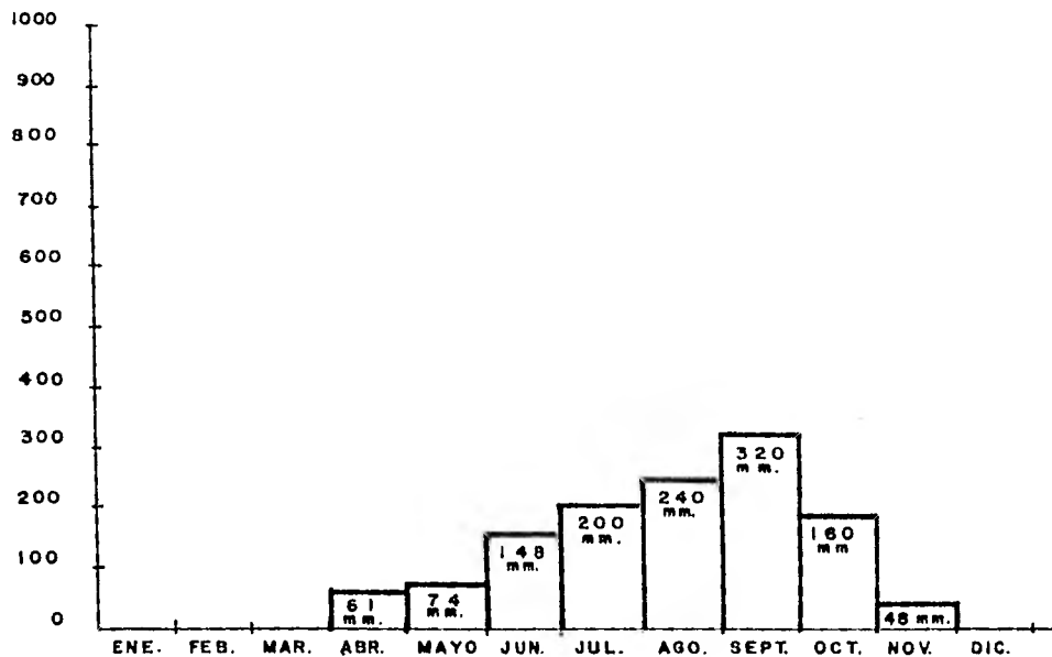
FIG. 3 PRECIPITACION PLUVIAL EN EL MUNICIPIO LA UNION GRO. EN EL AÑO 1979 (9)
