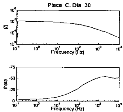
Placa (C), con convertidor de óxido después de 30 días
