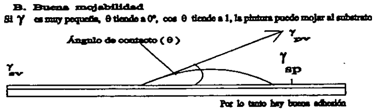
Fig. 4 Contacto de la pintura con el sustrato. A. Existe una pobre adhesión. B. Existe buena adhesión
