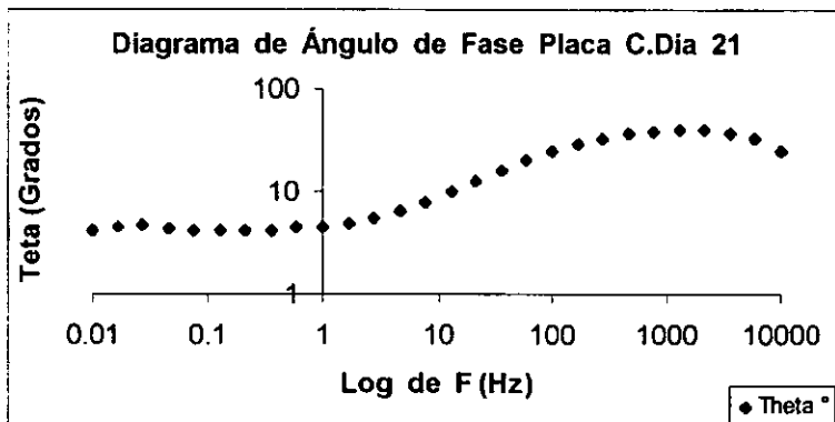
Figura 3.2.3. Placa c en inmersión después de 21 días
