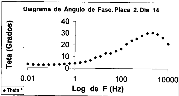
Figura 3.2.6. Placa 2 en inmersión después de 14 días.
