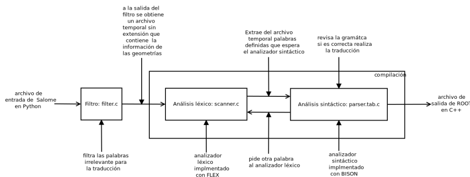
Figura 4.3. Arquitectura de salomeToROOT.
