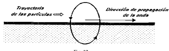
Imagen 2.2-6: Ondas Rayleigh. ( www.lpi.tel.uva.es/ , s.f.)
