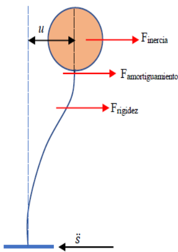
Imagen 5.1-1: Sistema de 1GL
