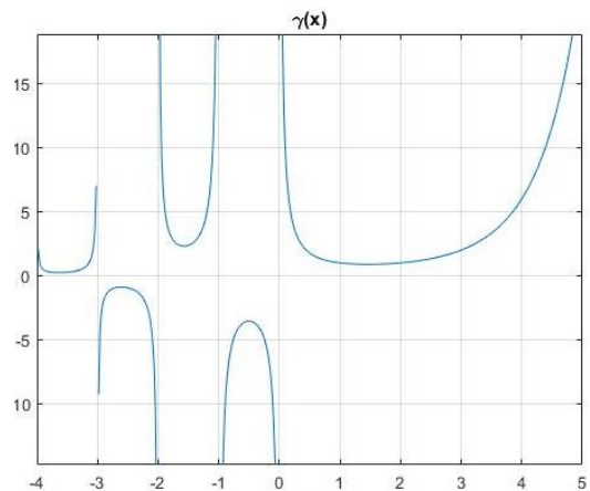
Imagen 3.2-1: Gráfica de la función Gamma
