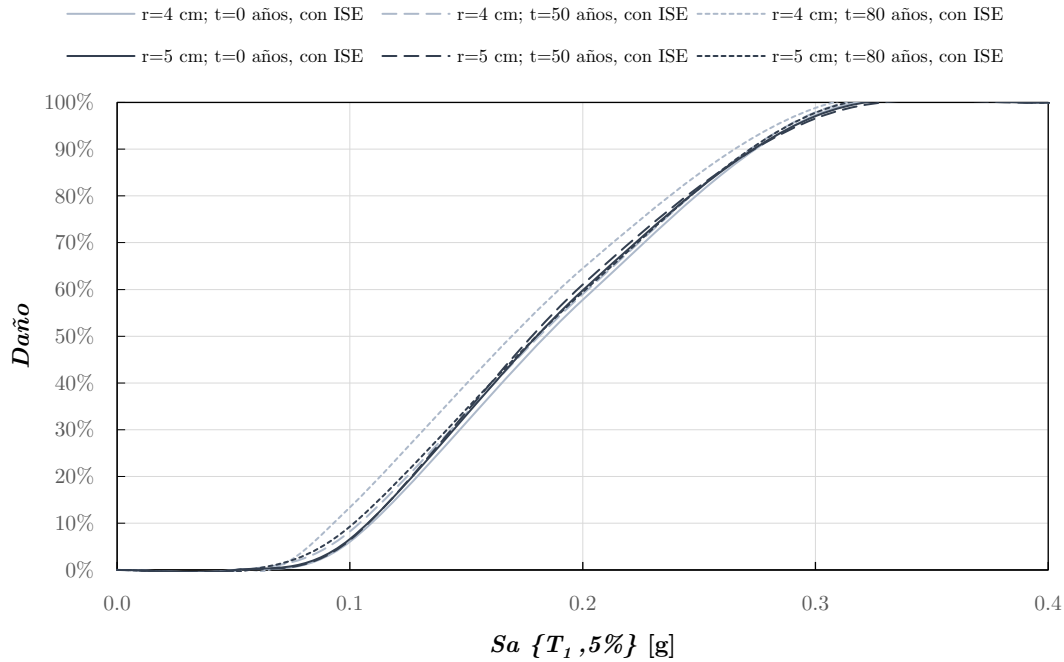
Figura 51. Funciones de vulnerabilidad de las estructuras 7N-3×2C, tomando en cuenta, de manera conjunta, los efectos del intemperismo y de la interacción suelo-estructura
