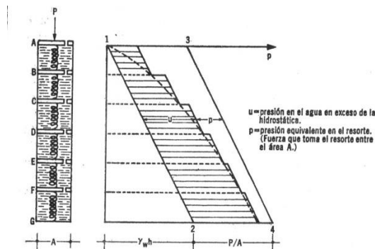
Figura X-8. Esquema del modelo de Terzaghi, comprendiendo varias cámaras.
