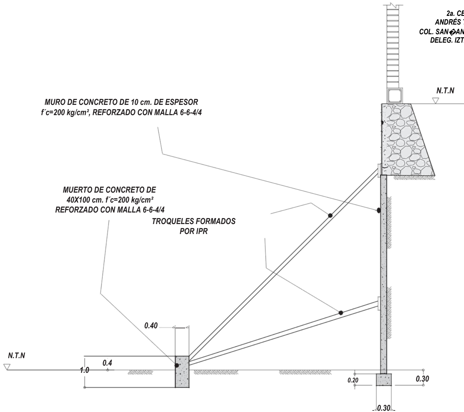
MURO DE CONTENCIÓN HACIA COLINDANCIAS
