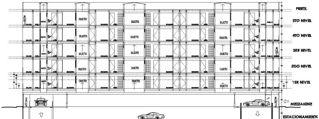
CORTE VERTICAL LONGITUDINAL
