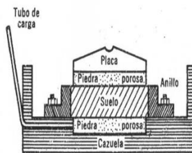
Figura X-2. Detalle de la colocación de la muestra en el consolidómetro de anillo fijo.
