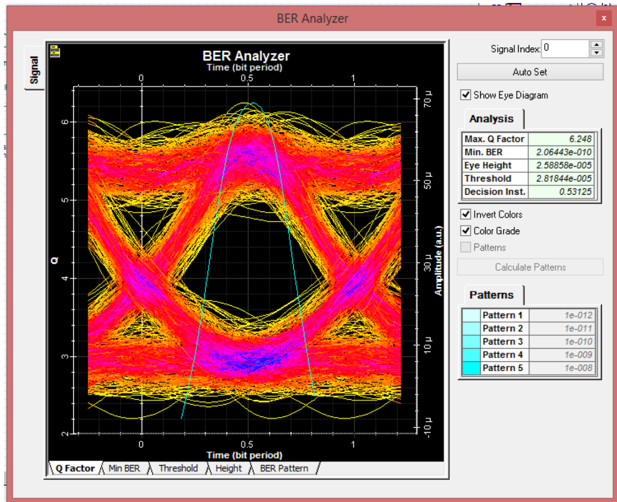
Figura 34. BER del enlace de "Emiliano Zapata - Vicente Guerrero". Fuente: Elaboración propia utilizando el software Optisystem™ (2023).
