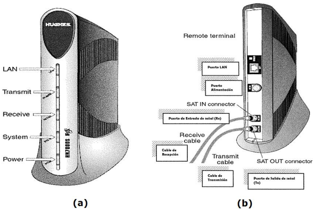
Figura 51. Indicadores de conexión para instalación de un modem satelital (modelo HN7000S).
