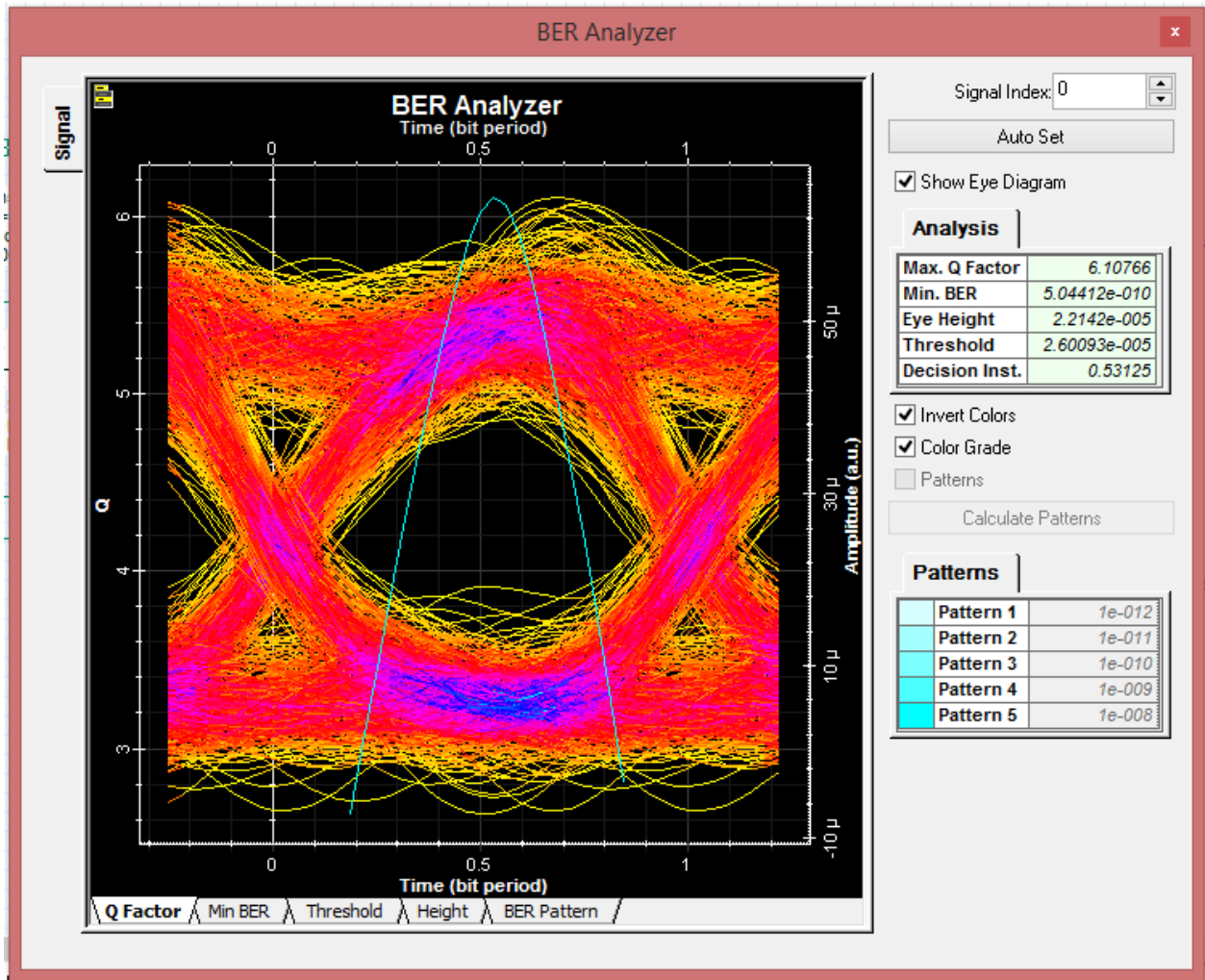
Figura 38. Segundo BER del enlace "Rosario-Cataviña".
