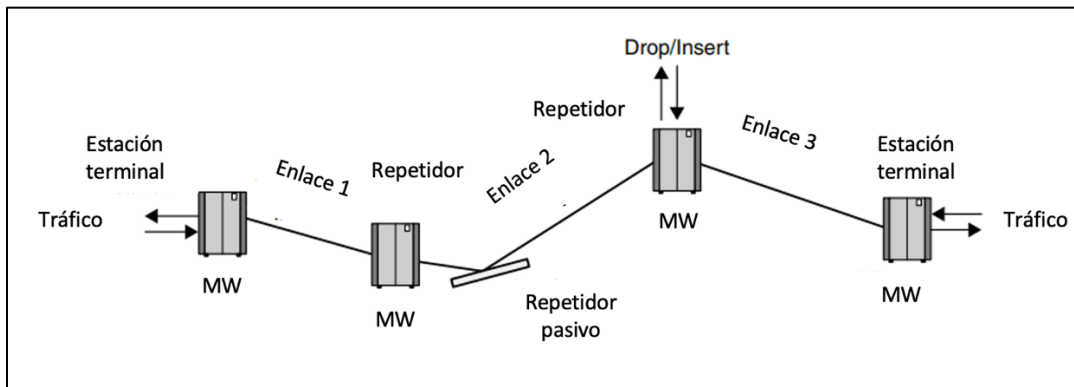
Figura 13. Radioenlace con repetidores.
