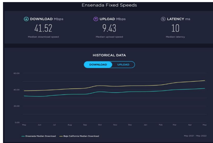
Figura 6. Tasas de transmisión downlink promedio en Ensenada, banda ancha fija.
