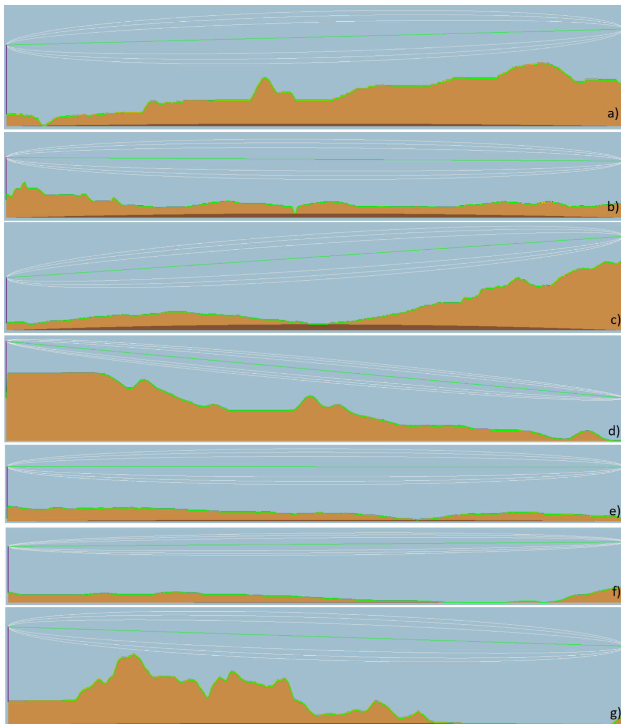
Figura 48. Propuesta de enlaces para la provisión de internet en campo "La Costilla."
