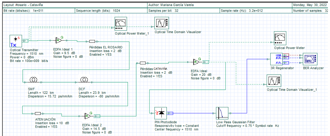
Figura 29. Diagrama de simulación de enlace de fibra óptica en el software OptiSystem para el enlace "Ejidos Nueva Odisea – Rosario - Cataviña".
