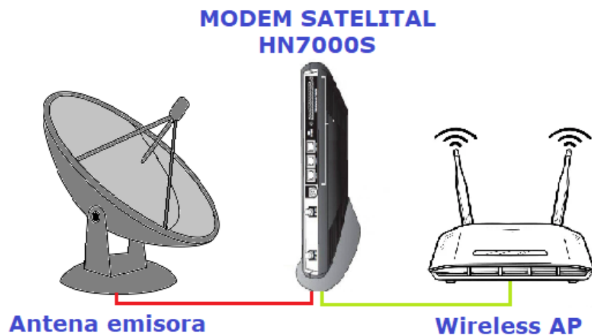
Figura 50. Diagrama de Conexión para estación terrena.
