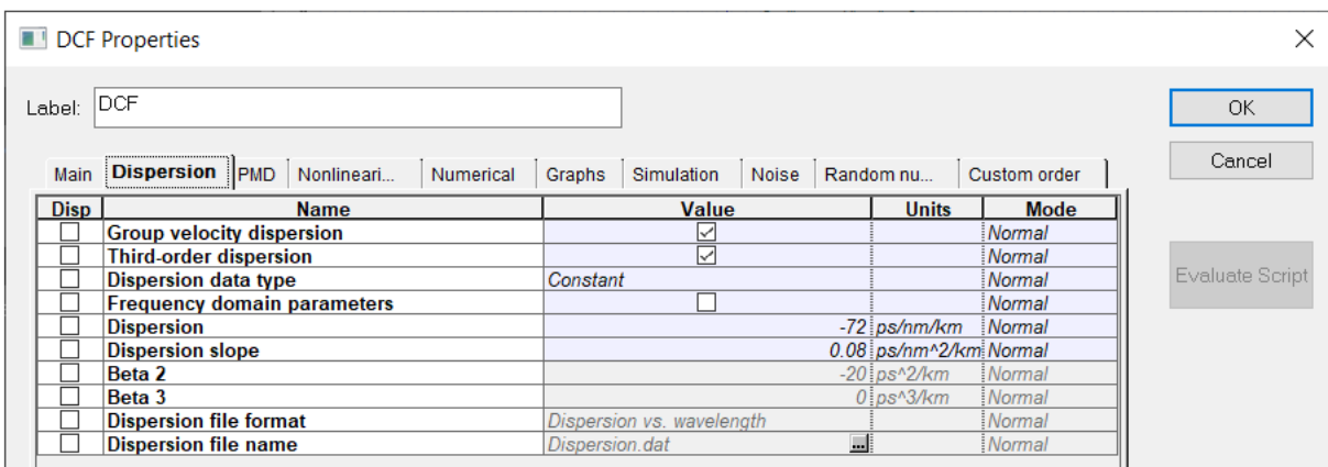
Figura 30. Propiedades de la pestaña Dispersion de la fibra óptica de compensación cromática para el enlace de Rosario - Cataviña.
