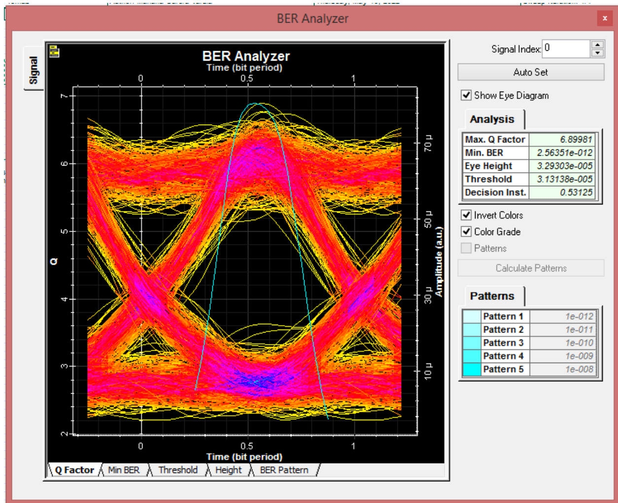
Figura 32. BER obtenido del enlace "Las Cañadas – Santo Tomás".
