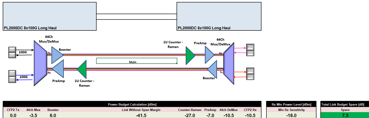
Figura 22. Presupuesto de Potencia para enlaces menores a 190km.
