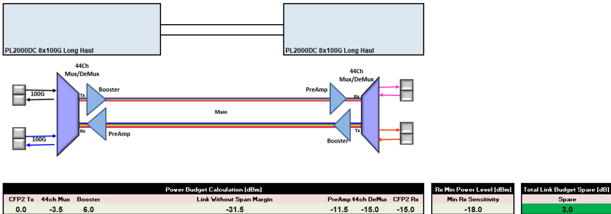
Figura 20. Presupuesto de Potencia para enlaces menores a 90km.
