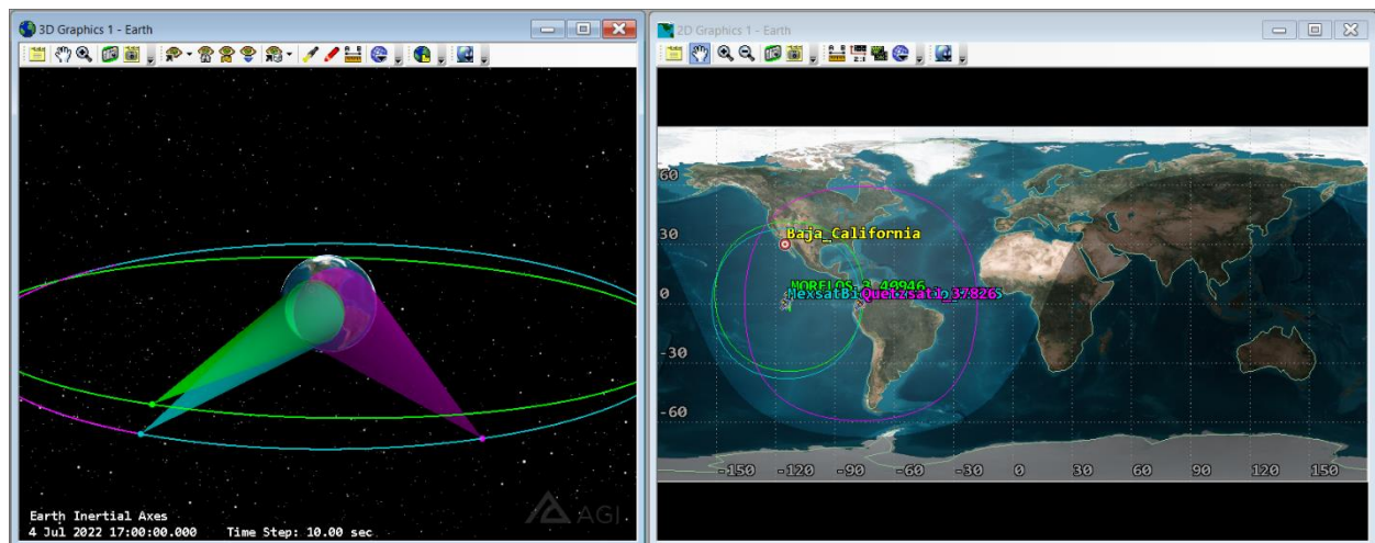
Figura 69. Ángulos de Apertura seleccionados para los satélites colocados para la estación terrena de Campo "La Costilla".
