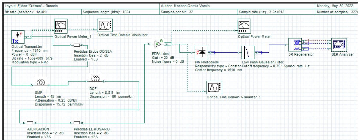
Figura 28. Diagrama de simulación de enlace de fibra óptica del software OptiSystem para el tramo de "Ejidos Nueva Odisea – Rosario".
