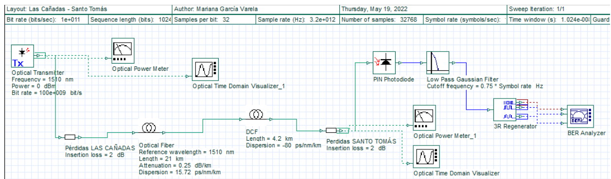
Figura 23. Diagrama de Simulación del Enlace de Fibra Óptica del software OptiSystem para el tramo "Las Cañadas - Santo Tomás"
