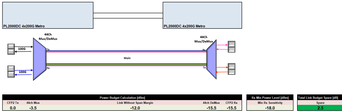
Figura 19. Presupuesto de Potencia para enlaces menores a 34km.
