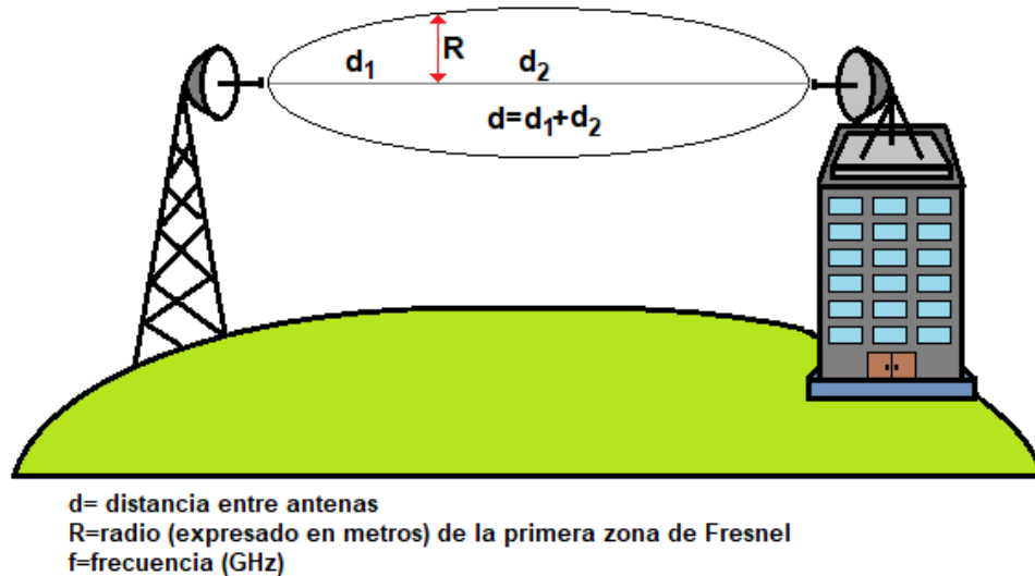
Figura 8. Radio de la primera zona de Fresnel.
