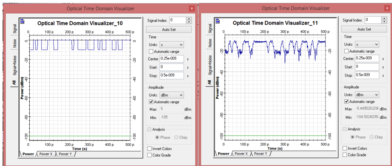
(b) Visualizando la salida del Osciloscopio en Watts
