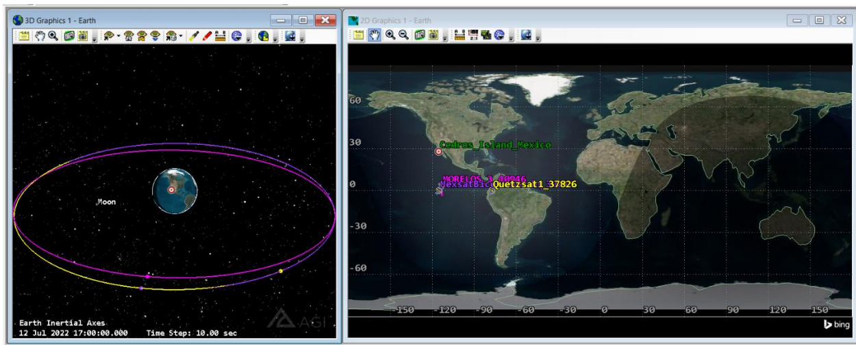
Figura 55. Satélites geostacionarios insertados para la simulación del enlace en Isla de Cedros. Fuente: Elaboración propia utilizando el software STK™. (2023).
