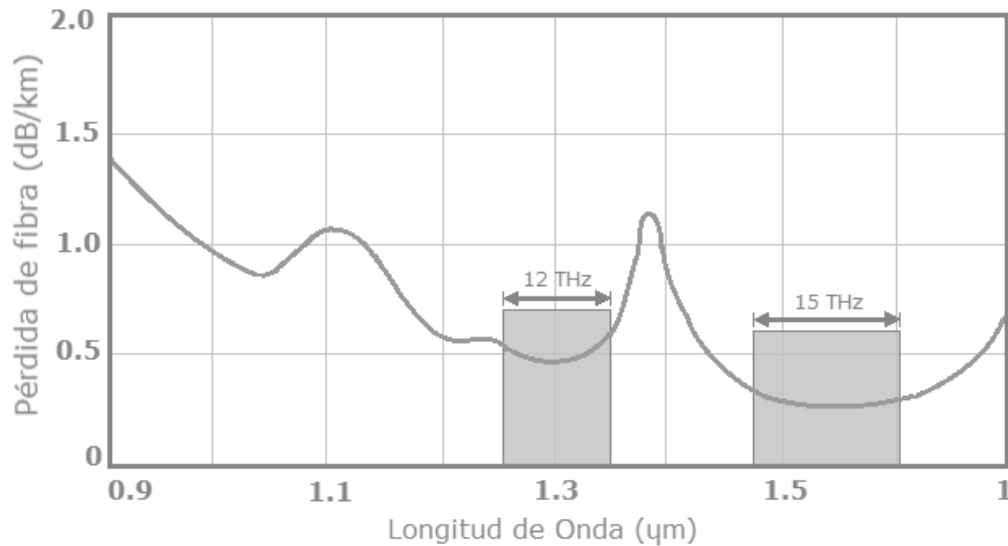
Figura 6. Ventanas de transmisión de bajas pérdidas de las fibras de sílice en las regiones de longitudes de onda cercanas a 1,3 y 1,55 \mu\text{m} .
