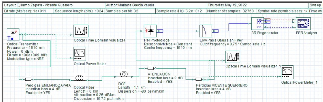
Figura 27. Diagrama de simulación de enlace de fibra óptica del software OptiSystem para el tramo de "Emiliano Zapata – Vicente Guerrero".
