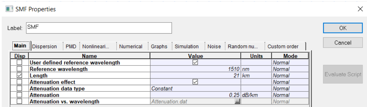
Figura 25. Propiedades de la pestaña Main de la Fibra Monomodo utilizada en la Simulación.
