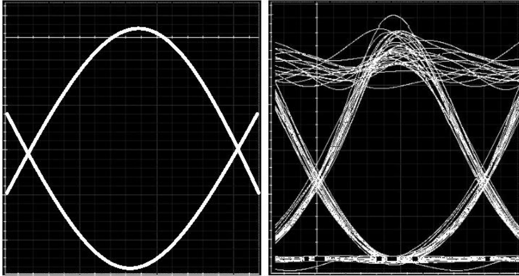
Figura 7. Ejemplo de Diagrama de Ojo ideal vs. Degradado.
