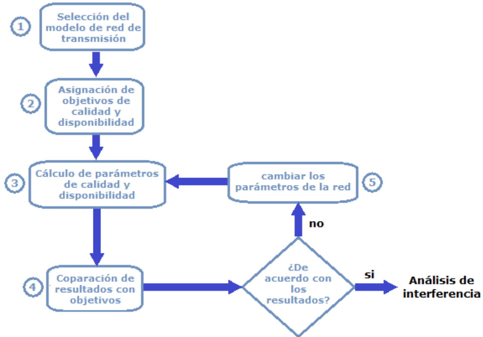
Figura 14. Proceso para establecer objetivos de calidad y disponibilidad.
