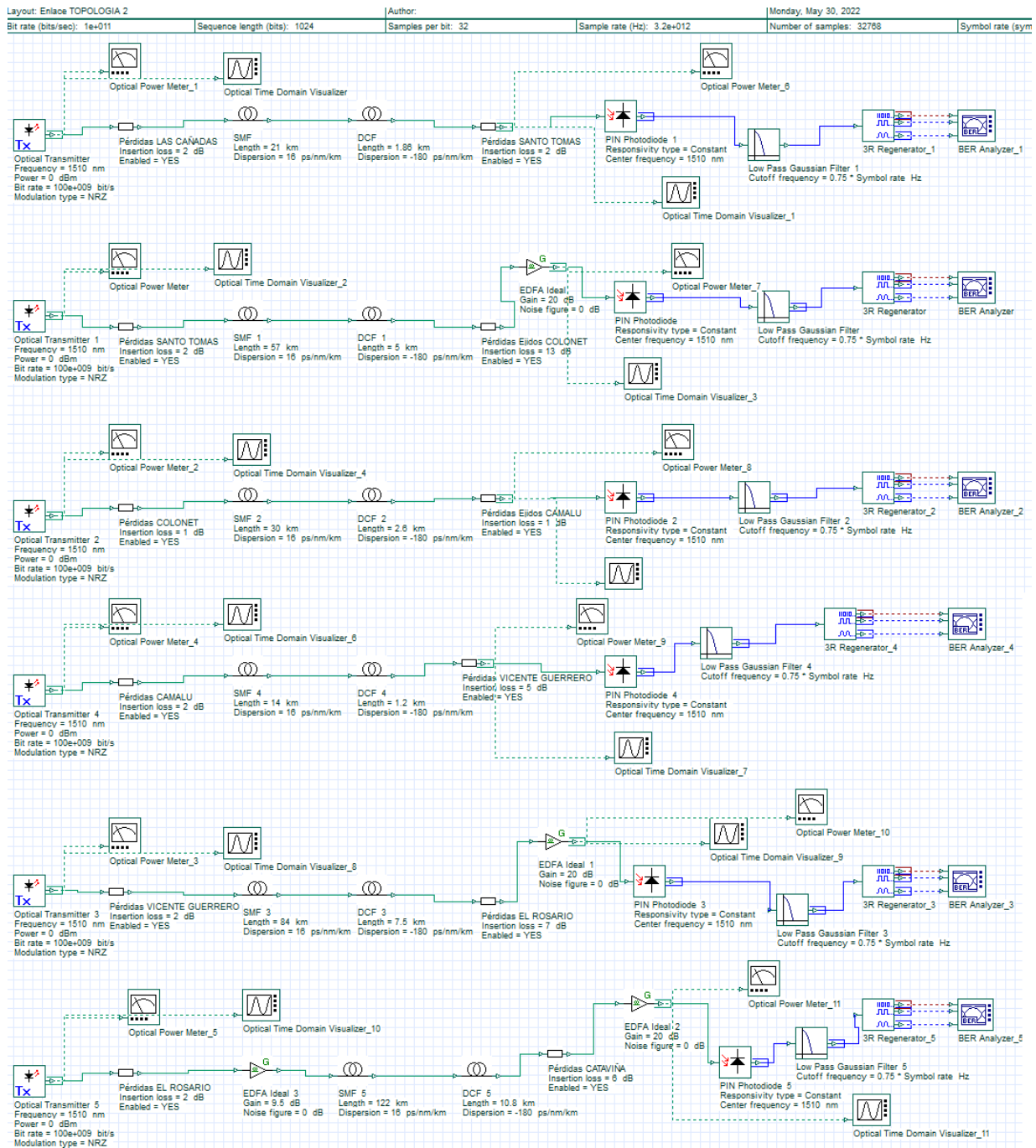
Figura 59. Diagrama de Simulación de Enlace de Fibra Óptica de OptiSystem para el enlace "Las Cañadas - Cataviña".
