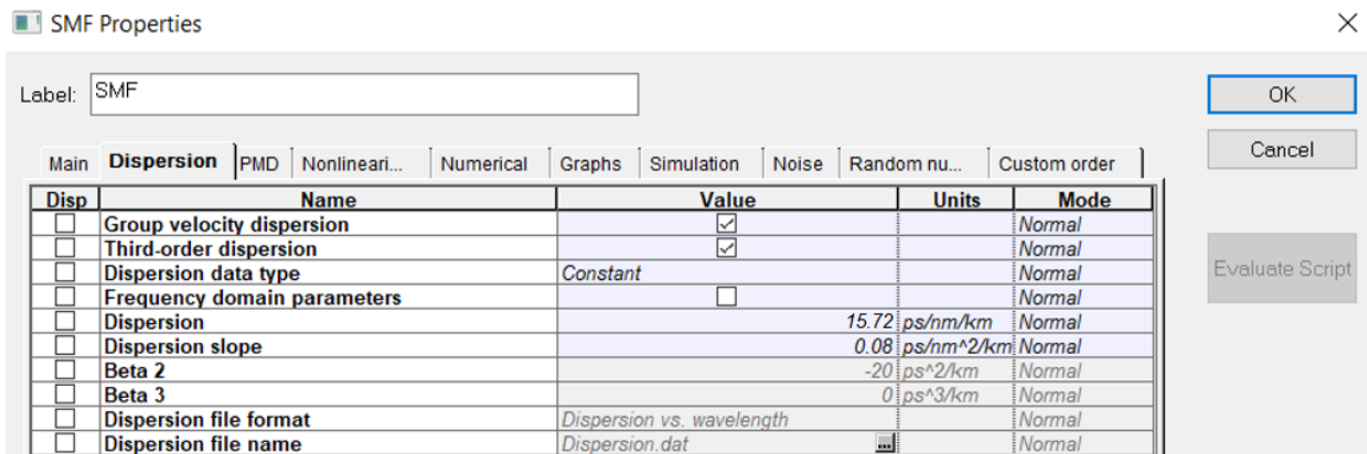
Figura 26. Propiedades de la pestaña "Dispersion" de la fibra monomodo utilizada en la simulación.
