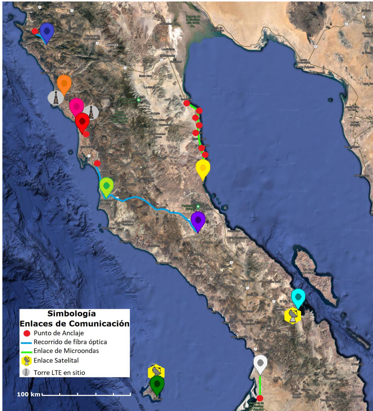
Mapa 16. Propuesta de Topología 1. Fuente: Elaboración propia (2022).
