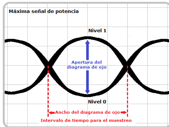
Figura 12. Ejemplo de patrón de Diagrama de ojo de una señal óptica vista en un osciloscopio.
