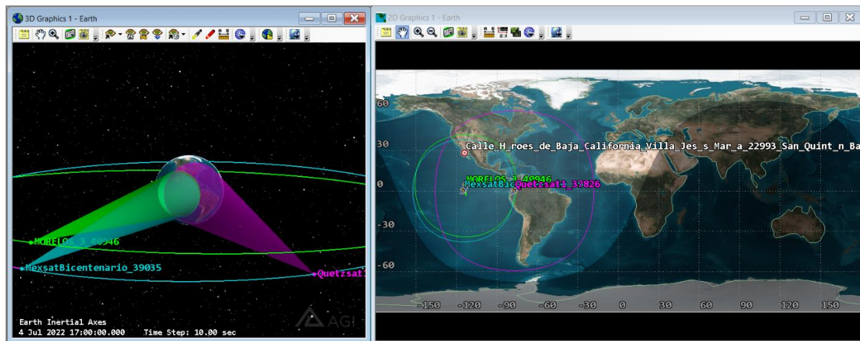
Figura 70. Proyección geográfica de los ángulos de apertura en relación con la estación terrena de Villa de Jesús María.
