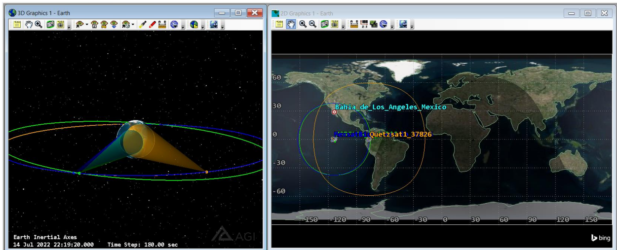
Figura 54. Ángulos de apertura y áreas de radiación de las antenas satelitales. Fuente: Elaboración propia utilizando el software STK™. (2023).
