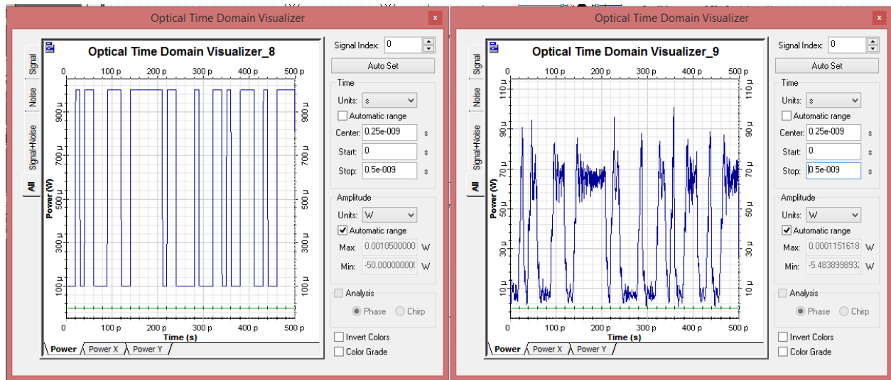
(a) Visualizando la salida del Osciloscopio en Watts.
