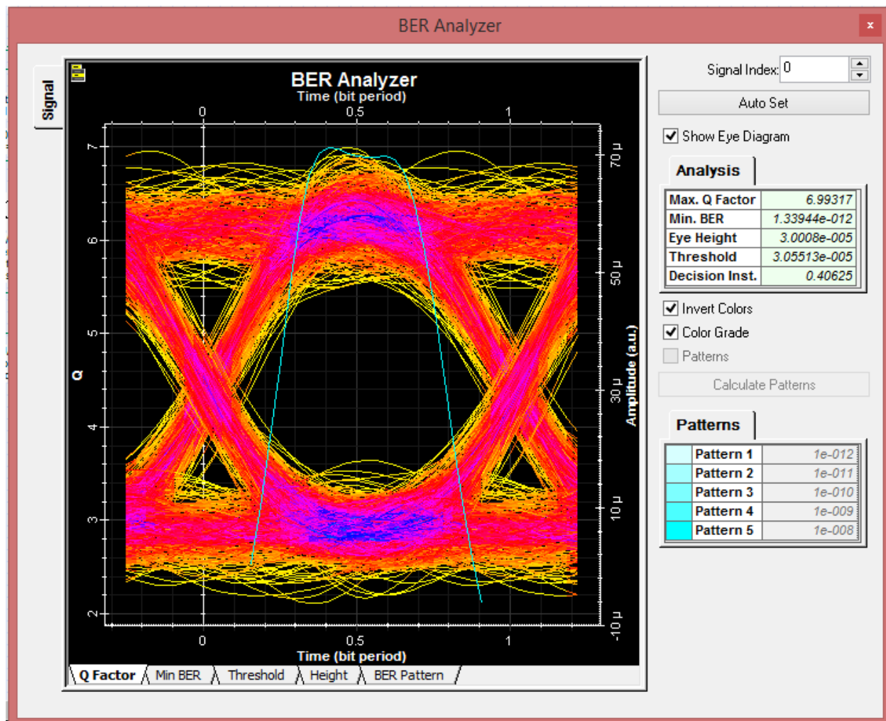
Figura 36. Primer BER del enlace "Ejidos Nueva Odisea-Rosario".
