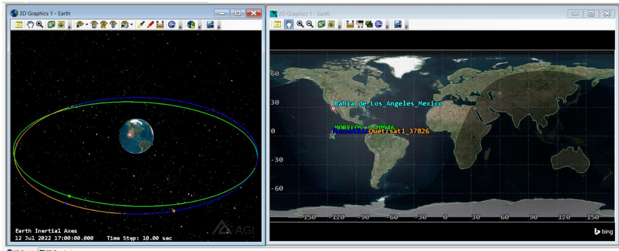
Figura 53. Satélites geostacionarios insertados para la simulación del enlace en Bahía de los Ángeles.
