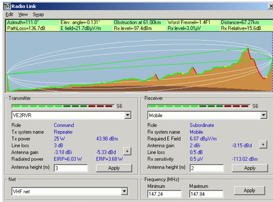
Figura 15. Radioenlace con elevación de terreno en Radio Mobile™.
