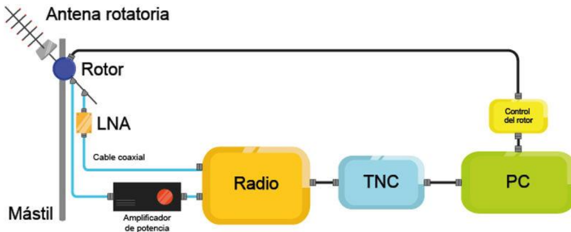
Figura 9. Esquema típico de la estructura de estación de monitoreo terrestre.
