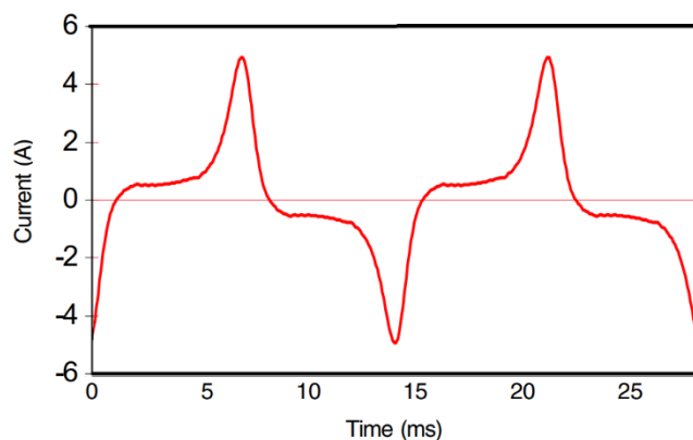
Figura 6. Corriente de magnetización de un transformador. THD=76.1%
