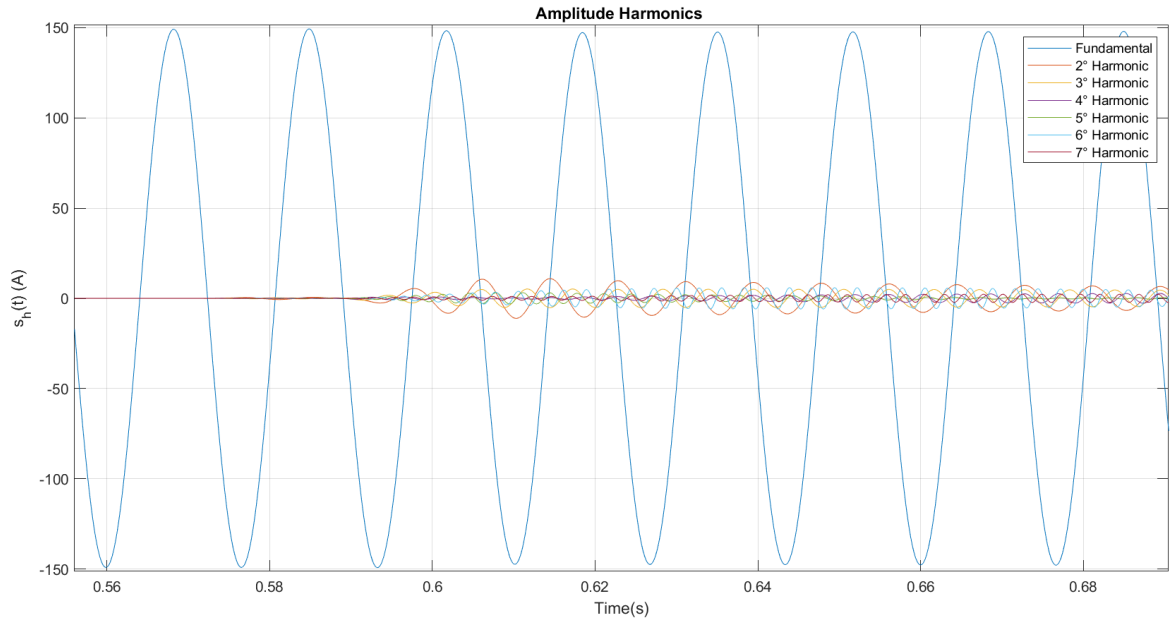
Figura 24. Los componentes armónicos que componen a la corriente aparecidos durante la energización de un transformador.
