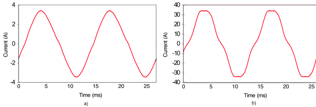
Figura 7. a) Corriente de un refrigerador 120 V. THD=6.3% b) Corriente de un aire acondicionado domestico 240 V. THD=10.5%
