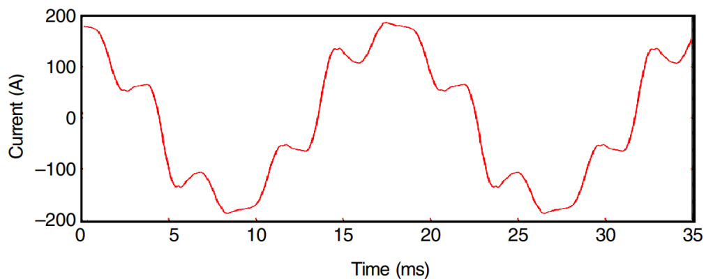
Figura 14. Corriente medido en estación del metro.
