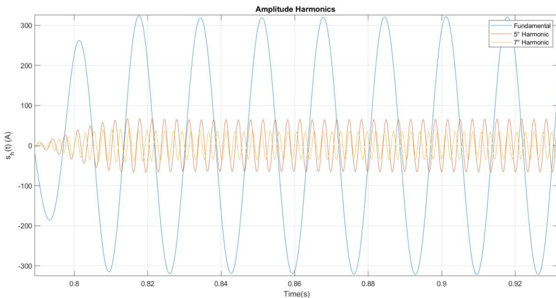
Figura 26. Los componentes armónicos que componen a la corriente aparecidos durante al conectar la estación del metro al sistema.
