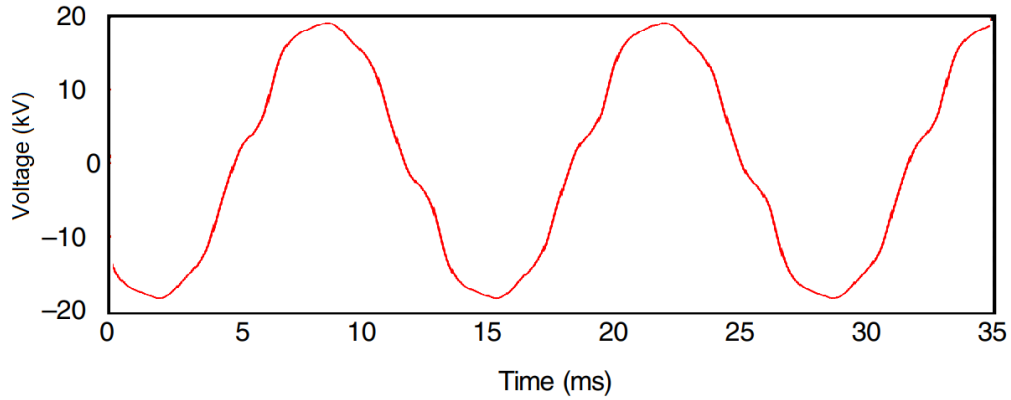
Figura 15. Voltaje medido en estación del metro.
