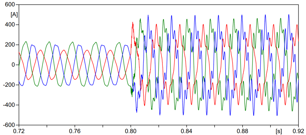
Figura 25. Corrientes resultantes en t=0.20 s en ATPDraw al conectar la estación del metro.
