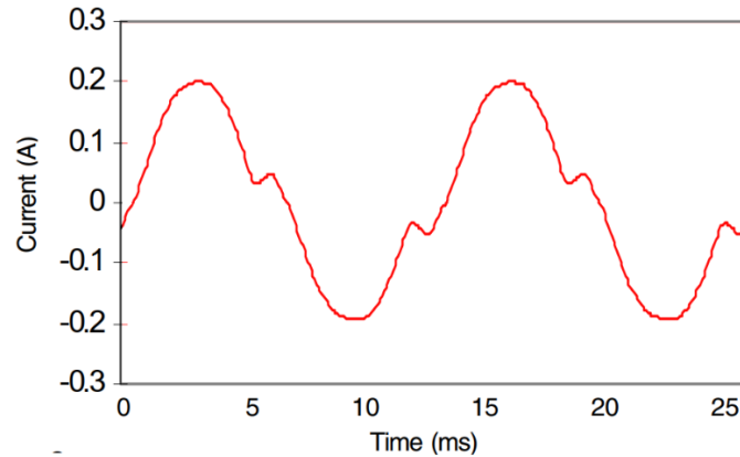
Figura 8. Corriente de lampara fluorescente con balastro magnético. THD=18.5%.
