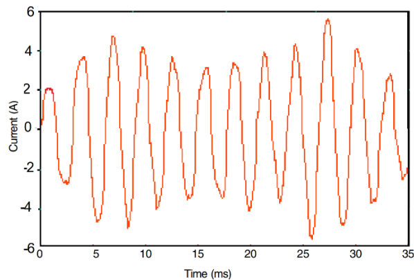
Figura 9. Corriente de horno eléctrico.
