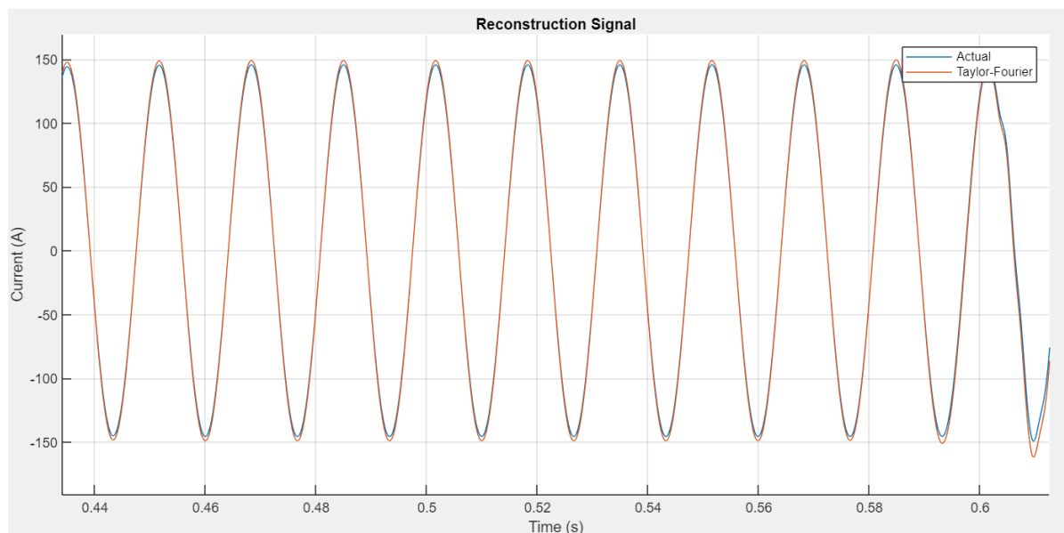
Figura 30. Reconstrucción de la corriente con la Transformada digital de Taylor-Fourier.
