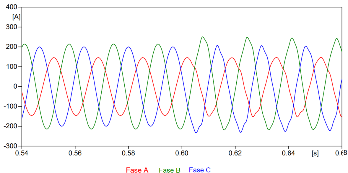
Figura 23. Corrientes resultantes en t=0.60 s en ATPDraw al energizar un transformador.
