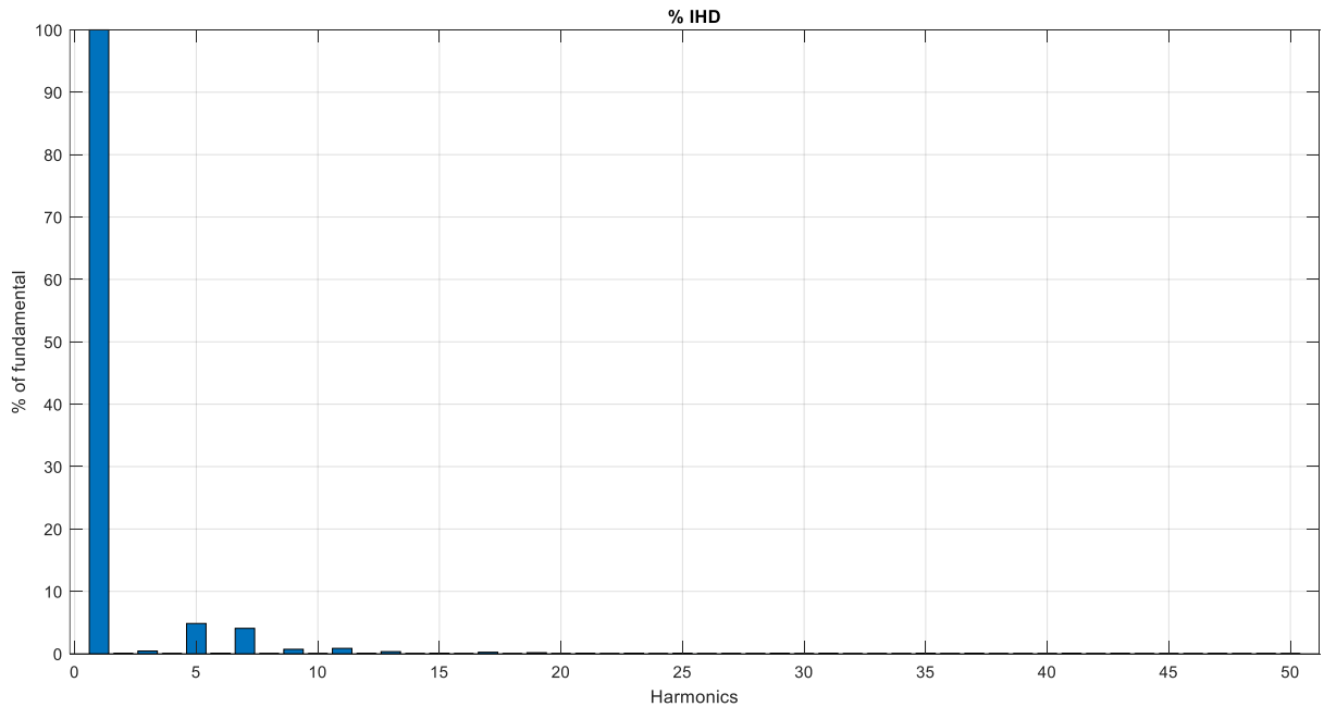
Figura 16. IHD del voltaje medido en la estación del metro.
