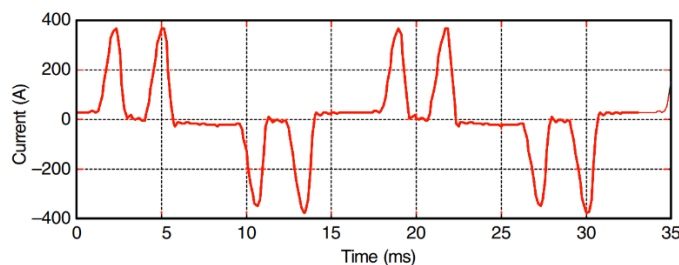
Figura 13. Corriente de PWM-type ASD.
