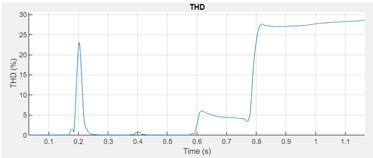
Figura 34. THD del sistema durante todo el tiempo.
