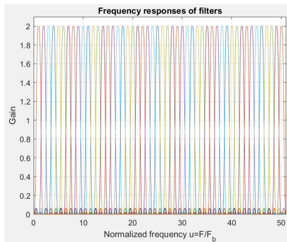
Figura 36 Banco de filtros digitales de Taylor-Fourier con su frecuencia normalizada.
