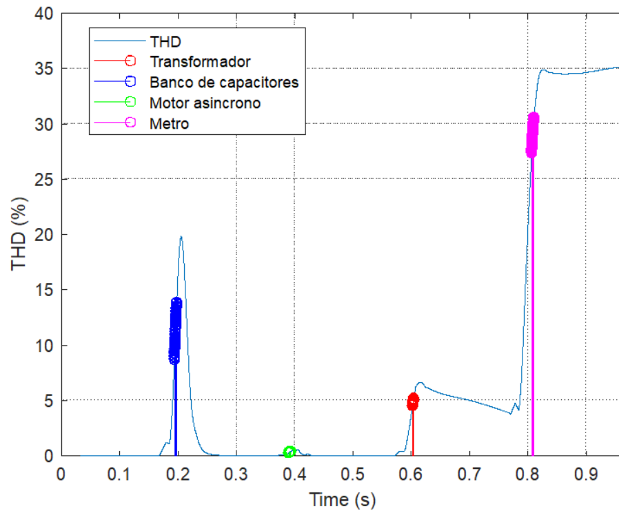
Figura 28. Localizador de cargas no lineales modeladas en el sistema de distribución 23 kV en las tres fases.
