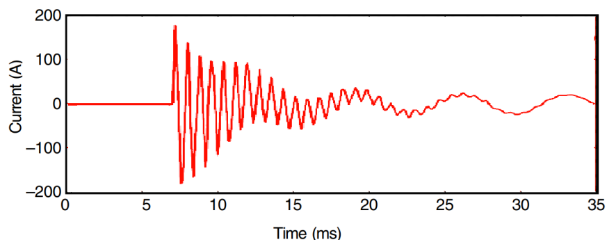
Figura 11. Corriente de la energización de un banco de capacitores.
