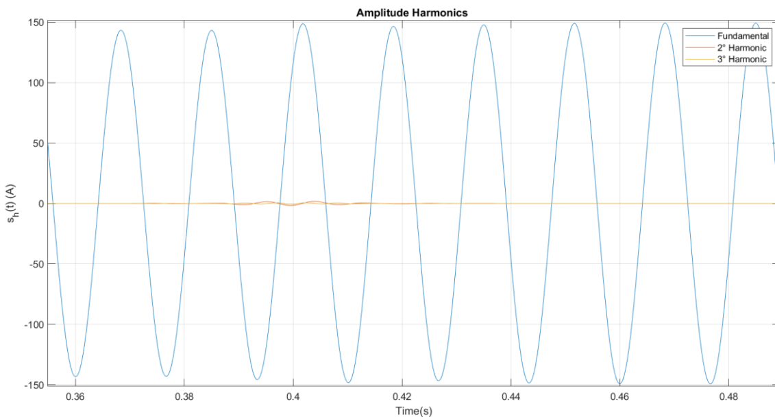
Figura 22. Los componentes armónicos que componen a la corriente aparecidos durante la energización de un banco de capacitores.
