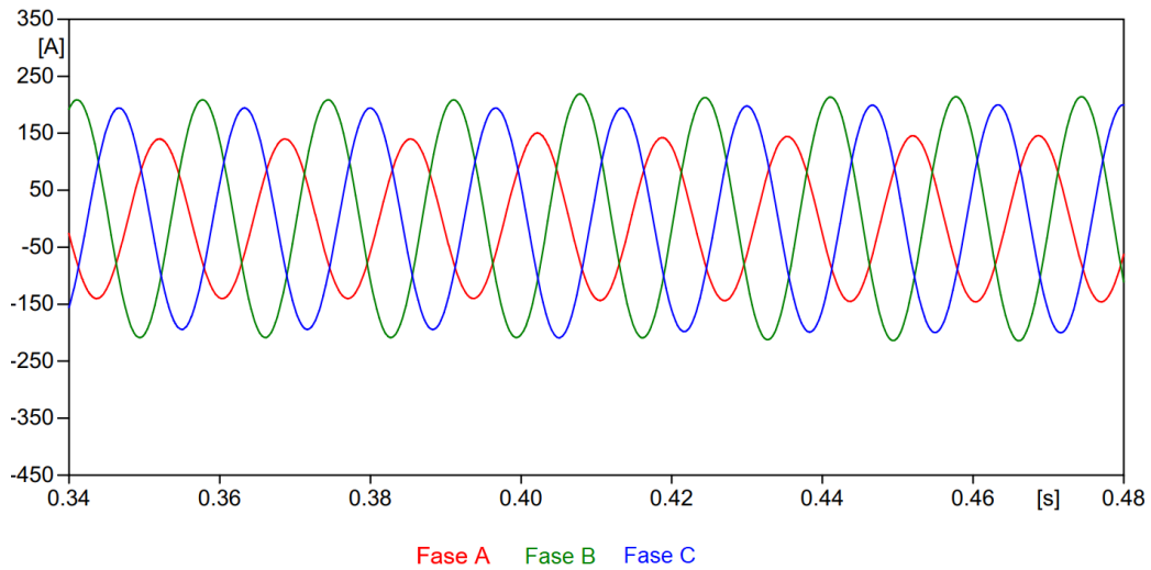
Figura 21. Corrientes resultantes en t=0.40 s en ATPDraw al arranque de un motor de inducción.
