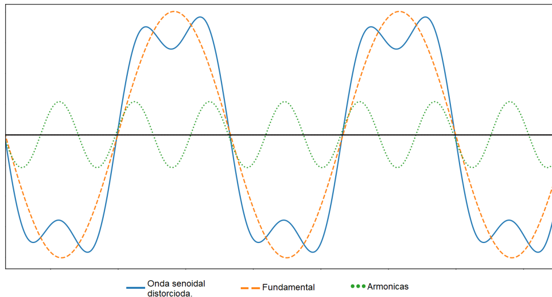
Figura 1 Onda senoidal distorsionada con su descomposición de la señal en sus componentes.
