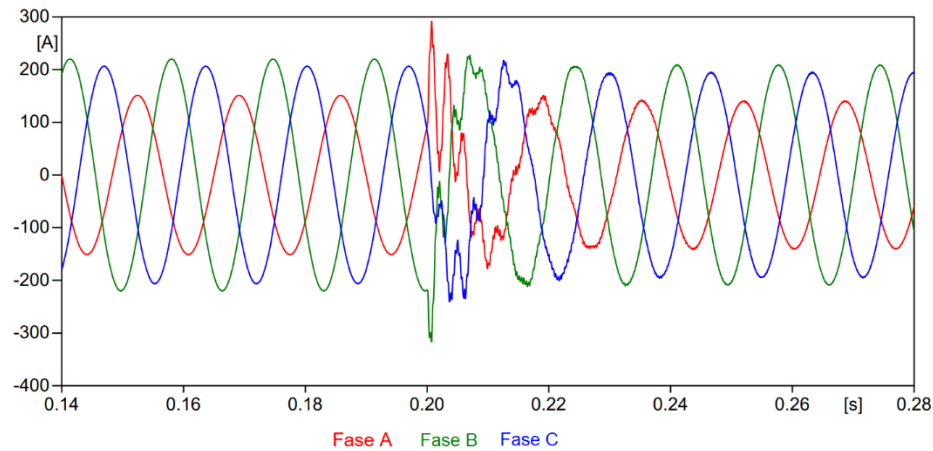
Figura 19. Corrientes resultantes en t=0.20 s en ATPDraw al energizar un banco de capacitores.
