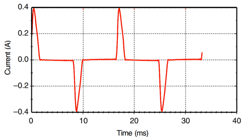
Figura 10. Corriente de variador de velocidad ajustable.
