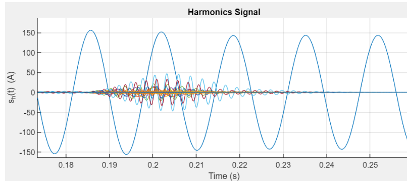
Figura 31. Descomposición de corriente en sus principales en sus componentes
