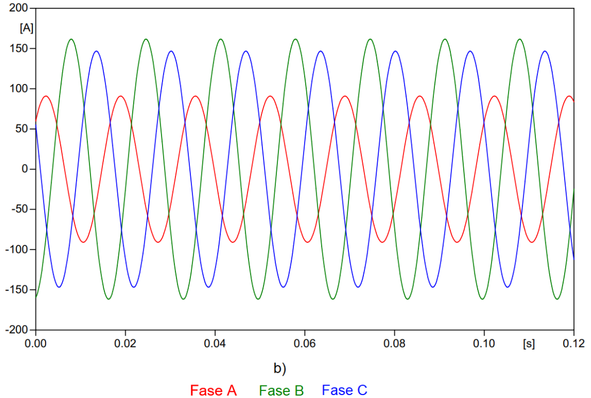
Figura 18. a) Voltaje del sistema resultante, sin conexión de cargas no lineales. b) Corriente del sistema resultante, sin conexión de cargas no lineales.
