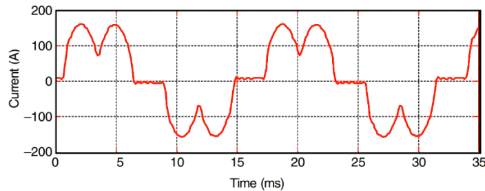
Figura 12. Corriente de una fuente de corriente de tipo de variador da velocidad ajustable.
