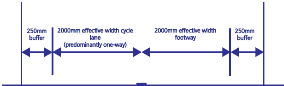
Figura 2.9 Ancho mínimo para los caminos delimitados de Queen's Walk Fuente: Atkins, 2016
