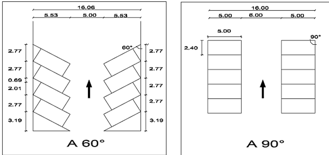
Figura 5.2 Cajones de estacionamiento orientados a 60° y 90° para autos grandes. Fuente: Norma Técnica Complementaria para el Proyecto Arquitectónico
