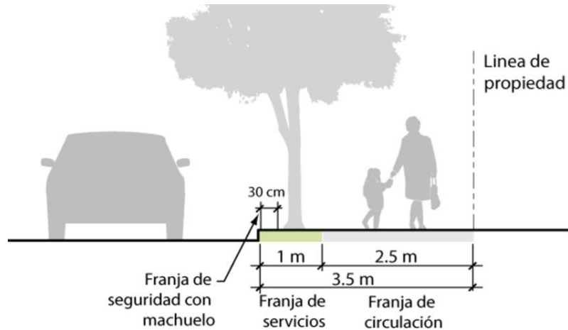
Figura 1.4 Ejemplo de configuración de una banqueta de 3.5 m de ancho Fuente: Manual de lineamientos y estándares para vías peatonales y ciclistas
