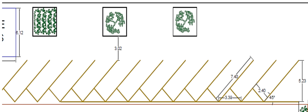
Figura 5.5 Dimensiones de la propuesta de cajones orientados a 45^\circ
