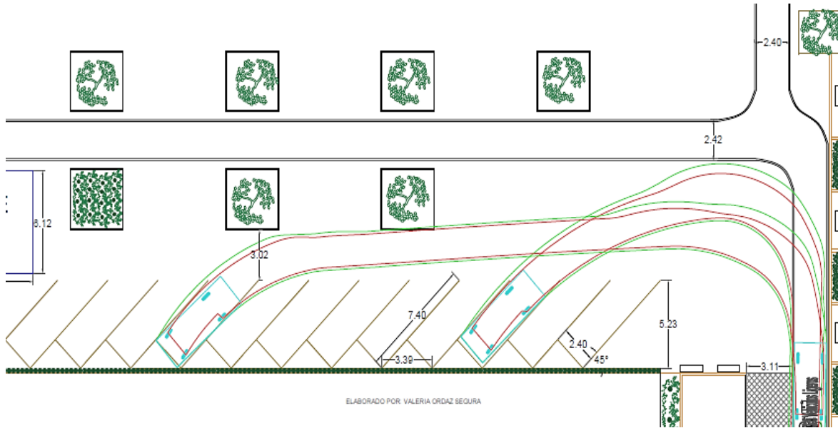
Figura 5.11 Zona de influencia del vehículo para el estacionamiento a 45° Fuente: Elaboración propia
