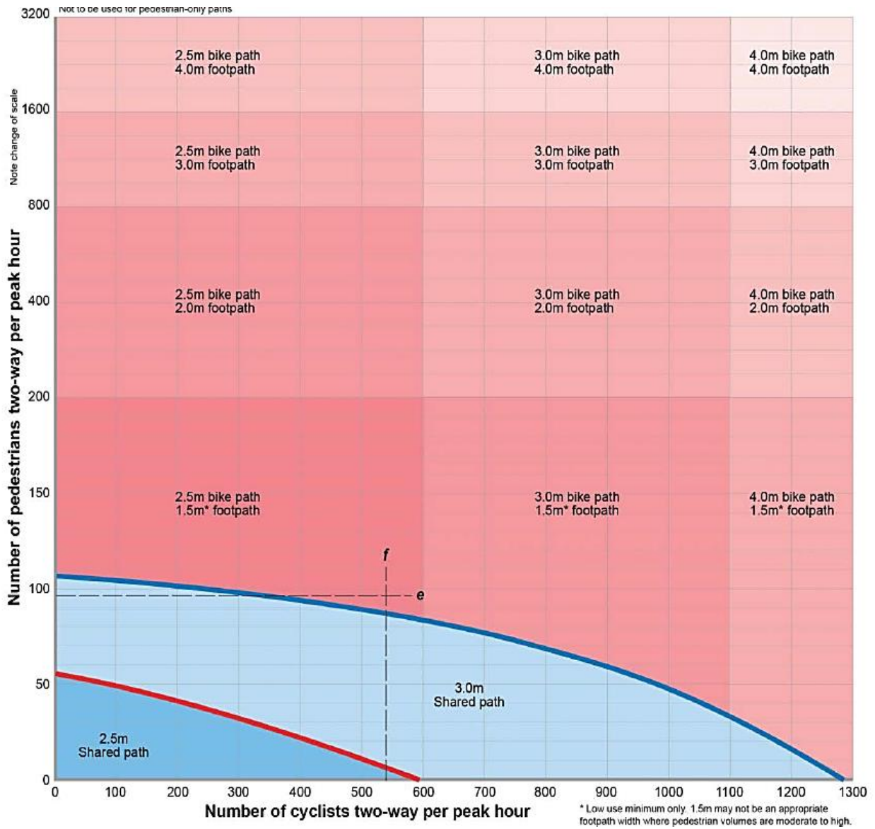
Figura 2.12 Grafico empleado en Queensland, Australia para el diseño de caminos compartidos Fuente: Queensland DTMR, 2014
