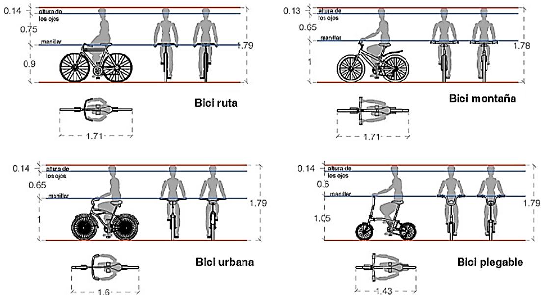
Figura 1.5 Dimensiones de distintos tipos de bicicletas en metros Fuente: Manual de lineamientos y estándares para vías peatonales y ciclista
