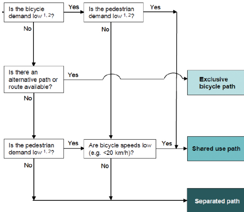
Figura 2.7 Guía simplificada para elegir un tipo de camino compartido Fuente:Austroads, 2009
