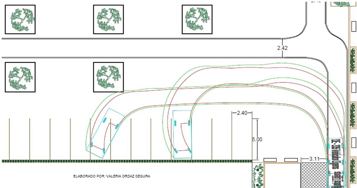
Figura 5.9 Zona de influencia del vehículo para el estacionamiento a 90° Fuente: Elaboración propia
