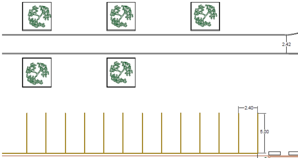
Figura 5.3 Dimensiones de la propuesta de cajones orientados a 90^\circ Fuente: Elaboración propia
