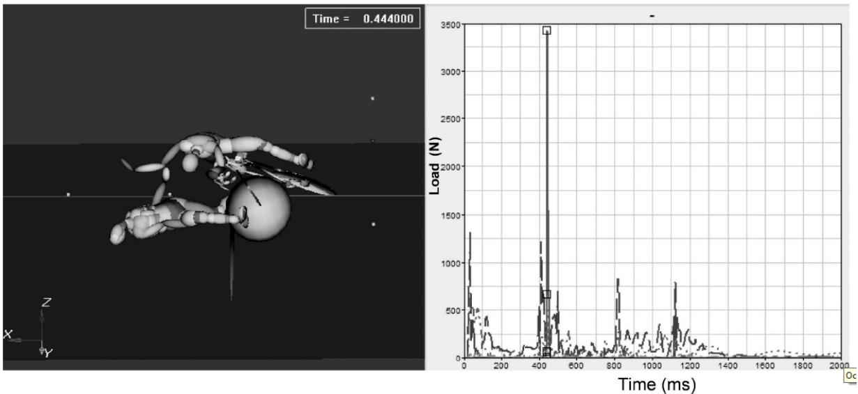
Figura 2.2 Carga de compresión axial en el cuello a través del tiempo durante un impacto
