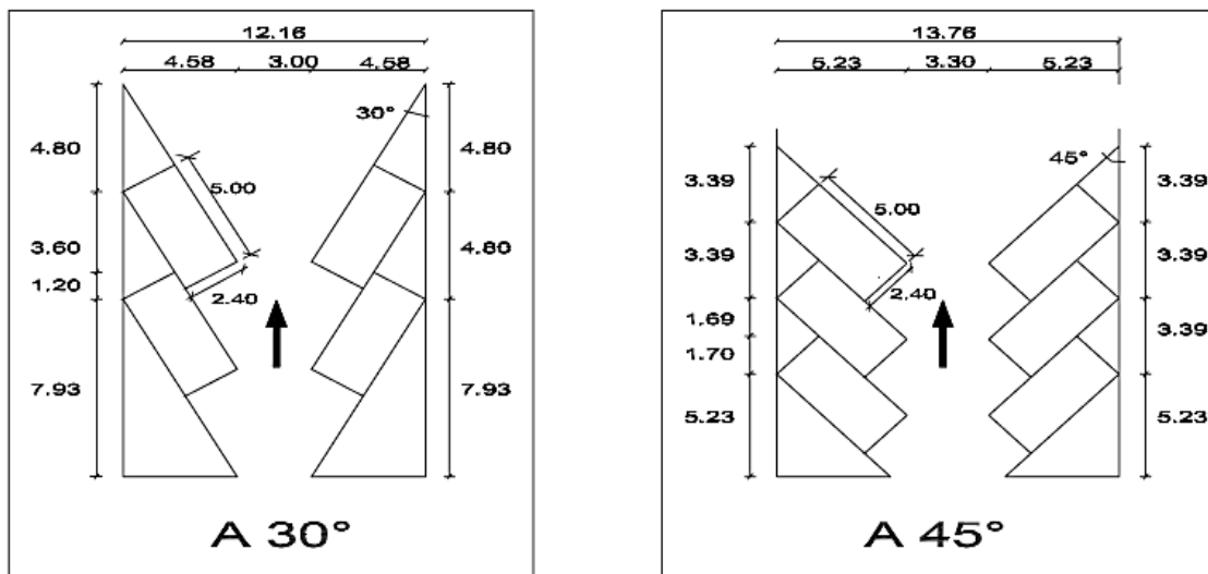
Figura 5.1 Cajones de estacionamiento orientados a 30° y 45° para autos grandes.
