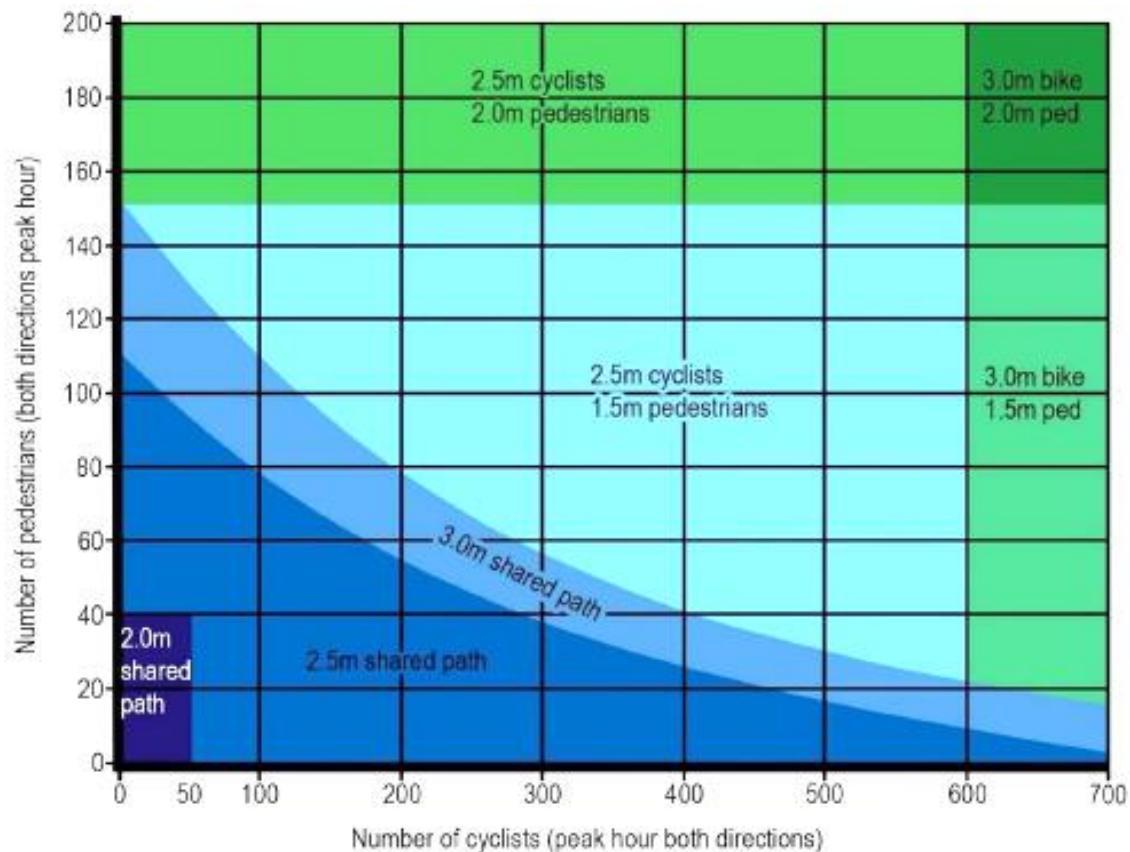
Figura 2.10 Ancho mínimo en función de la cantidad de usuarios.
