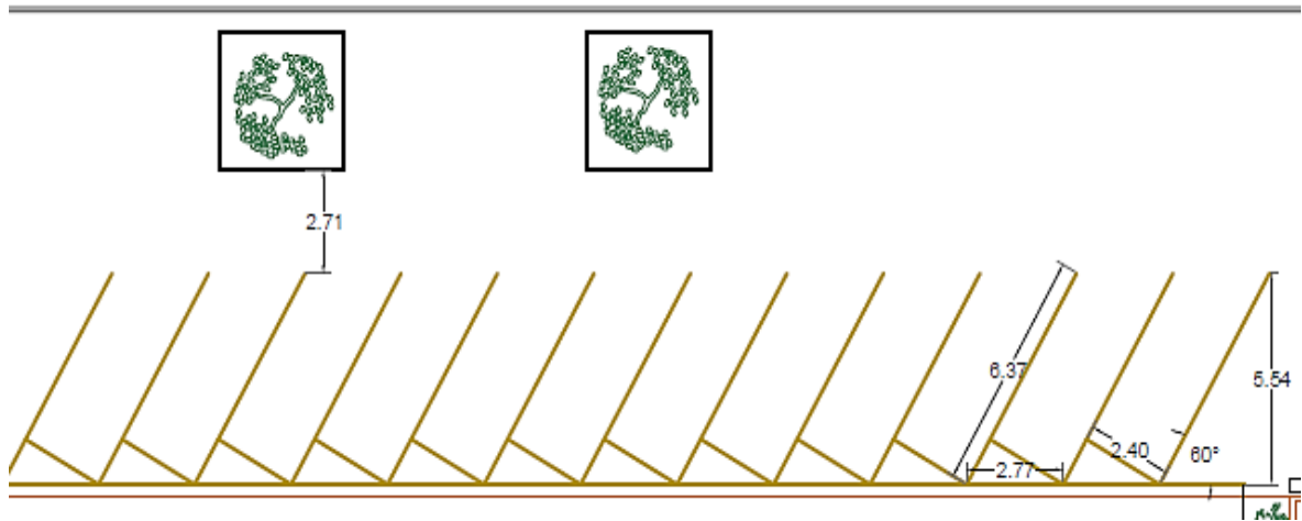
Figura 5.4 Dimensiones de la propuesta de cajones orientados a 60^\circ
