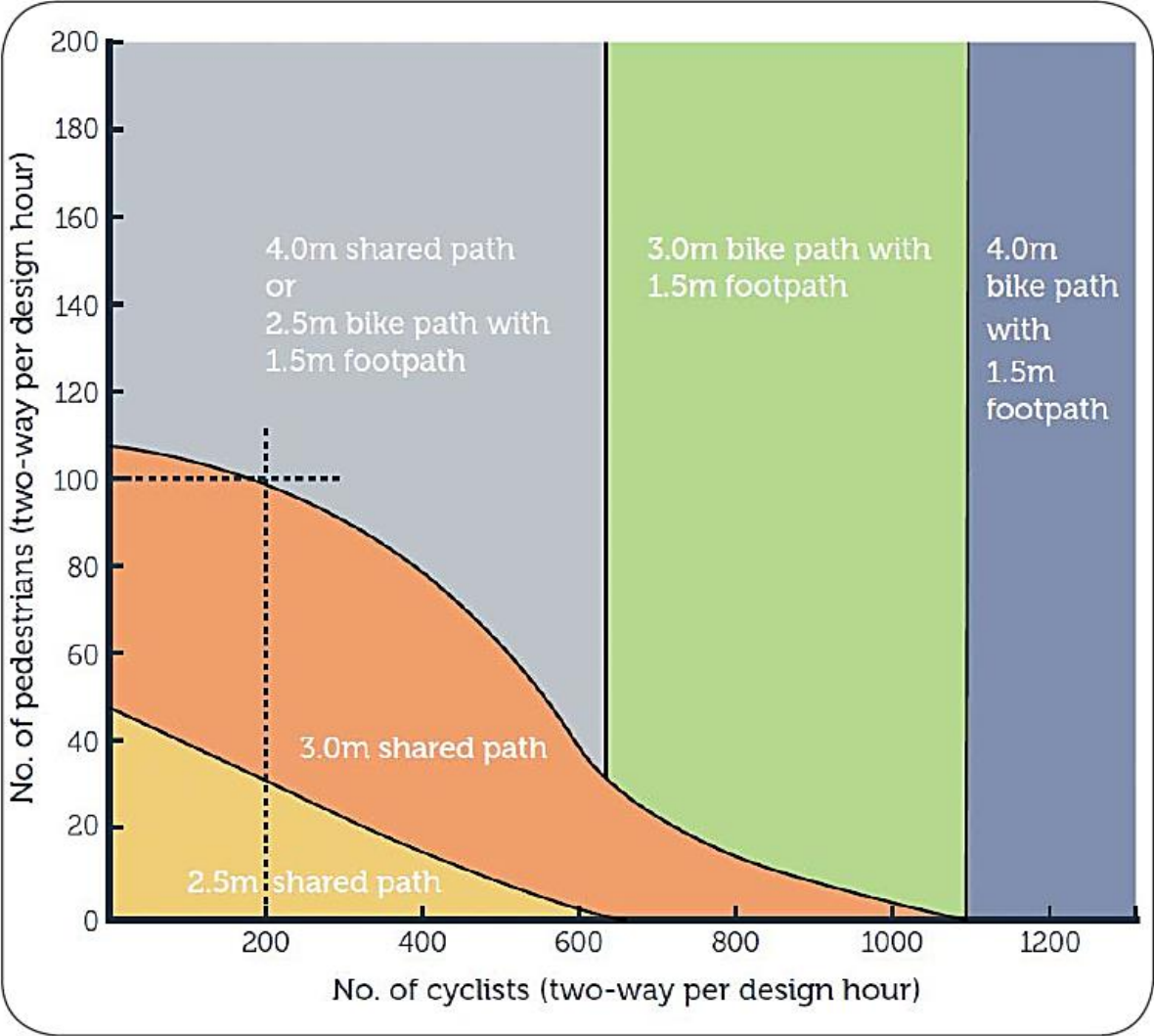
Figura 2.11 Grafico empleado en Victoria, Australia para el diseño de caminos compartidos Fuente: VicRoads, 2013
