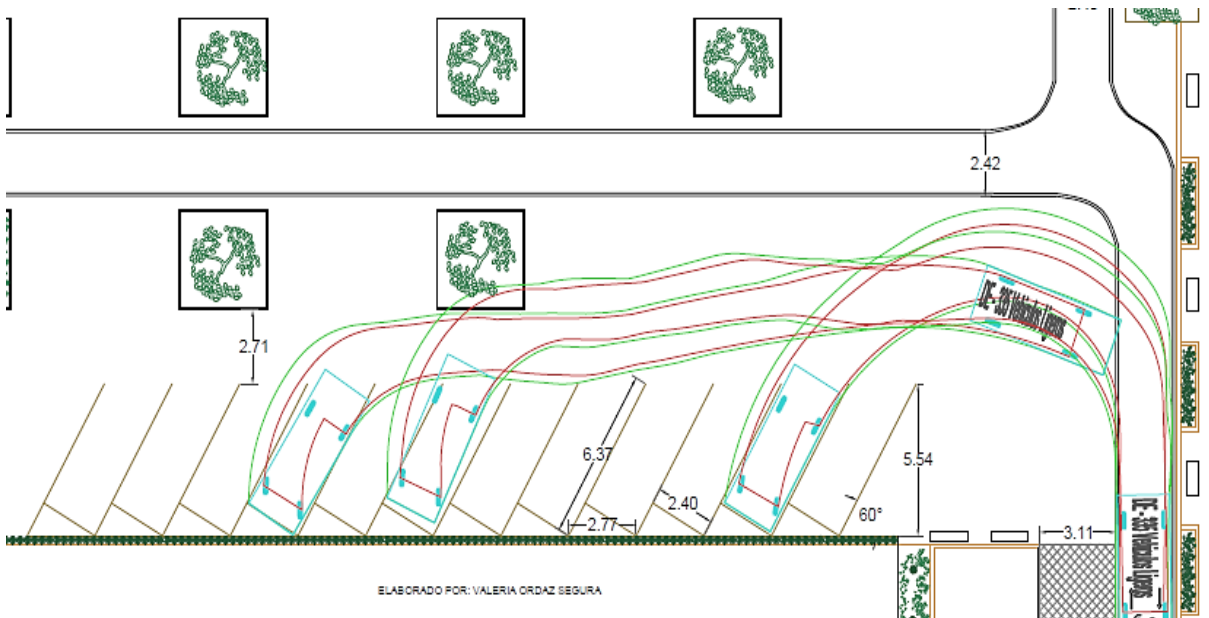
Figura 5.10 Zona de influencia del vehículo para el estacionamiento a 60° Fuente: Elaboración propia
