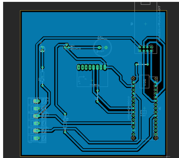
Figura 3.13 Diagrama PCB de los módulos esclavos.
