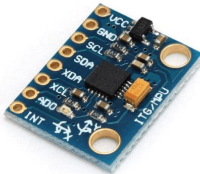
Figura 2.19 Módulo MPU-6050.
