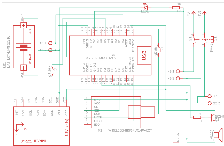
Figura 3.12 Diagrama esquemático de los módulos esclavos.
