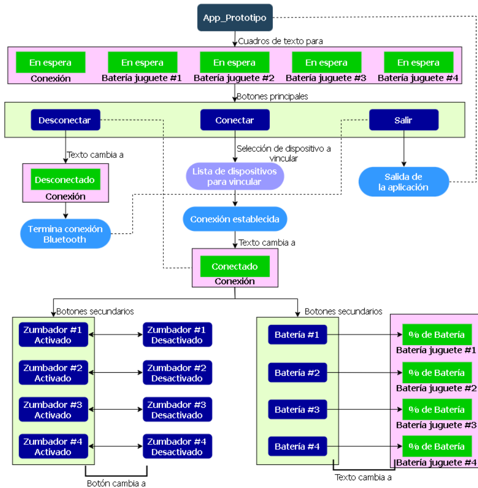
Figura 3.17 Mapa de navegación para la aplicación desarrollada para el prototipo.
