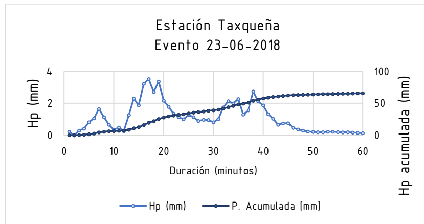
Gráfica 9 Hietograma de un evento convectivo 23-06-2018 en la estación Taxqueña.
