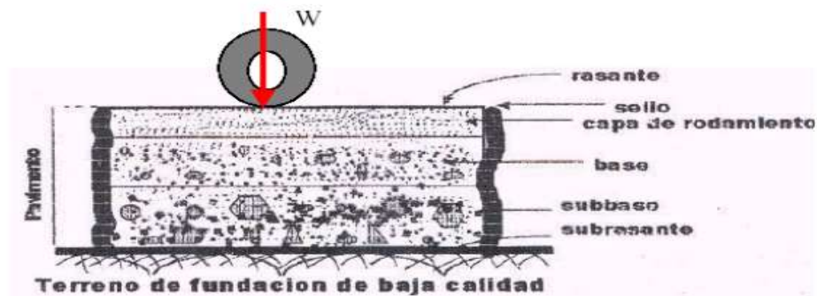
Figura 1: Estructura del pavimento
