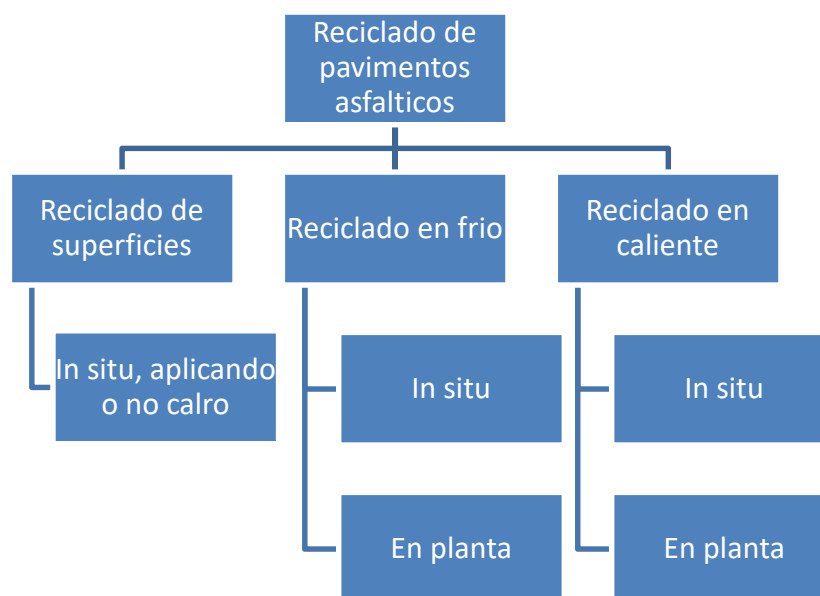
Figura 3: clasificación de técnicas de reciclado de pavimentos
