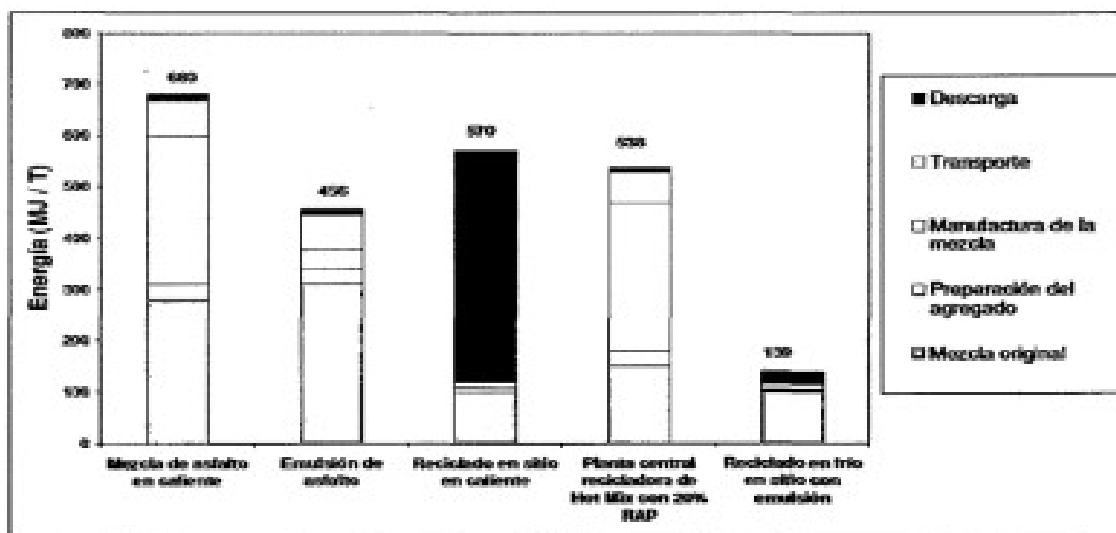
Figura 4: costo y energía de producción de mezcla asfáltica
