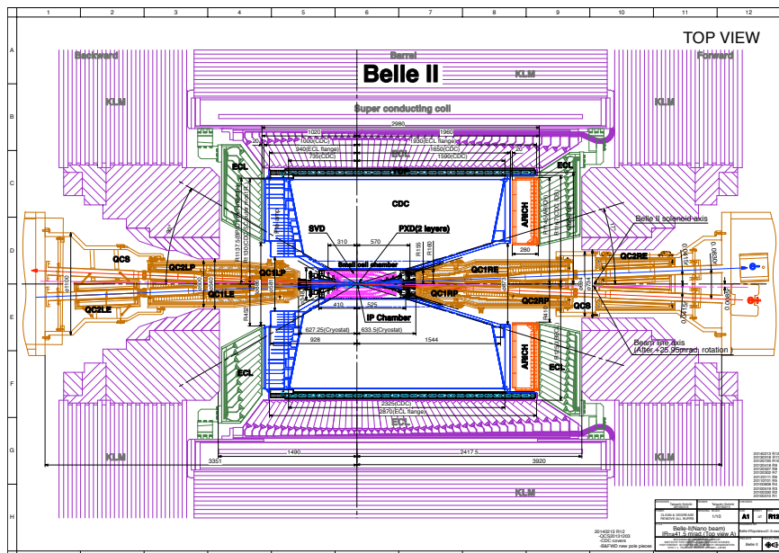
Figura 3.2: Componentes del detector del experimento Belle II.
