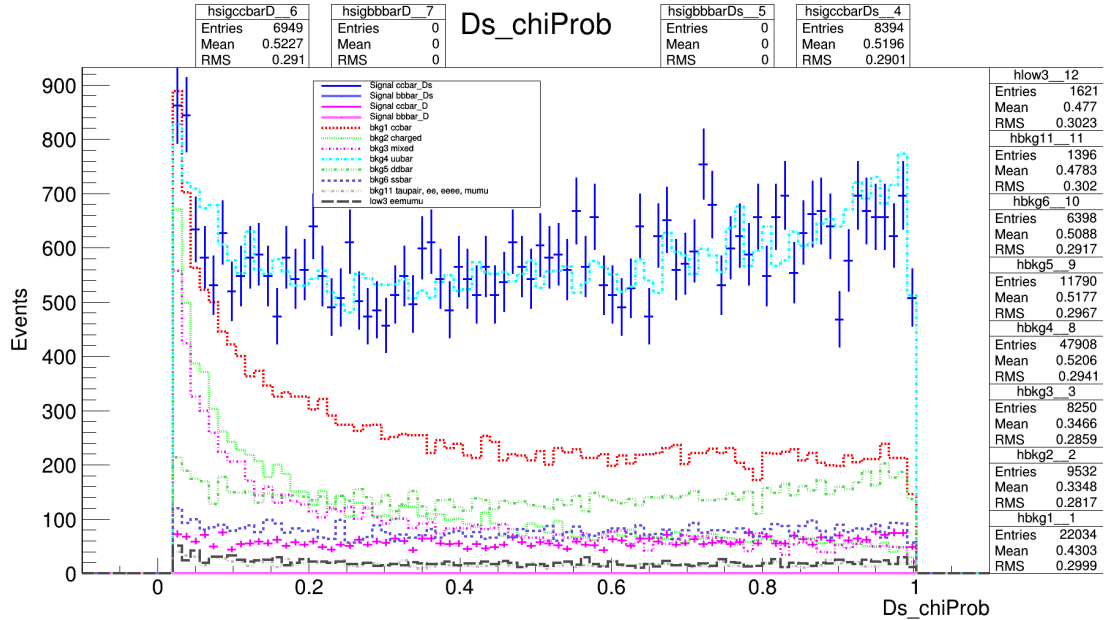
Figura 4.16: Distribución de la variable Ds\_chiProb después de optimización. Las cruces azules corresponden a nuestra señal (candidatos a D_s^+ ) provenientes de la producción c\bar{c} . Las cruces color magenta corresponden a la señal D^+ provenientes de la producción c\bar{c} . El resto de las líneas corresponden al fondo.
