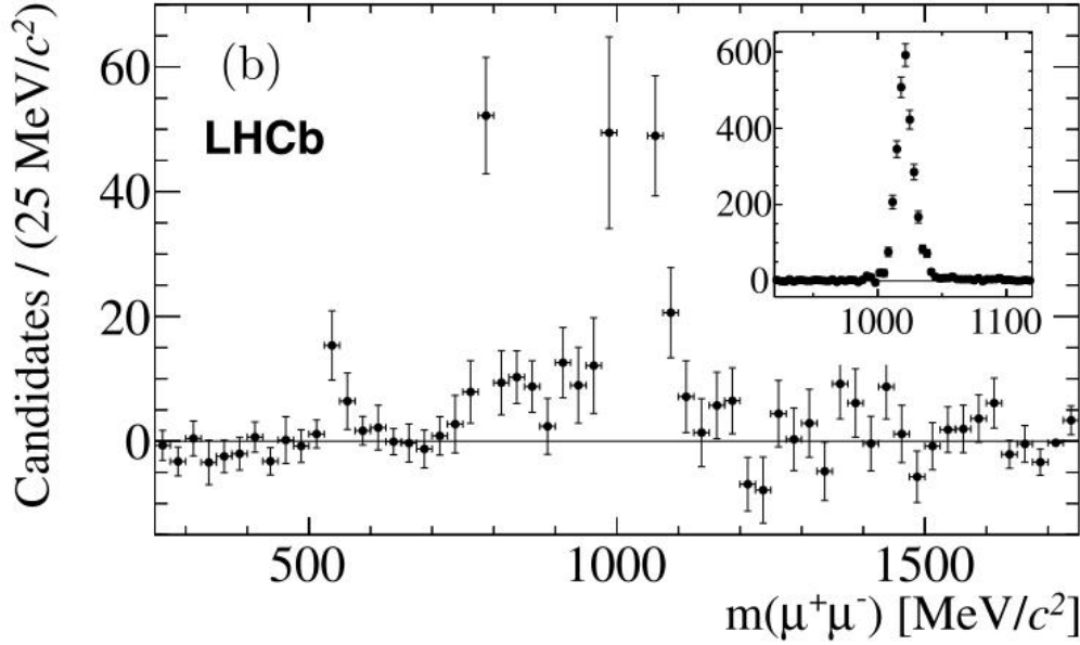
Figura 2.2: Espectro de la masa dileptonica m(\mu^+\mu^-) del decaimiento D_s \rightarrow \pi\mu^-\mu^+ observado por LHCb [14]
