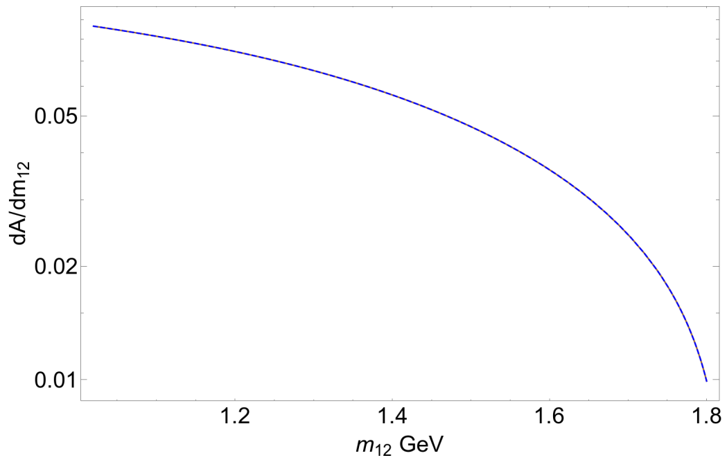
Figura 2.10: Distribución de A_{FB}|_{\cos\theta} en \cos\theta = 0.1 para el decaimiento D_s \rightarrow 3\pi . Ninguna diferencia se logra apreciar comparado con la estimación puramente del espacio fase.
