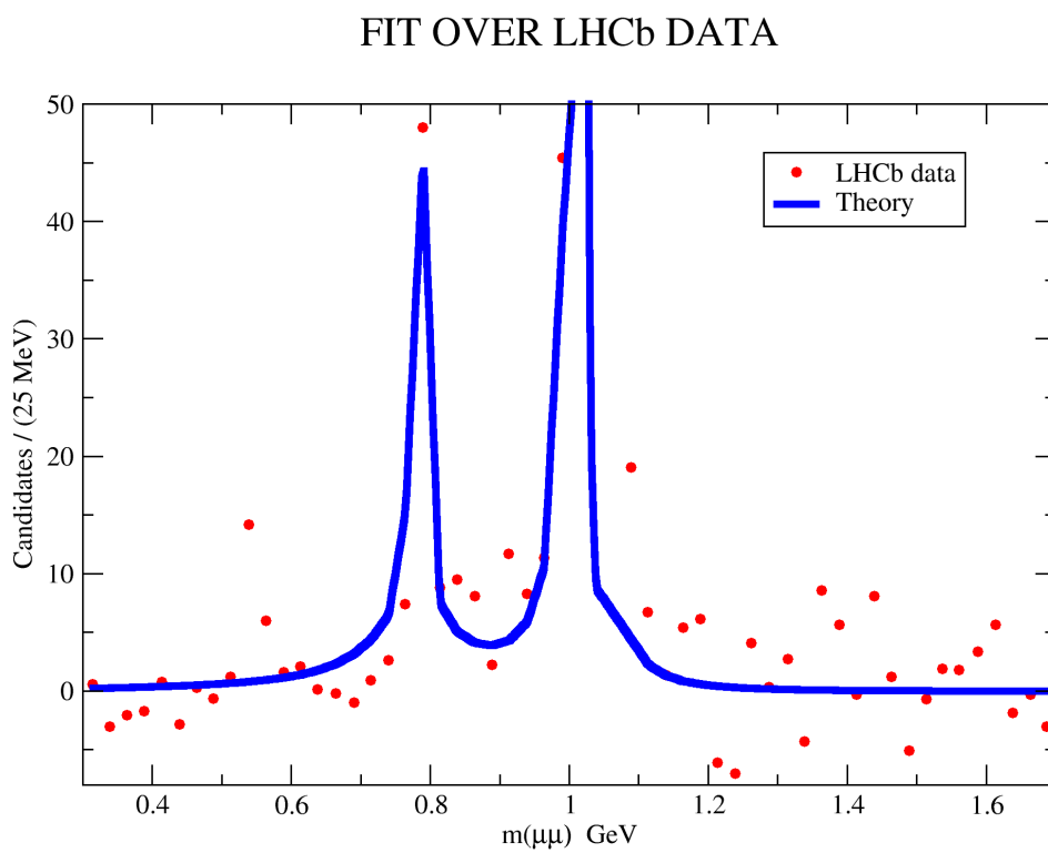
Figura 2.3: Ajuste a los datos de LHCb.
