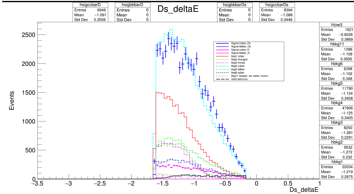
Figura 4.17: Distribución de la variable D_s\_deltaE después de optimización. Las cruces azules corresponden a nuestra señal (candidatos a D_s^+ ) provenientes de la producción c\bar{c} . Las cruces color magenta corresponden a la señal D^+ provenientes de la producción c\bar{c} . El resto de las líneas corresponden al fondo.
