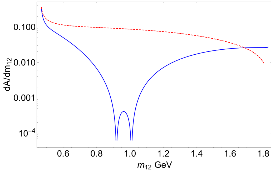
Figura 2.13: Distribución de A_{FB}|\cos\theta en SD para \cos\theta = 0.1 (línea sólida), comparada con la estimación puramente espacio fase (línea punteada).
