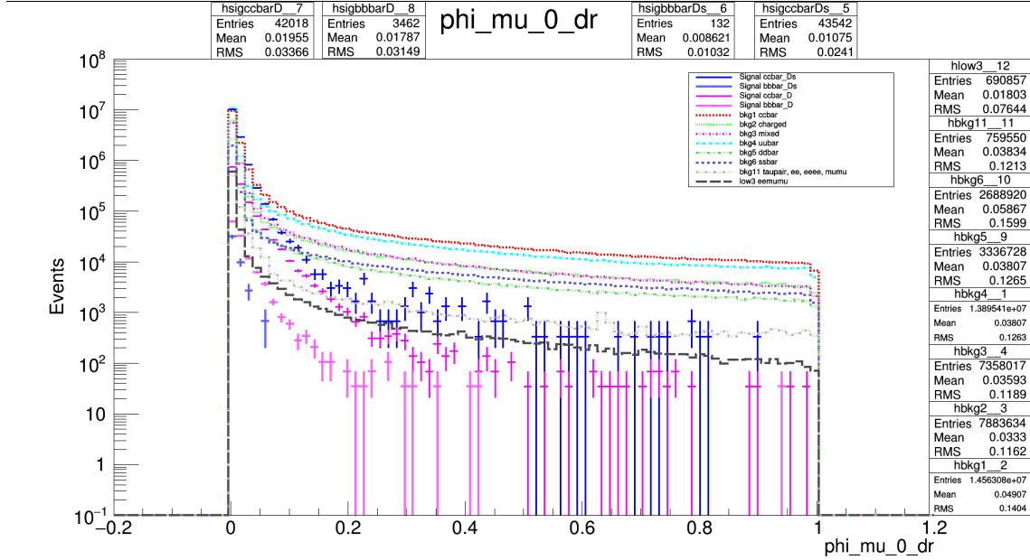
Figura 4.13: Distribución de la variable dr de uno de los muones. Las cruces azules más delgadas corresponden a nuestra señal ( candidatos a D_s^+ ) provenientes de la producción c\bar{c} mientras las cruces azules más gruesas corresponden a lo que queda de la señal proveniente de la producción b\bar{b} . Las cruces color magenta corresponden a las señales D^+ , las cruces gruesas corresponden a la producción b\bar{b} mientras a las cruces delgadas a la producción c\bar{c} . El resto de las líneas corresponden al fondo.
