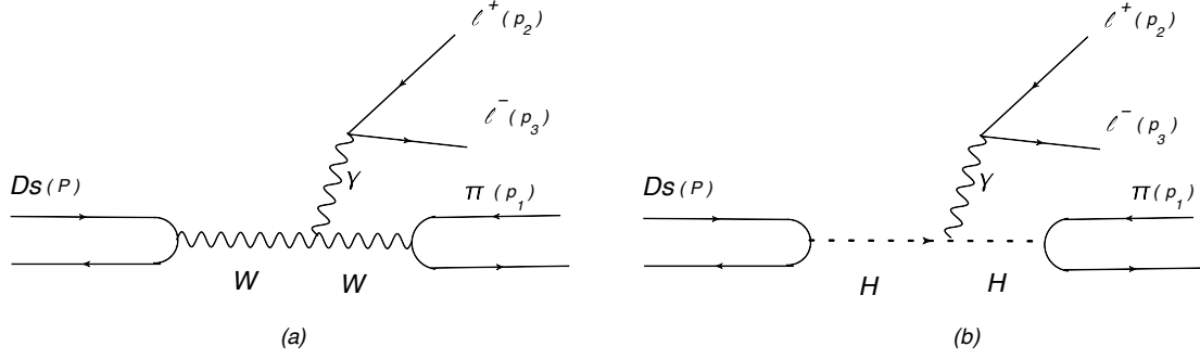
Figura 2.11: Contribución de corta distancia (SD) para el decaimiento D_s \rightarrow \pi \mu \mu en el (a) ME y (b) 2HDM-II.
