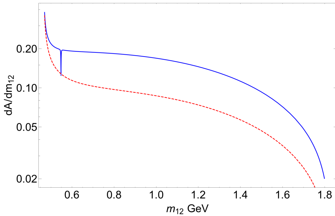
Figura 2.8: Distribución dA/m_{12} = A_{FB}|_{\cos\theta} para \cos\theta = 0.1 (línea sólida azul) obtenida de la contribución LD, comparada con la estimación puramente de espacio fase (línea punteada roja).
