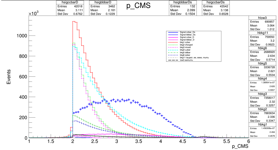
Figura 4.4: Distribución de la variable p_{CMS} . Las cruces azules más delgadas corresponden a nuestra señal ( candidatos a D_s^+ ) provenientes de la producción c\bar{c} mientras las cruces azules mas gruesas corresponden a lo que queda de la señal proveniente de la producción b\bar{b} . Las cruces color magenta corresponden a las señales D^+ , las cruces gruesas corresponden a la producción b\bar{b} mientras a las cruces delgadas a la producción c\bar{c} . El resto de las líneas corresponden al fondo.
