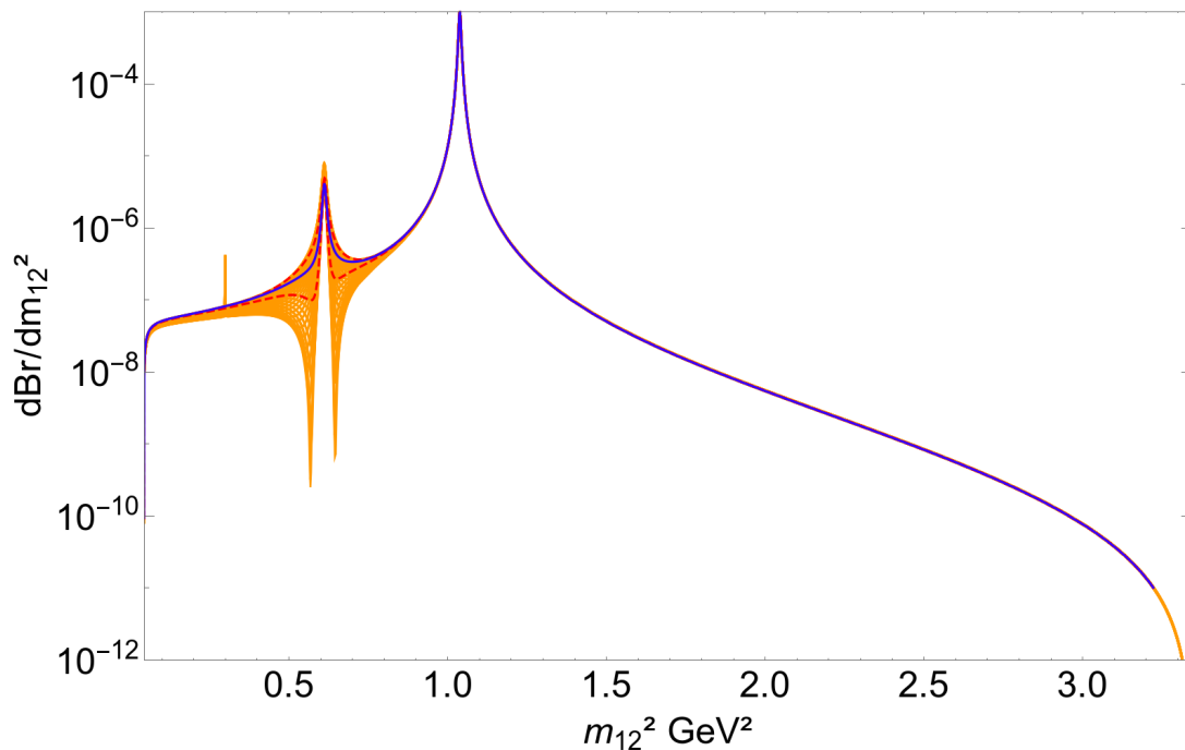
Figura 2.4: Masa invariante del dimuón para el decaimiento D_s^+ \rightarrow \pi^+ \mu^+ \mu^- obtenidos de las contribuciones de larga distancia. El área sombreada (color naranja) corresponde a la región permitida para la fase relativa \delta_{\rho\phi} , mientras que las líneas punteadas (rojas) limitan la región a una sigma del valor central de \delta_{\rho\phi} (línea sólida azul) obtenida del ajuste a los datos de LHCb.
