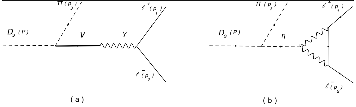
Figura 2.1: Contribución de Larga Distancia (LD) para el decaimiento D_s \rightarrow \pi \ell^- \ell^+ , mediado por un mesón vectorial (a) y un mesón pseudo-escalar (b).
