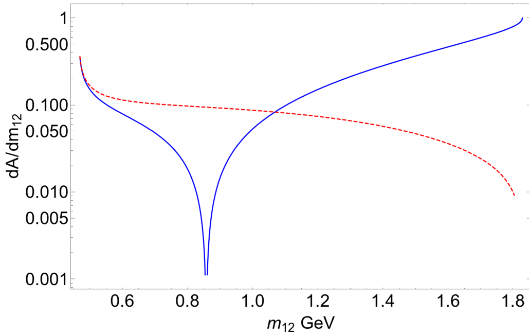
Figura 2.14: Distribución de A_{FB}|_{\cos\theta} para 2HDM-II a \cos\theta = 0.1 (línea sólida), comparada con la estimación puramente del espacio fase (línea punteada).
