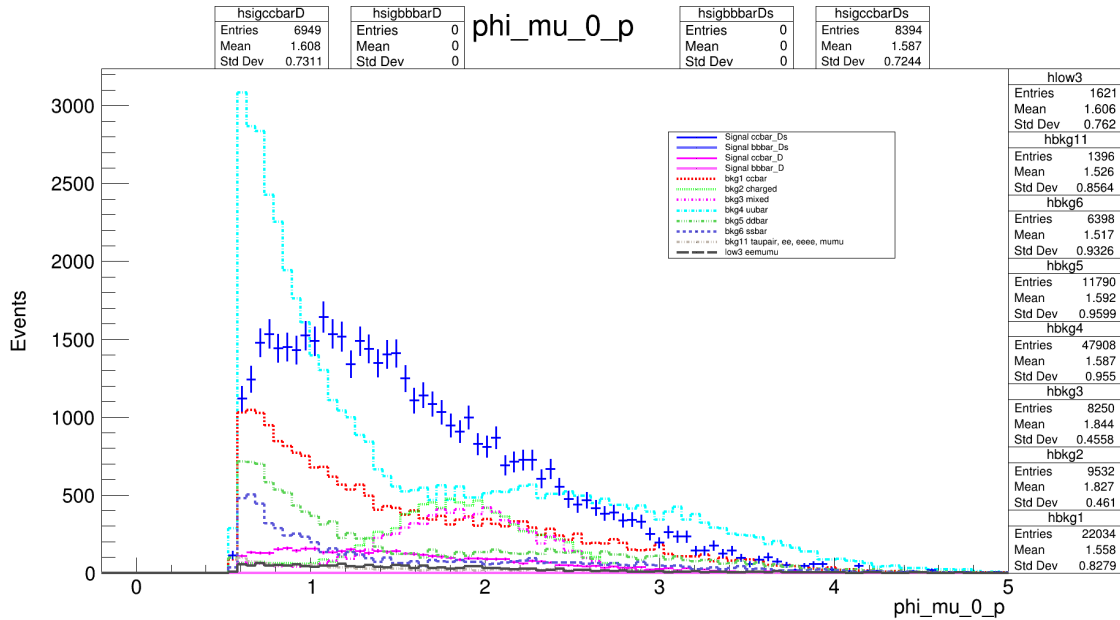
Figura 4.18: Distribución de la variable \mu\_p después de optimización. Las cruces azules corresponden a nuestra señal (candidatos a D_s^+ ) provenientes de la producción c\bar{c} . Las cruces color magenta corresponden a la señal D^+ provenientes de la producción c\bar{c} . El resto de las líneas corresponden al fondo.
