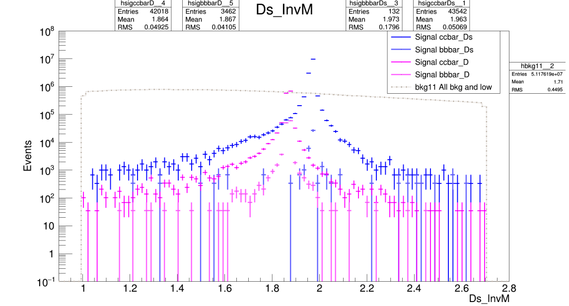
Figura 4.23: Distribución de la masa invariante de \pi^+ \mu^+ \mu^- después de preselección. Las cruces azules corresponden a nuestra señal (candidatos a D_s^+ ) provenientes de la producción c\bar{c} . Las cruces color magenta corresponden a la señal D^+ provenientes de la colisión c\bar{c} . La línea punteada corresponde a todo el fondo sumado. Se incluye la señal de b\bar{b} remanente con línea delgada azul y magenta.
