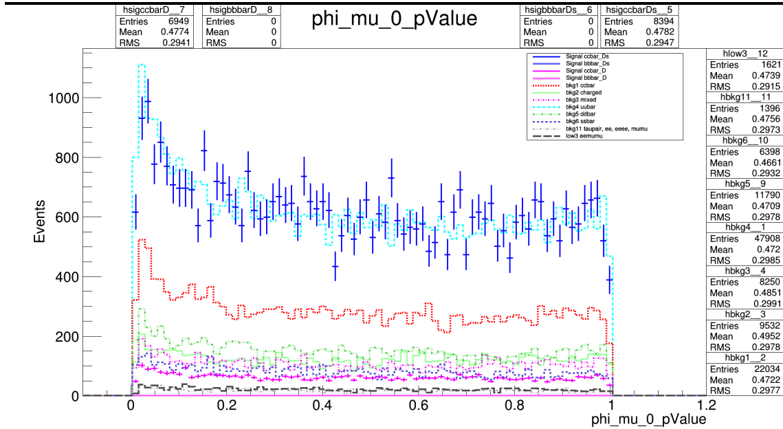
Figura 4.21: Distribución de la variable \mu\_pValue después de optimización. Las cruces azules corresponden a nuestra señal (candidatos a D_s^+ ) provenientes de la producción c\bar{c} . Las cruces color magenta corresponden a la señal D^+ provenientes de la producción c\bar{c} . El resto de las líneas corresponden al fondo.
