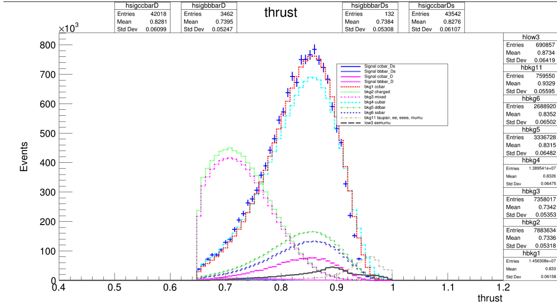
Figura 4.9: Distribución de la variable "thrust". Las cruces azules más delgadas corresponden a nuestra señal ( candidatos a D_s^+ ) provenientes de la producción c\bar{c} mientras las cruces azules mas gruesas corresponden a lo que queda de la señal proveniente de la producción b\bar{b} . Las cruces color magenta corresponden a las señales D^+ , las cruces gruesas corresponden a la producción b\bar{b} mientras a las cruces delgadas a la producción c\bar{c} . El resto de las líneas corresponden al fondo.
