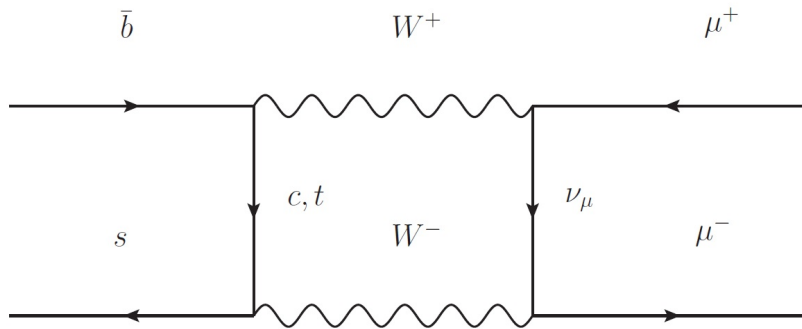
Figura 1.2: Diagrama de caja: canal W para el proceso b\bar{s} \rightarrow \mu\mu . El quark intermedio u no se considera ya que la contribución de su masa es despreciable comparada con la masa de los quarks c y t .
