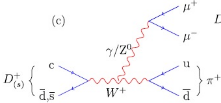
Figura 2.5: Diagrama de Feynman para la aniquilación débil de un mesón D_s^+
