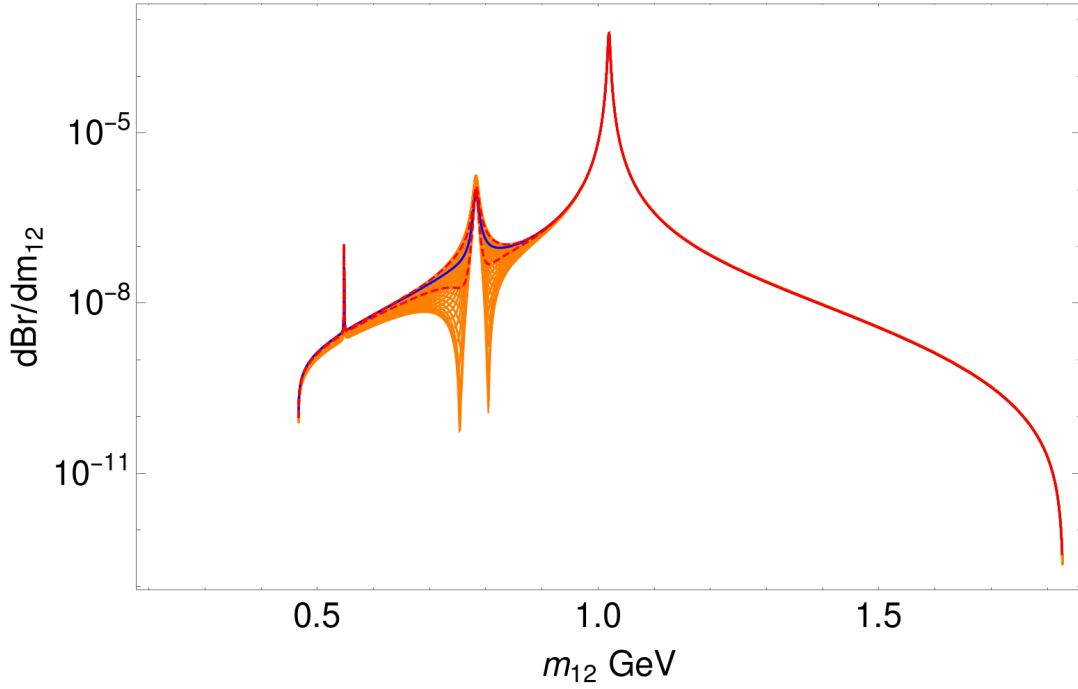
Figura 2.7: La región más favorecida cinemáticamente en la distribución de la masa invariante del di-muon m_{12} = m_{\mu\mu} , debido a las contribuciones de LD, se encuentra para \cos\theta = 0.1 (denotado como d\mathcal{B}r/dm_{12} = \frac{1}{\Gamma_{D_s}}/dm_{\mu\mu} ). El área sombreada (color naranja) corresponde a la región permitida para la fase relativa \delta_{\rho\phi} en toda el dominio, mientras que las líneas punteadas (rojo) limitan la región a 1\sigma obtenida del ajuste a los datos de LHCb para \delta_{\rho\phi} . La línea sólida (azul) corresponde al valor central del ajuste.
