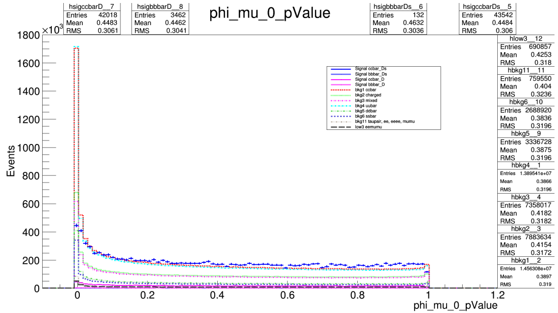
Figura 4.10: Distribución de la variable mu_pValue. Las cruces azules más delgadas corresponden a nuestra señal ( candidatos a D_s^+ ) provenientes de la producción c\bar{c} mientras las cruces azules más gruesas corresponden a lo que queda de la señal proveniente de la producción b\bar{b} . Las cruces color magenta corresponden a las señales D^+ , las cruces gruesas corresponden a la producción b\bar{b} mientras que las cruces delgadas corresponden a la producción c\bar{c} . El resto de las líneas corresponden al fondo.
