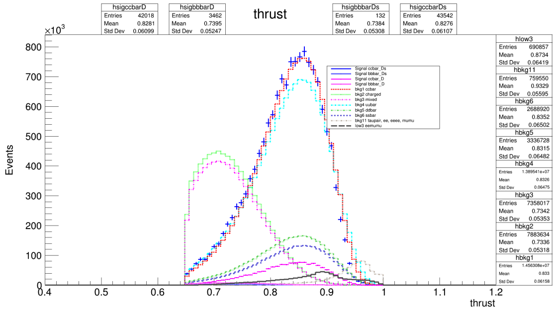
Figura 4.12: Distribución de la variable "thrust". Las cruces azules más delgadas corresponden a nuestra señal ( candidatos a D_s^+ ) provenientes de la producción c\bar{c} mientras las cruces azules mas gruesas corresponden a lo que queda de la señal proveniente de la producción b\bar{b} . Las cruces color magenta corresponden a las señales D^+ , las cruces gruesas corresponden a la producción b\bar{b} mientras a las cruces delgadas a la producción c\bar{c} . El resto de las líneas corresponden al fondo.
