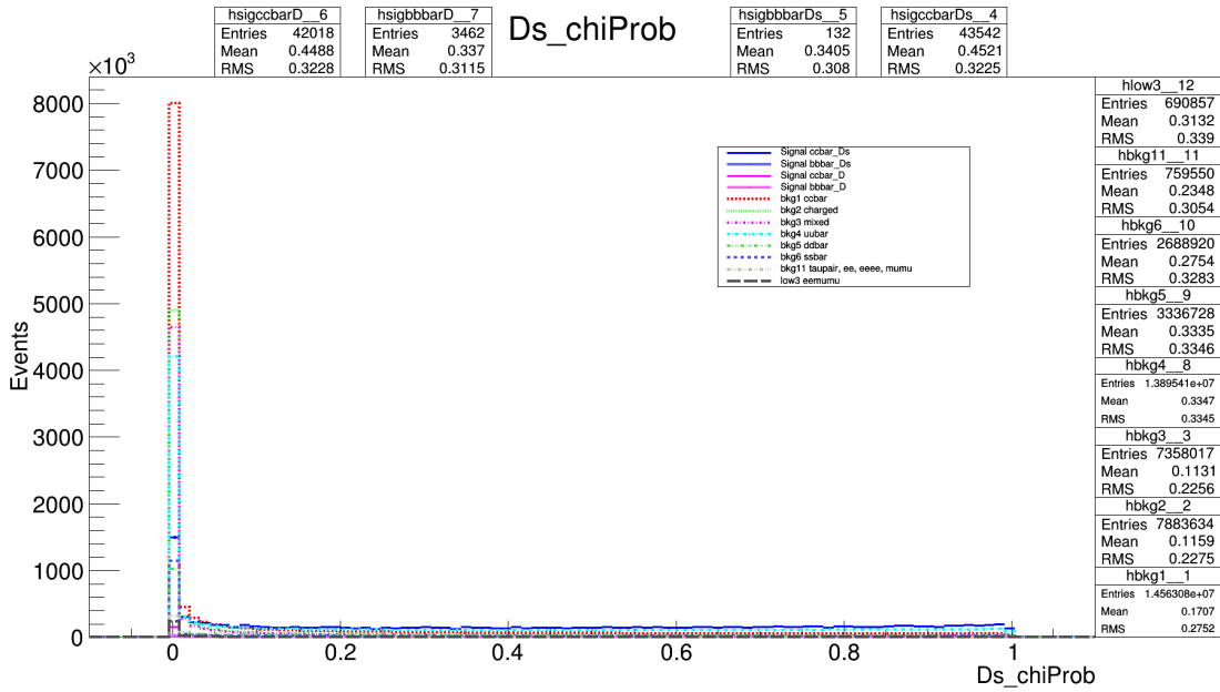
Figura 4.5: Distribución de la variable Ds\_chiProb . Las cruces azules más delgadas corresponden a nuestra señal ( candidatos a D_s^+ ) provenientes de la producción c\bar{c} mientras las cruces azules mas gruesas corresponden a lo que queda de la señal proveniente de la producción b\bar{b} . Las cruces color magenta corresponden a las señales D^+ , las cruces gruesas corresponden a la producción b\bar{b} mientras a las cruces delgadas a la producción c\bar{c} . El resto de las líneas corresponden al fondo.
