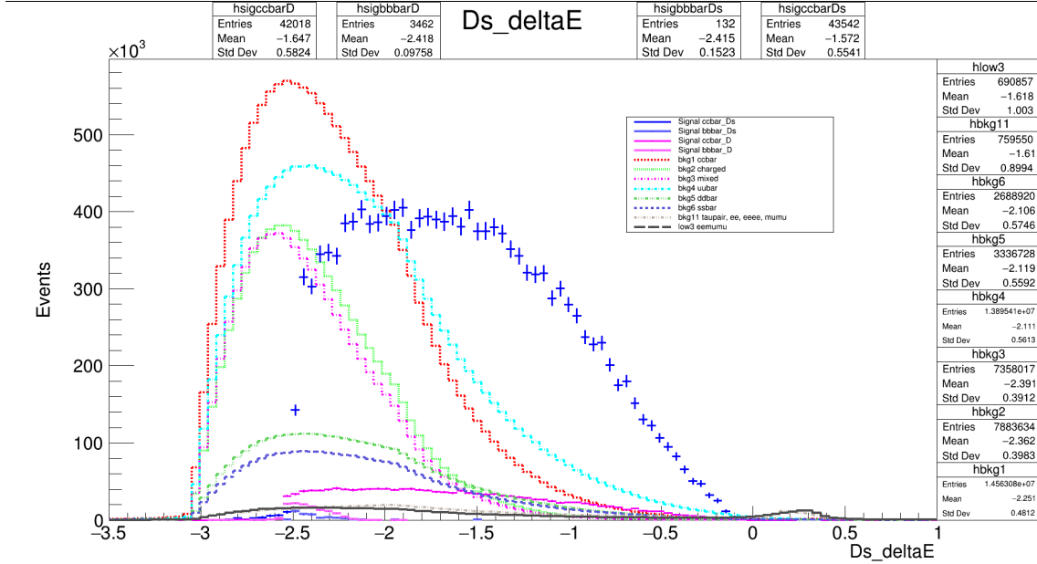
Figura 4.11: Distribución de la variable D_s\_deltaE\_high . Las cruces azules más delgadas corresponden a nuestra señal ( candidatos a D_s^+ ) provenientes de la producción c\bar{c} mientras las cruces azules mas gruesas corresponden a lo que queda de la señal proveniente de la producción b\bar{b} . Las cruces color magenta corresponden a las señales D^+ , las cruces gruesas corresponden a la producción b\bar{b} mientras a las cruces delgadas a la producción c\bar{c} . El resto de las líneas corresponden al fondo.
