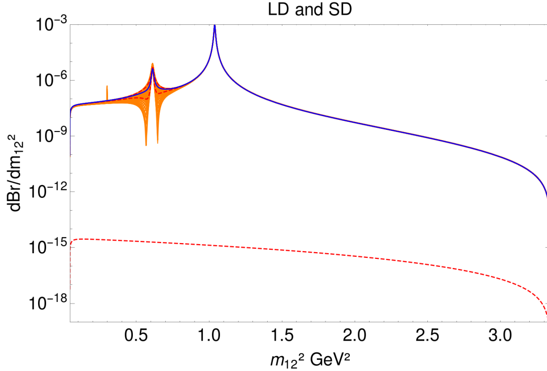
Figura 2.6: Comparación de las contribuciones de larga (línea sólida azul y área naranja) y corta (punteada roja) distancia al proceso: D_s \rightarrow \pi \ell^+ \ell^- . El área sombreada (color naranja) de la contribución de larga distancia corresponde como en la figura anterior, a la región permitida para la fase relativa \delta_{\rho\phi} y las líneas punteadas así como la línea azul corresponde a los errores y el valor central de la fase obtenida por el ajuste a los datos.
