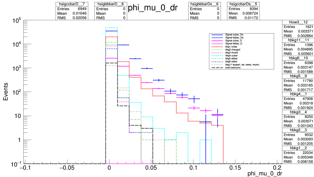
Figura 4.22: Distribución de la variable \mu_\text{on\_dr} después de optimización. Las cruces azules corresponden a nuestra señal (candidatos a D_s^+ ) provenientes de la producción c\bar{c} . Las cruces color magenta corresponden a la señal D^+ provenientes de la producción c\bar{c} . El resto de las líneas corresponden al fondo.
