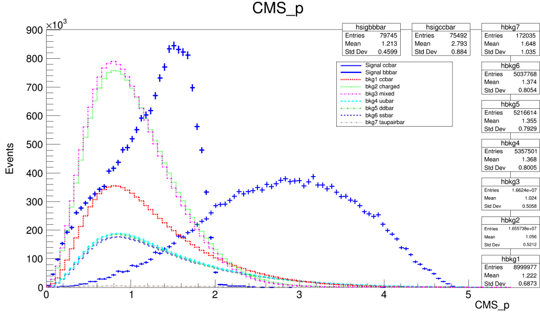
Figura 4.1: Distribución de la variable CMS\_p . Las cruces azules corresponden a nuestra señal (candidatos a D_s^+ ) provenientes de c\bar{c} y b\bar{b} , la última decayendo abruptamente alrededor de los 2 GeV/c.
