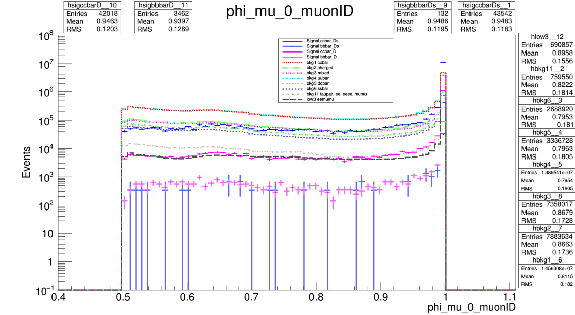
Figura 4.3: Distribución de la variable muonID. Las cruces azules más delgadas corresponden a nuestra señal ( candidatos a D_s^+ ) provenientes de la producción c\bar{c} mientras las cruces azules más gruesas corresponden a lo que queda de la señal proveniente de la producción b\bar{b} . Las cruces color magenta corresponden a las señales D^+ , las cruces gruesas corresponden a la producción b\bar{b} mientras a las cruces delgadas a la producción c\bar{c} . El resto de las líneas corresponden al fondo.
