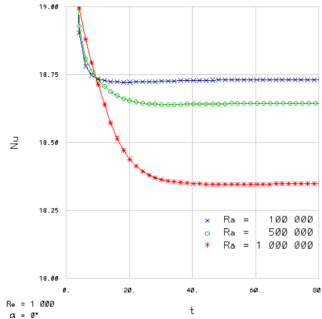
Figura 6.14: Números de Nusselt; \alpha_m = 0^\circ .
