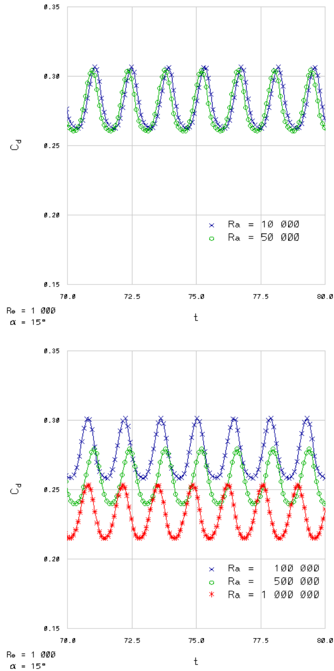
Figura 6.23: Coeficientes de arrastre; \alpha_m = 15^\circ .
