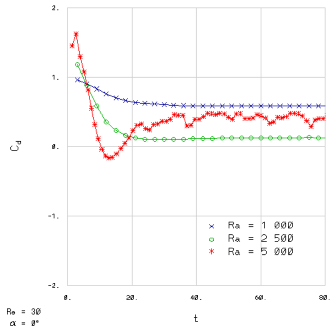
Figura 6.2: Coeficientes de arrastre; Re = 30 .
