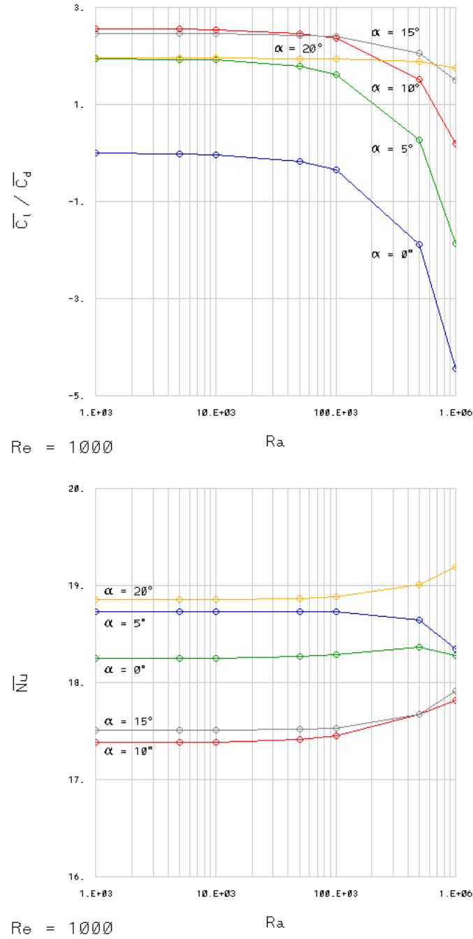
Figura 6.31: Influencia del número de Rayleigh; variación de \alpha_m .
