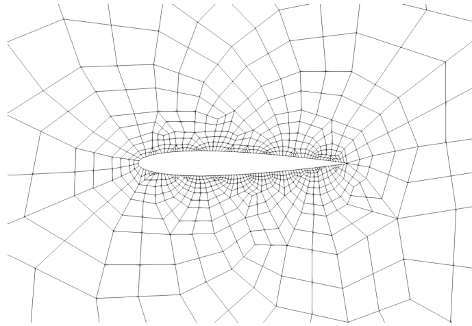
Figura 4.1: Malla original, acercamiento al perfil aerodinámico.
