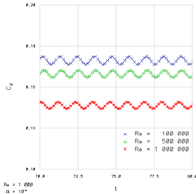
Figura 6.18: Coeficientes de arrastre; \alpha_m = 10^\circ .
