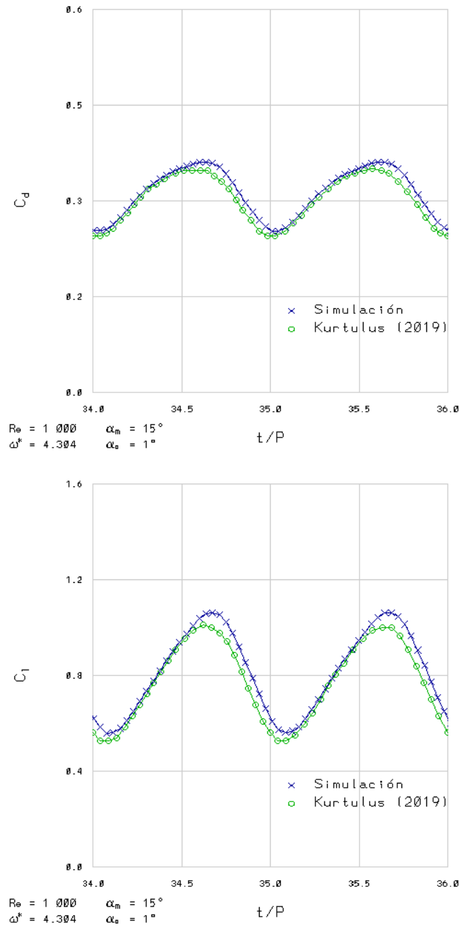
Figura 5.7: Validación de los coeficientes aerodinámicos; \alpha_m = 15^\circ, \omega^* = 4.304 .
