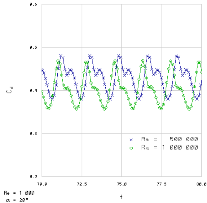
Figura 6.27: Coeficientes de arrastre; \alpha_m = 20^\circ .
