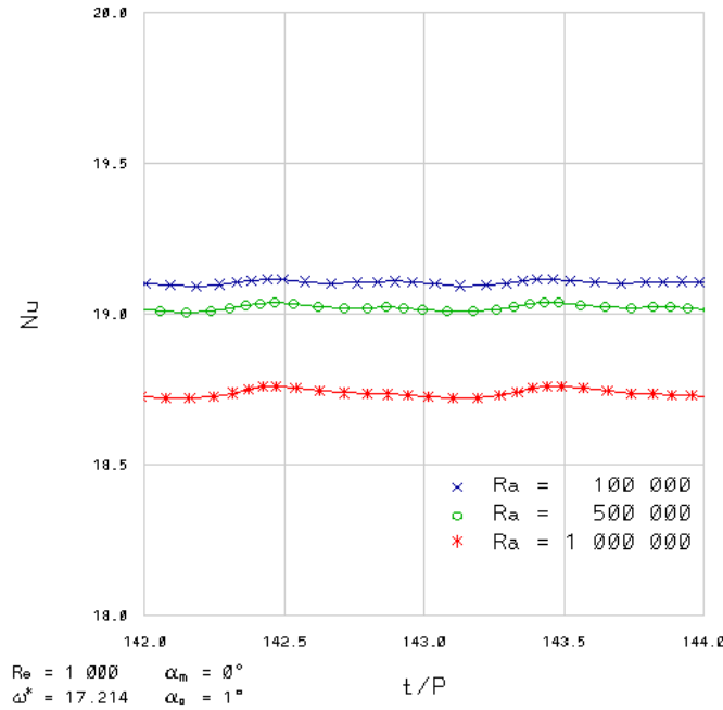
Figura 6.39: Números de Nusselt; \alpha_m = 0^\circ, \omega^* = 17.214 .
