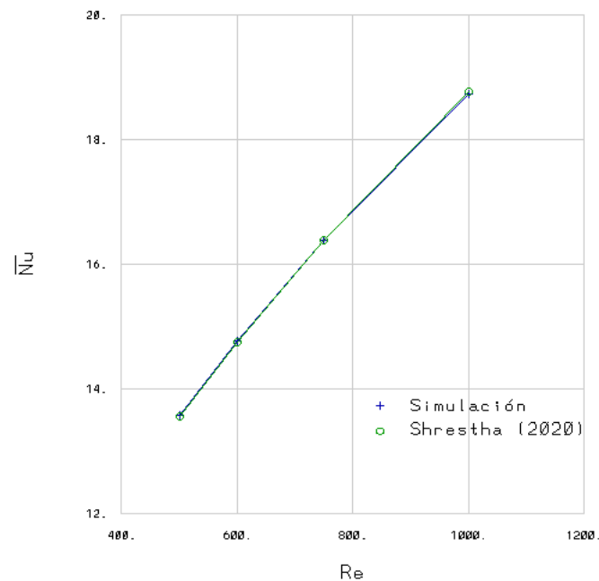
Figura 5.12: Validación del número de Nusselt; caso estático.
