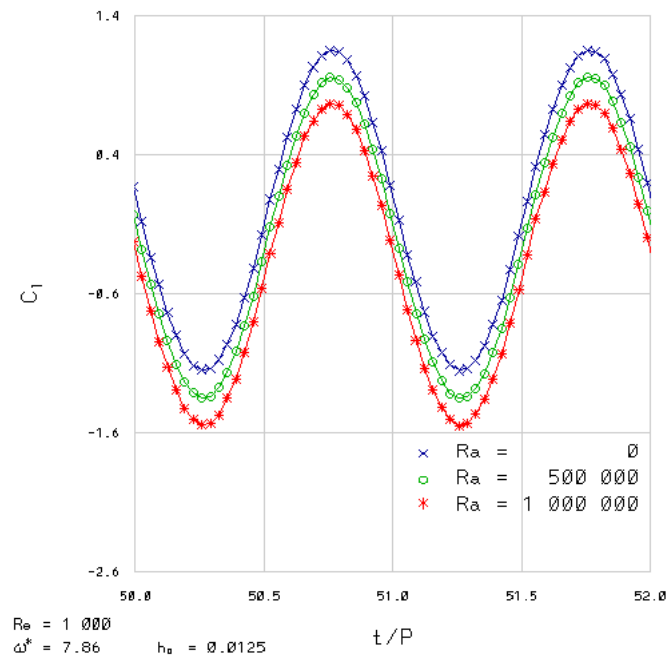
Figura 6.50: Coeficientes de sustentación; plunging .
