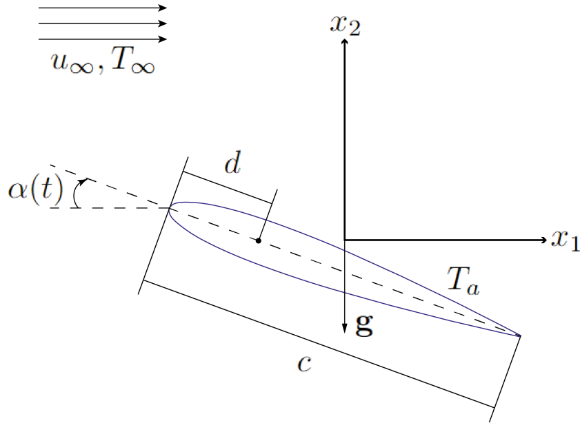
Figura 2.2: Esquema del perfil con movimiento de pitching .
