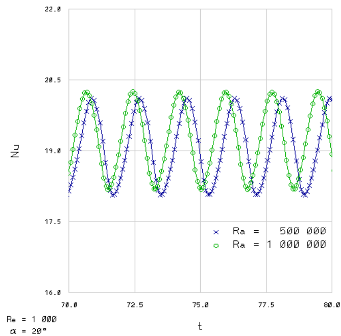
Figura 6.29: Números de Nusselt; \alpha_m = 20^\circ .
