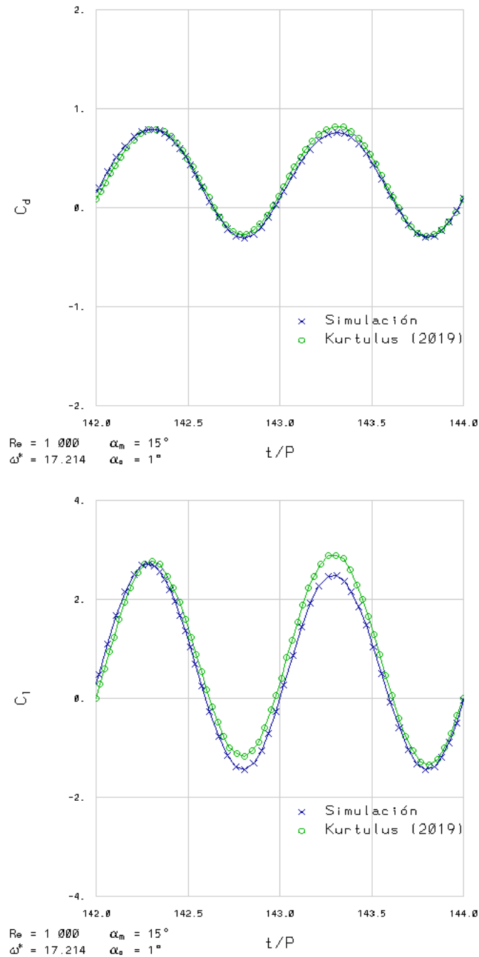
Figura 5.8: Validación de los coeficientes aerodinámicos; \alpha_m = 15^\circ , \omega^* = 17.214 .
