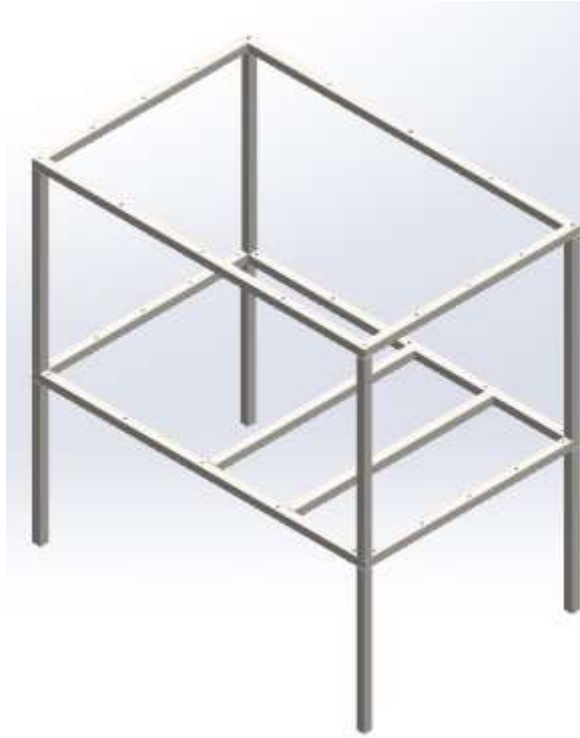
Imagen 127 PTR con el que se forma la estructura de la BCG 3 TR (elaboración propia)
