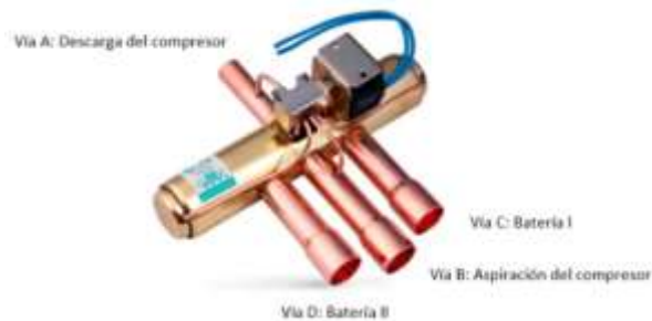
Imagen 28 Válvula de cuatro vías (Ibérica, 2016)
