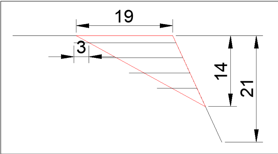
Fig. 11 Dimensiones del talud en metros. Propuesta 4, cara frontal (superior) y lateral (inferior).
