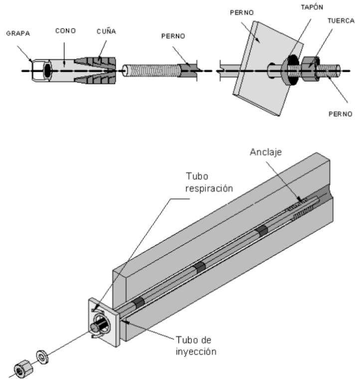
Fig. 5 Perno de anclaje puntual mecánico (Hoek & Brown, 1980).
