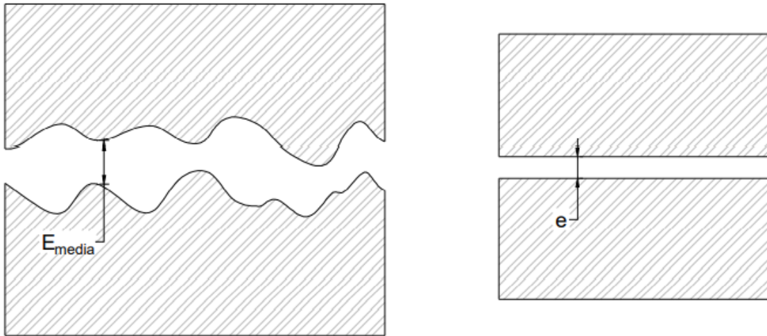
Fig. 2 Apertura eficaz o equivalente (Barton, 2004)
