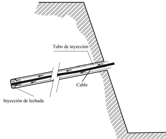
Fig. 6 Inyección de la lechada
