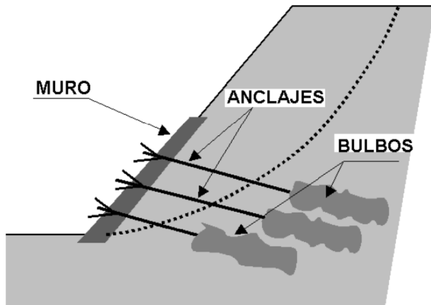
Fig. 7 Anclaje de muro
