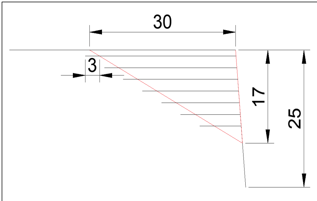
Fig. 10 Dimensiones del talud en metros. Propuesta 1, cara frontal (superior) y lateral (inferior).
