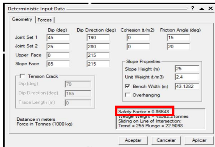
Fig. 9 Cuadro de datos del programa Swedge en donde se muestra el F.S. en el cuadro rojo. Elaboración propia.
