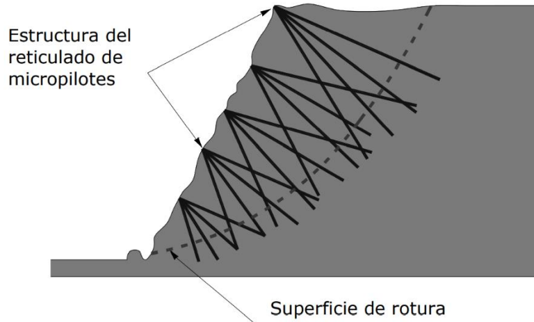
Fig. 3 Cosido de un deslizamiento con micropilotes (González de Vallejo, 2002)
