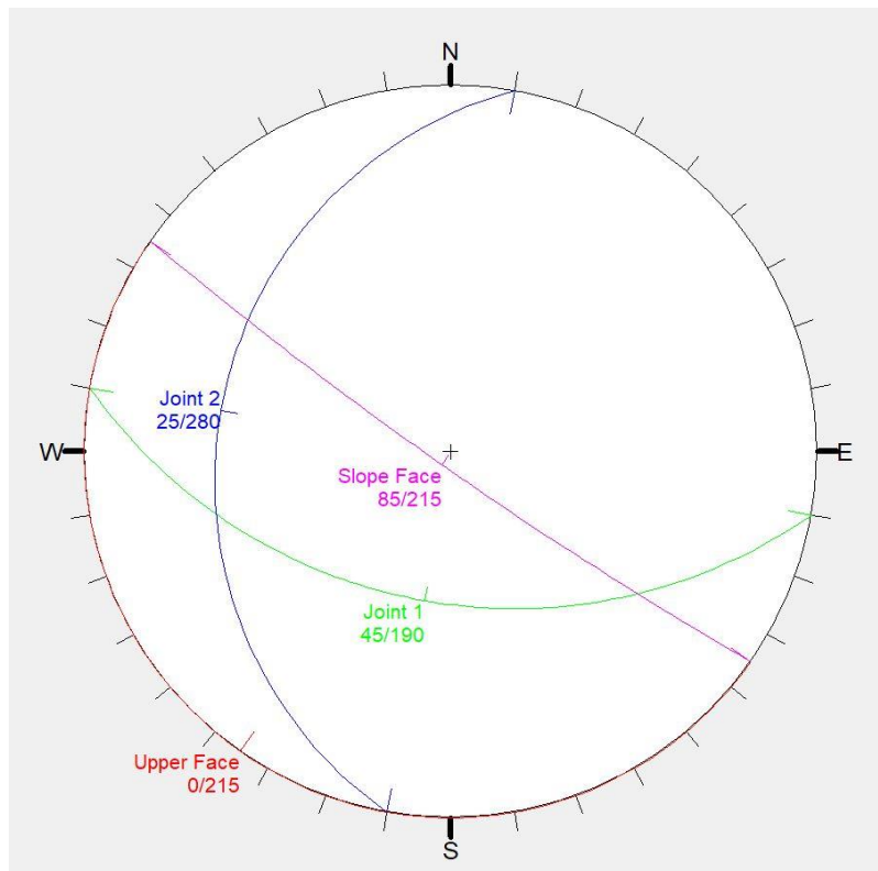
Fig.8 Proyección estereográfica de la formación de la cuña.
