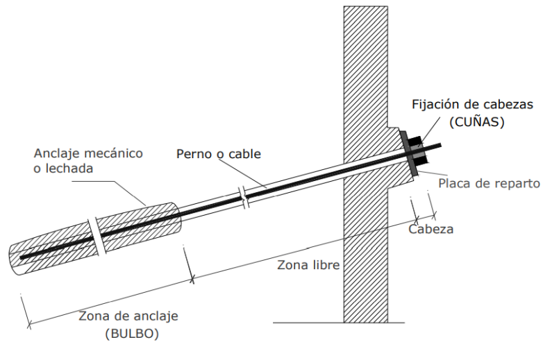
Fig. 4 Elementos de un anclaje (ministerio de Fomento, 2001)
