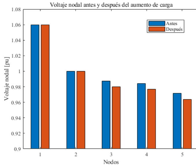
Figura 4.3. Comparación de voltaje nodal para el sistema de 5 nodos tras aumento del 20% de carga
