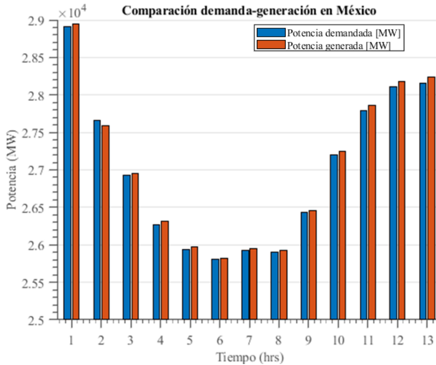
Figura 1.1. Comparación demanda-generación en México 1
