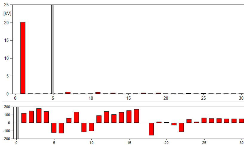
Figura 35. Espectro armónico de la señal de voltaje de la fase A.
