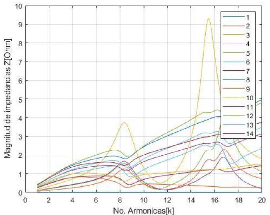
Figura 41. Barrido en frecuencia del sistema de 14 nodos IEEE.
