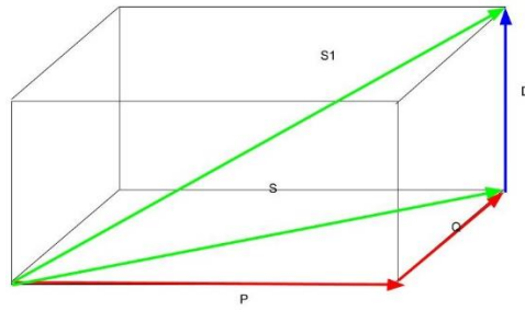
Figura 15. Triangulo de potencia (Diagrama fasorial).
