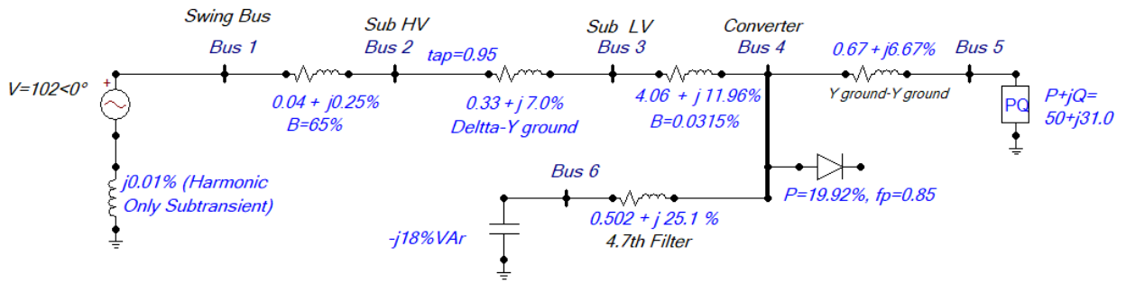
Figura 38. Diagrama unifilar de sistema de cinco nodos con filtro pasivo.
