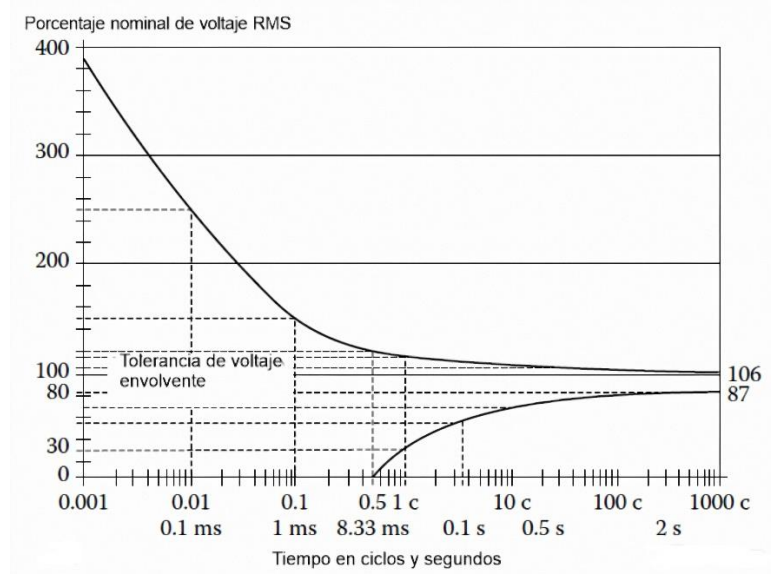
Figura 10. Curva CBEMA.
