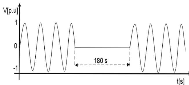
Figura 3. Interrupción de larga duración, de 3 minutos.
