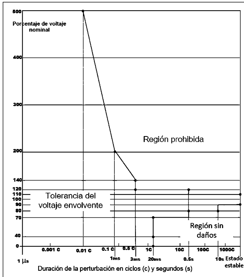
Figura 11. Curva ITIC.
