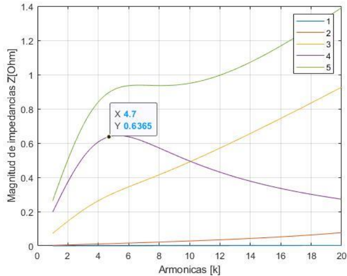
Figura 37. Barrido en frecuencias para corrección del factor de potencia en sistema de 5 nodos.
