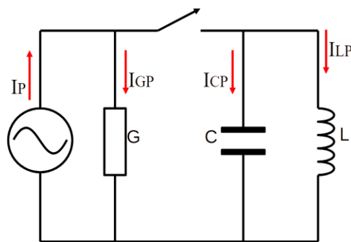
Figura 21. Circuito LC paralelo.
