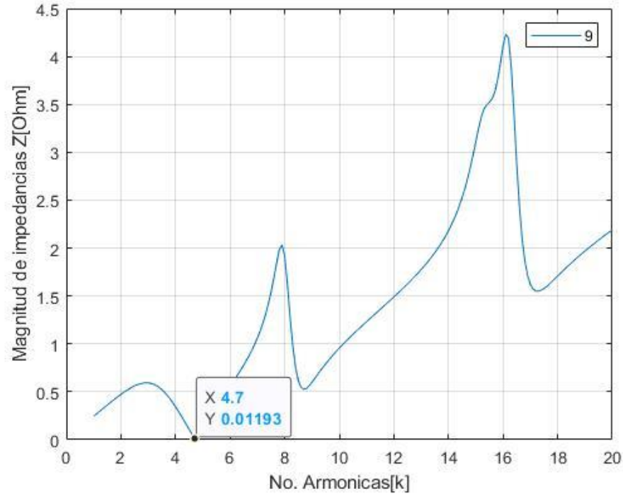
Figura 43. Mitigación del 5 o armónico para el nodo 9 del sistema de 14 nodos.
