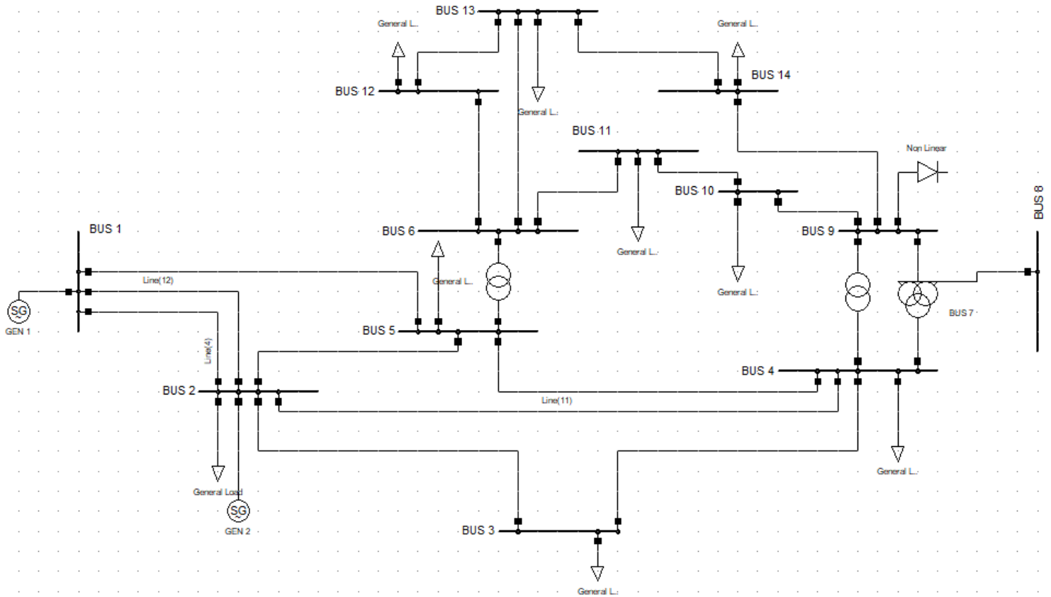
Figura 40. Sistema IEEE de 14 nodos.
