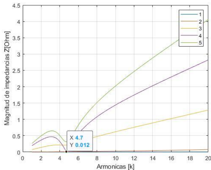
Figura 39. Mitigación del 5^{\circ} armónico.
