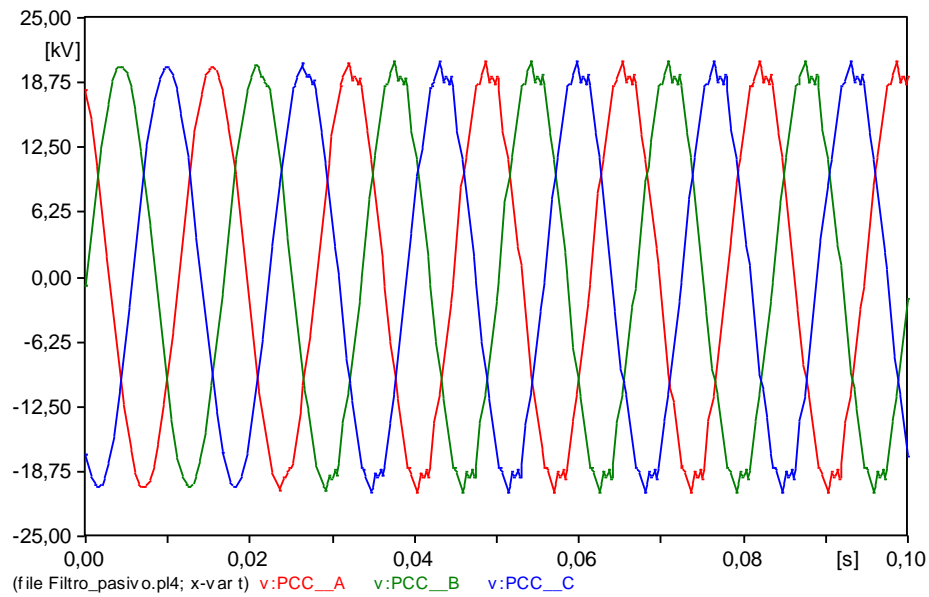
Figura 34. Señales de voltaje posterior a la implementación de un filtro pasivo para armónicos de 5 o orden en un sistema trifásico.
