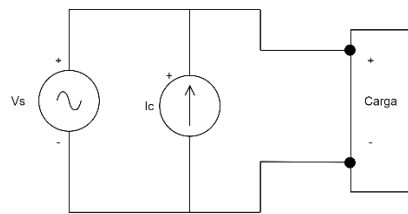
Figura 19 a) Filtro en paralelo
