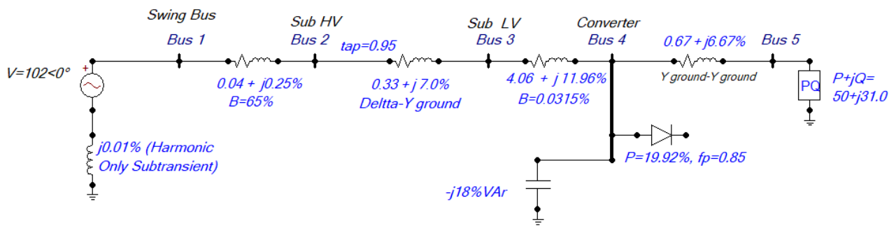
Figura 36. Diagrama Unifilar sistema 5 nodos.
