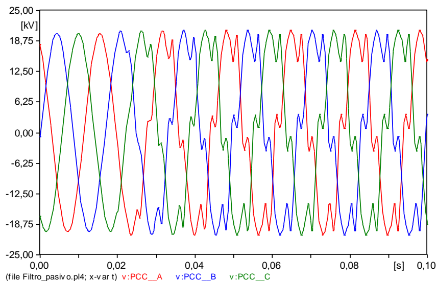
Figura 29. Señales de voltaje ante presencia de cargas no lineales en un sistema trifásico.
