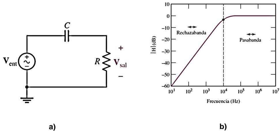
Figura 17. a) Circuito de filtro paso altas (paso altas) simple. b) Curva de respuesta de filtro paso altas. Donde cada punto corresponde a -3 dB. [37]
