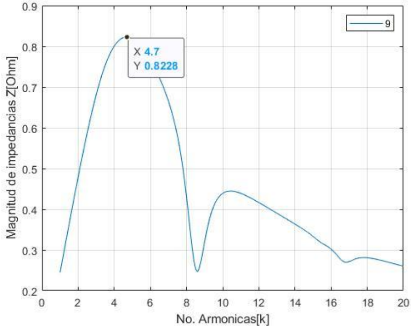
Figura 42. Barrido en frecuencia en el nodo 9 del sistema de 14 nodos.
