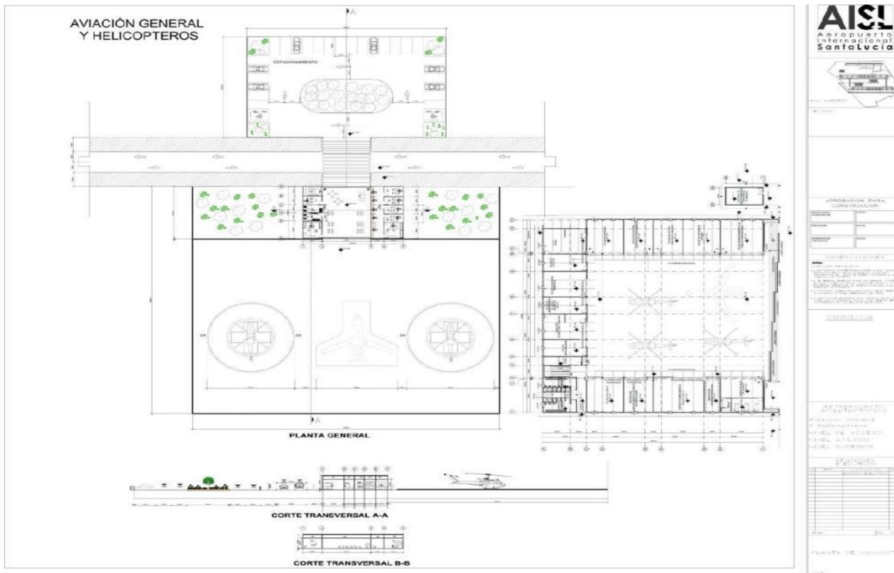
Imagen 78 Edificio de aviación general del AIFA, Proyecto arquitectónico. Planta y cortes.
