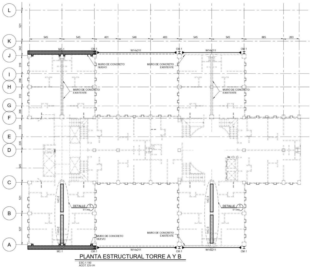
Ilustración 6 Planta general del edificio.
