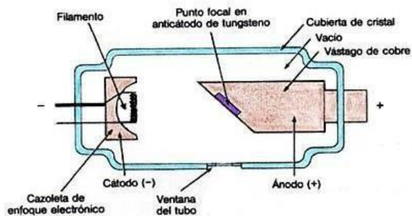
Fig. 4 Diagrama del tubo de Coolidge
