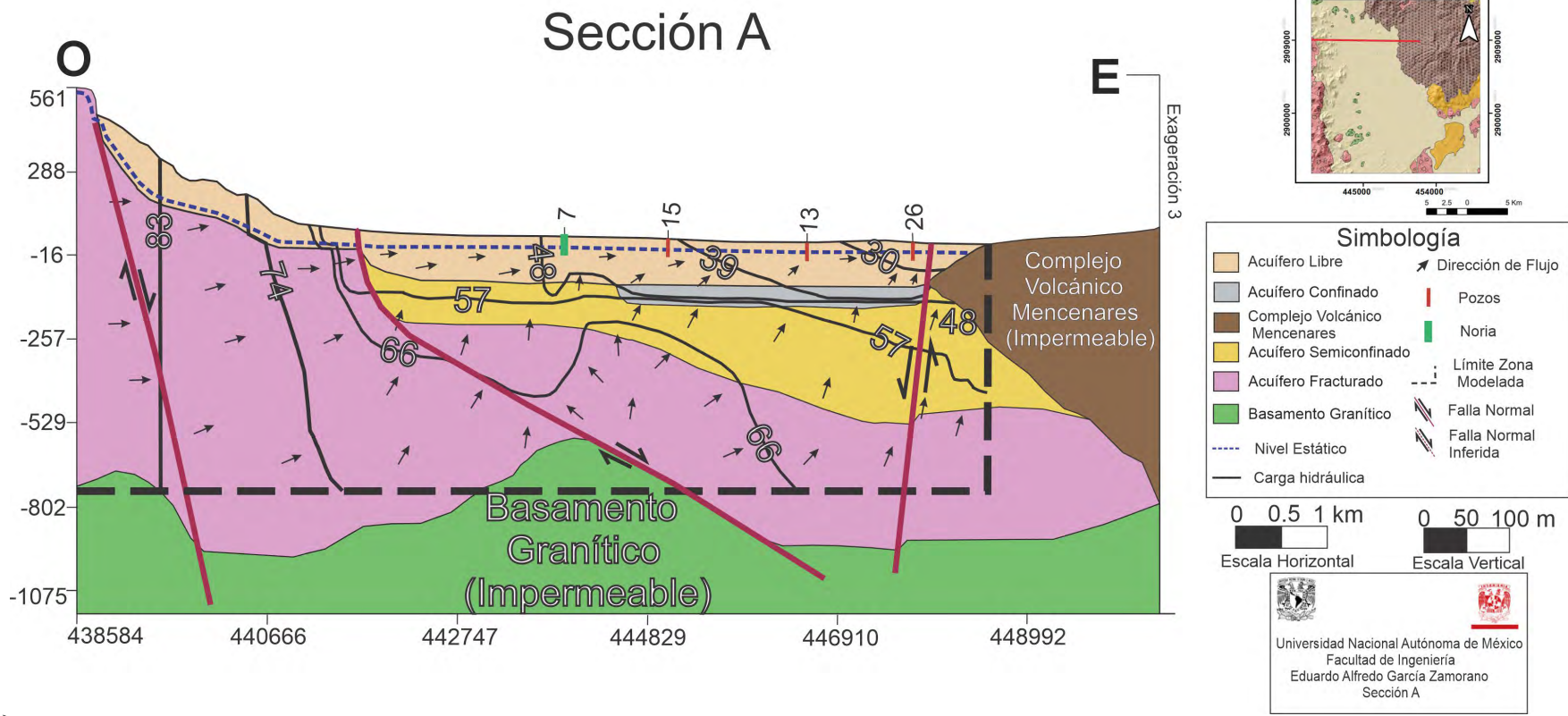
Figura 5.4: Sección hidrogeológica A.
