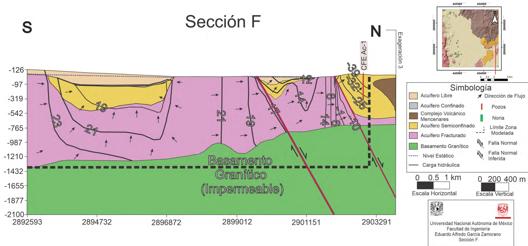
Figura 5.9: Sección hidrogeológica F.
