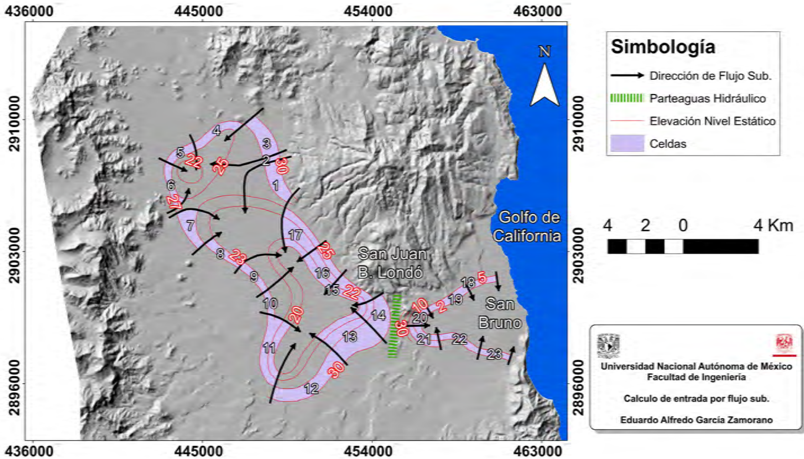
Figura 3.13: Cálculo de Flujos subterráneos para el año 2006.
