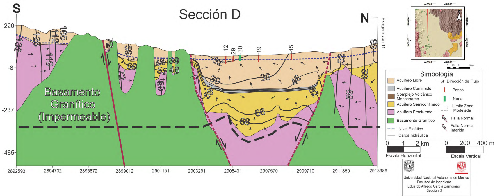
Figura 5.7: Sección hidrogeológica D.
