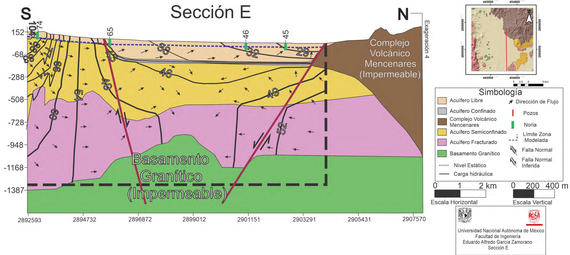
Figura 5.8: Sección hidrogeológica E.
