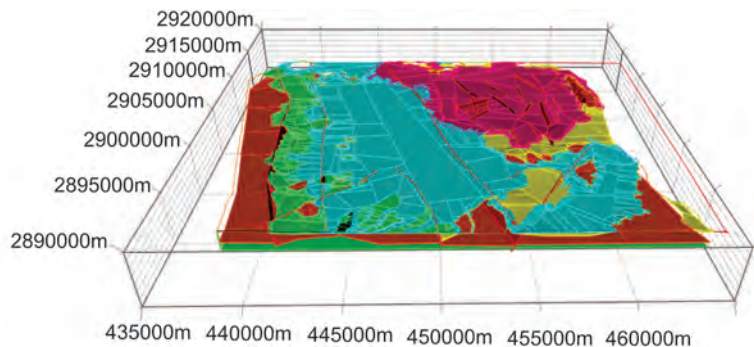
Figura 4.10: Construcción del modelo conceptual. Se muestran las bases de cada una de las unidades litológicas: En azul se observa la unidad de aluvión, en verde la unidad de Piedemonte, la amarilla la Formación Salada, la morada el Complejo Volcánico Mencenares, la café el Grupo Pre-Comondú y la verde oscuro el basamento.
