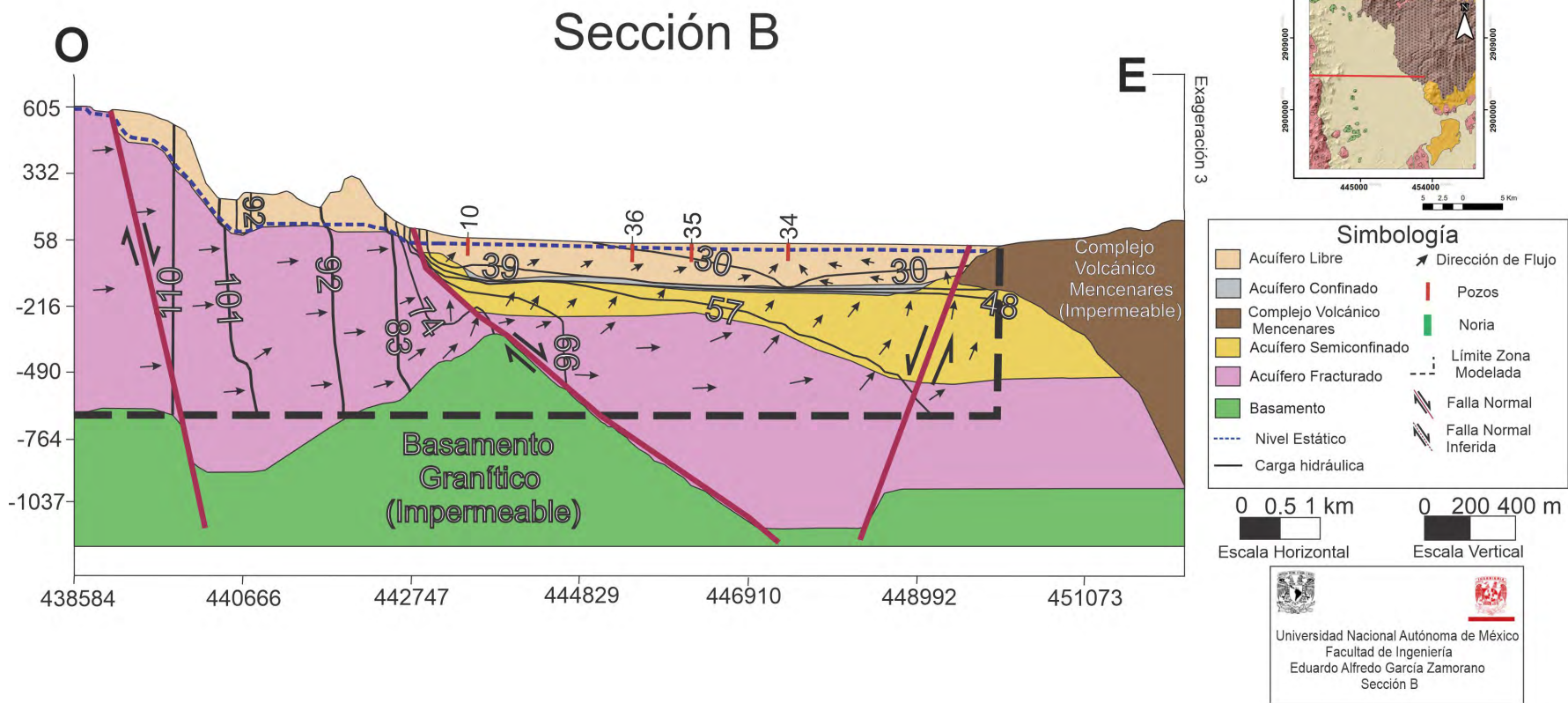
Figura 5.5: Sección hidrogeológica B.
