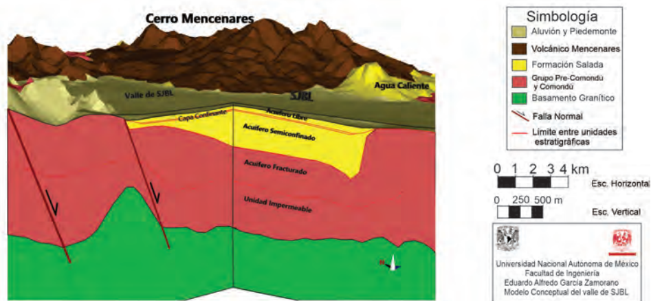
Figura 3.16: Modelo Conceptual del Valle de SJBL.
