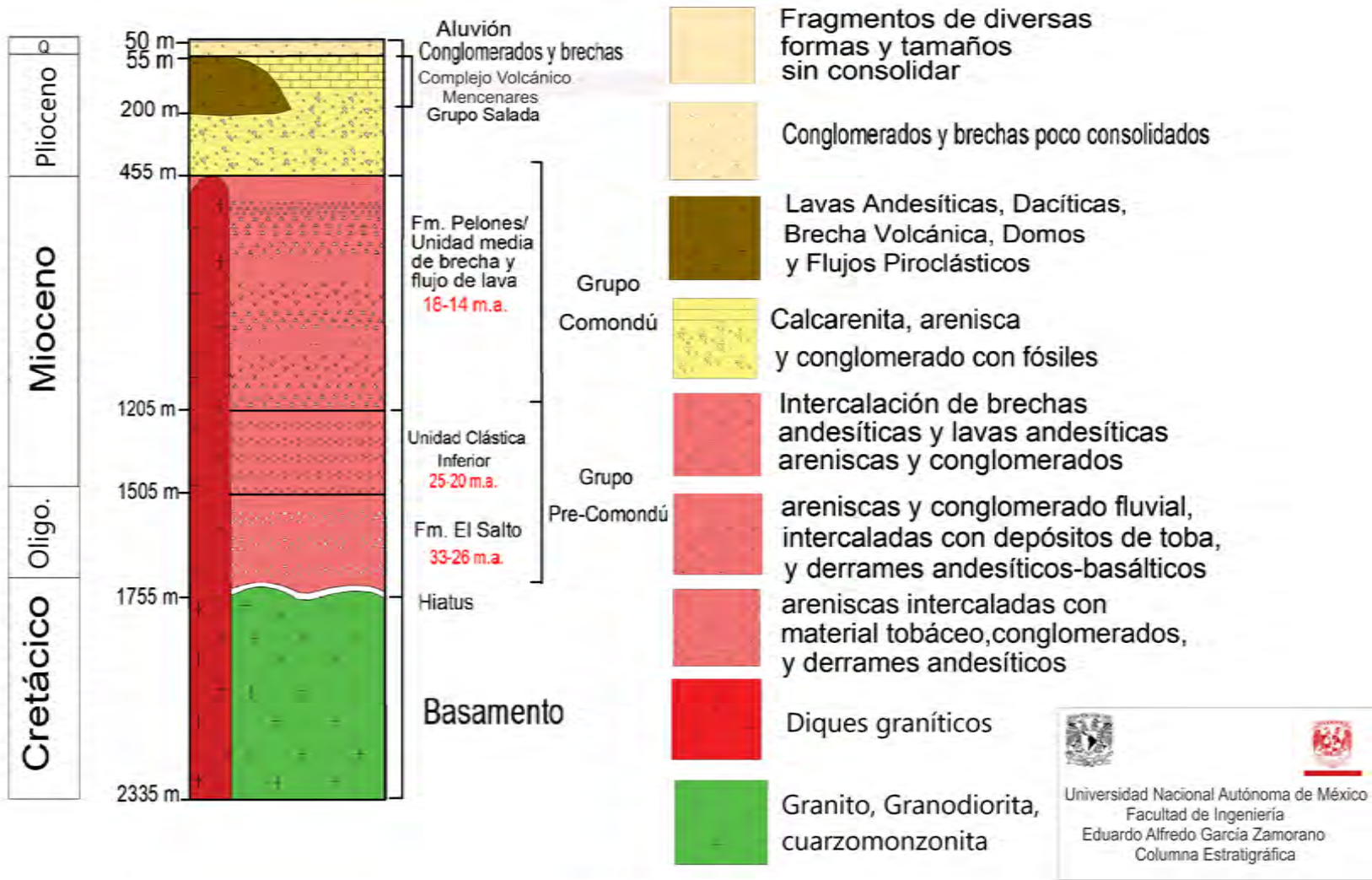
Figura 2.7: Columna estratigráfica.
