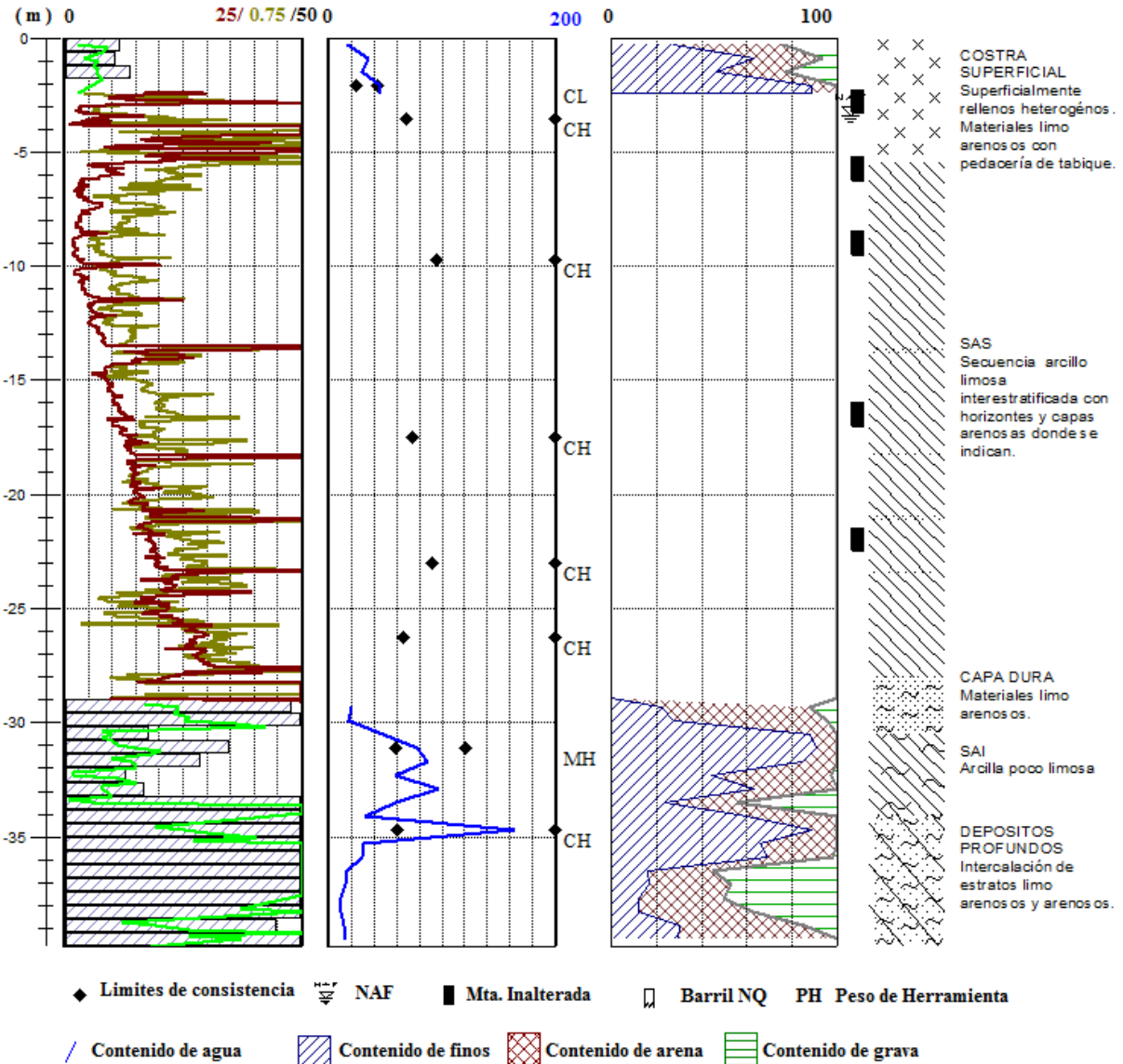
Figura 13. Perfil estratigráfico del SE-2
