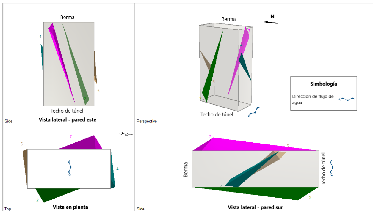
Figura 6.7 Cuñas formadas alrededor de la excavación, definidas por la cuña máxima.
