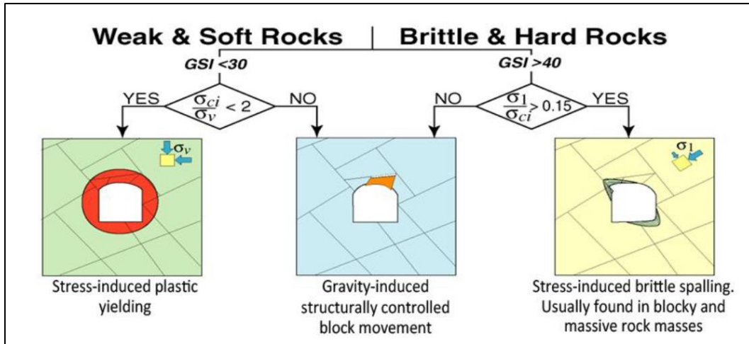
Figura 5.2 Mecanismo de inestabilidad basada en la calidad de roca GSI, resistencia de la roca intacta y nivel de esfuerzos (Martin et al. , 2003).
