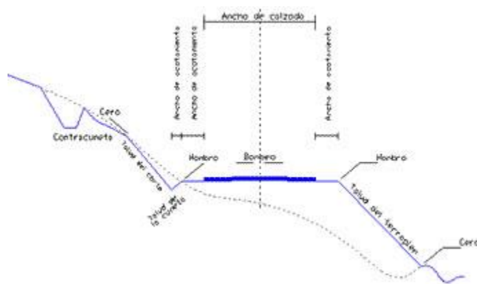
Figura 2.4.(e) Localización de una contra cuneta trapezoidal en un terreno natural fuente:
