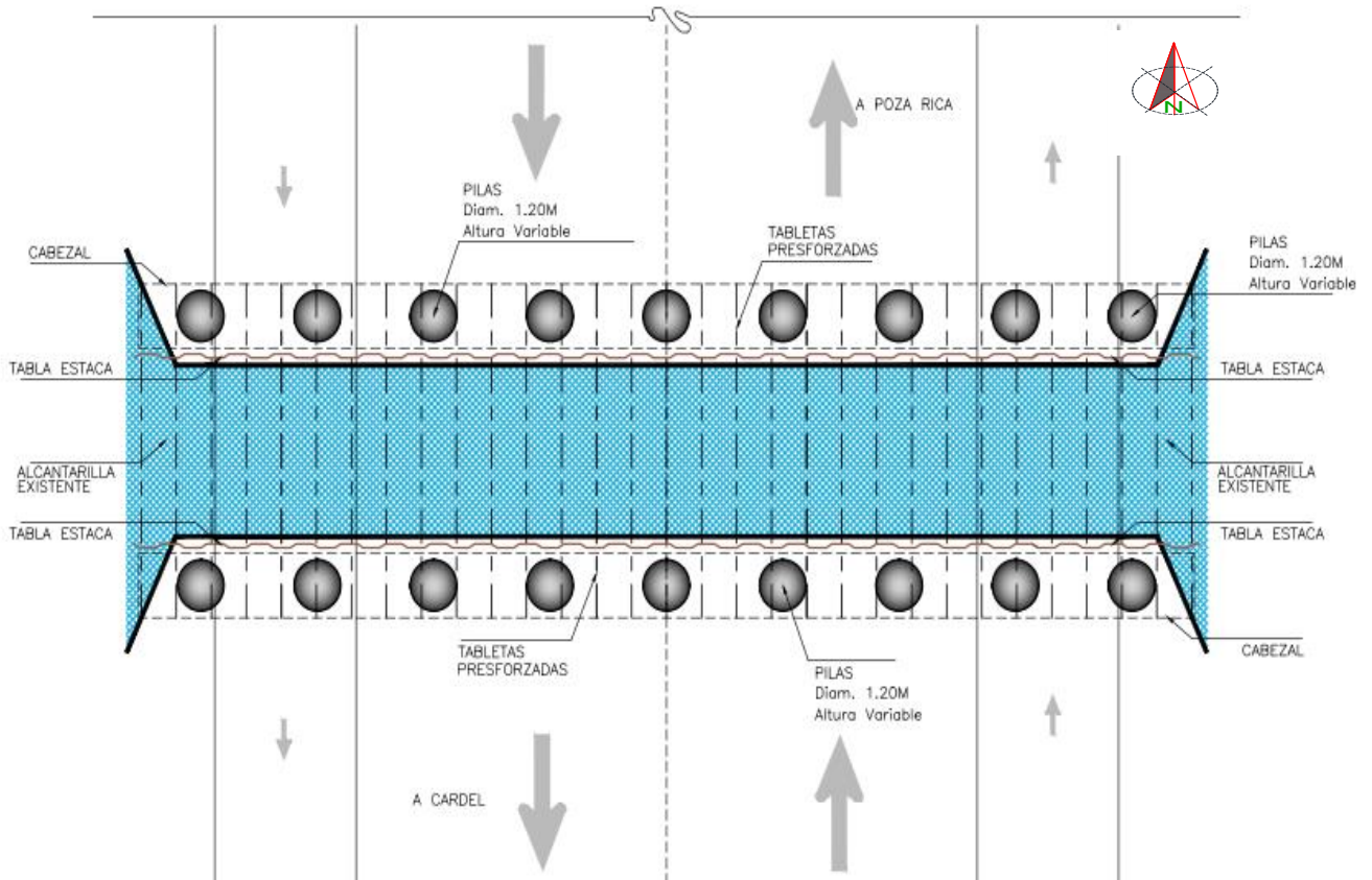
Figura 4.1 (a) Sección Planta de la alcantarilla P.S.V. San Isidro fuente obtenida por Euro estudios área de proyectos de la empresa Freyssinet de México
