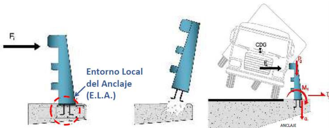
Figura 47. Fallo del entorno local del anclaje.
