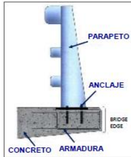
Figura 44. Representación gráfica de las partes de un parapeto
