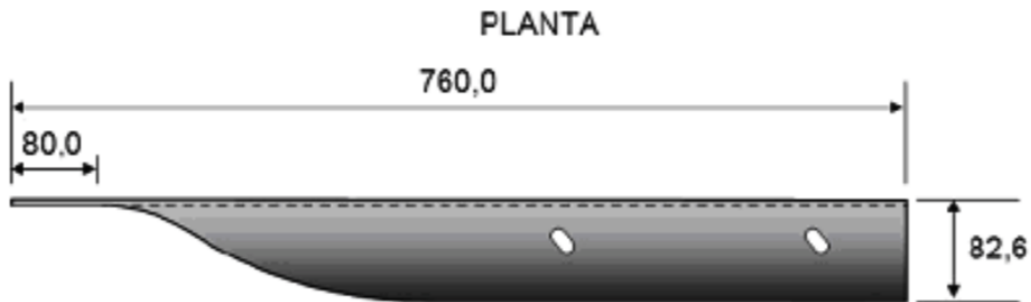
Figura 31. Vista de planta de una conexión
