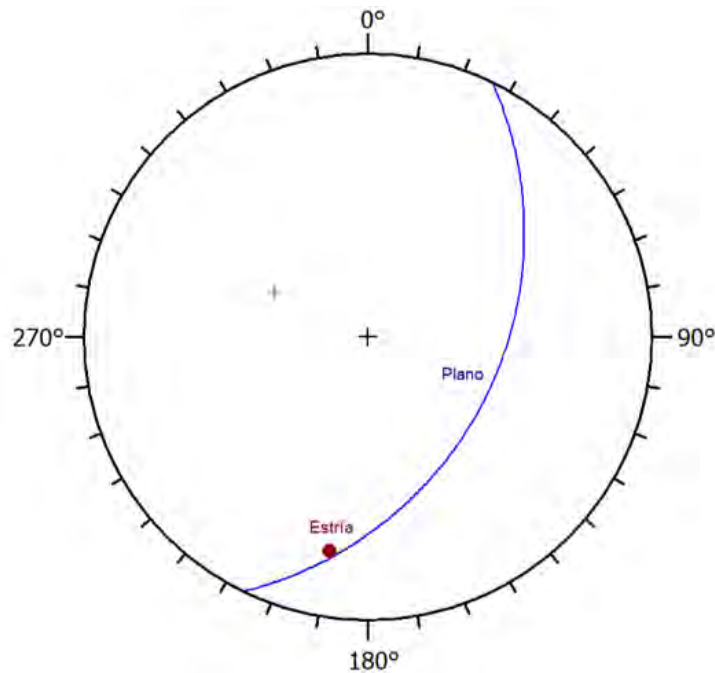
Figura 5.34: Actitud del plano de falla y estriación. Elaborado con Stereo32, 2019.
