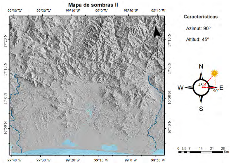
Figura 4.3: Mapa de sombras II: azimet 90^\circ y altitud 45^\circ
