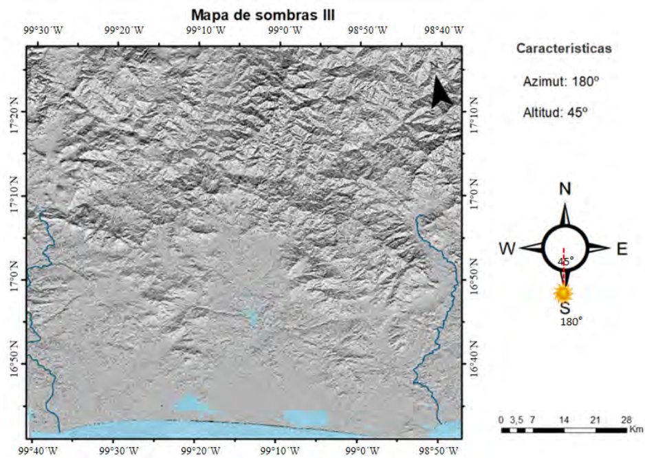
Figura 4.4: Mapa de sombras III: azimet 180^\circ y altitud 45^\circ
