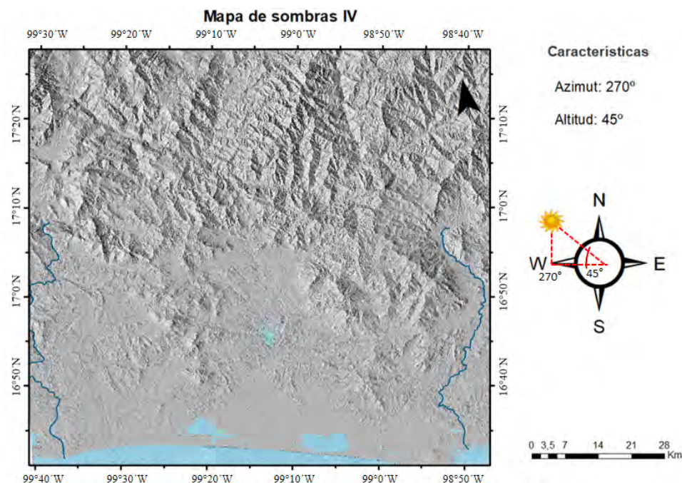
Figura 4.5: Mapa de sombras IV: azimuth 270° y altitud 45°
