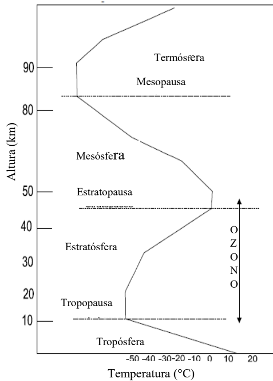
Figura 1. División de las capas de la atmósfera.
