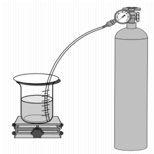
Figura 7. Esquema del sistema de burbujeo de CO 2 .
