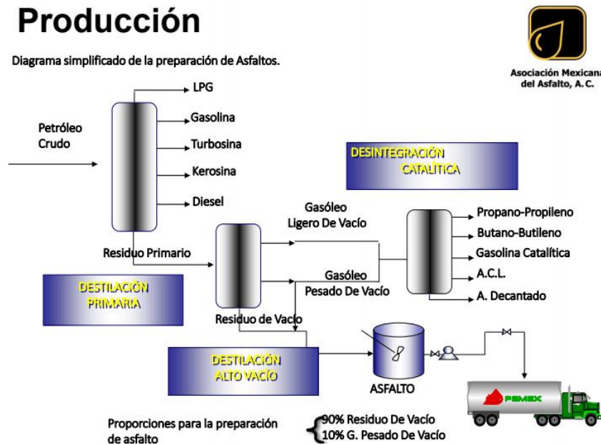
Figura 2.8.2. Diagrama del proceso de obtención del Asfalto.
