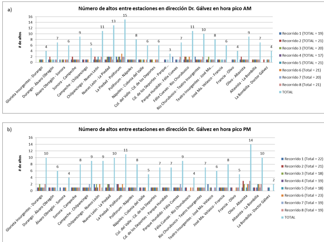
Figura 8.8: a) Número de altos a lo largo del tramo en dirección Dr. Gálvez en la hora pico matutina. b) Número de altos a lo largo del tramo en dirección Dr. Gálvez en la hora pico vespertina.
