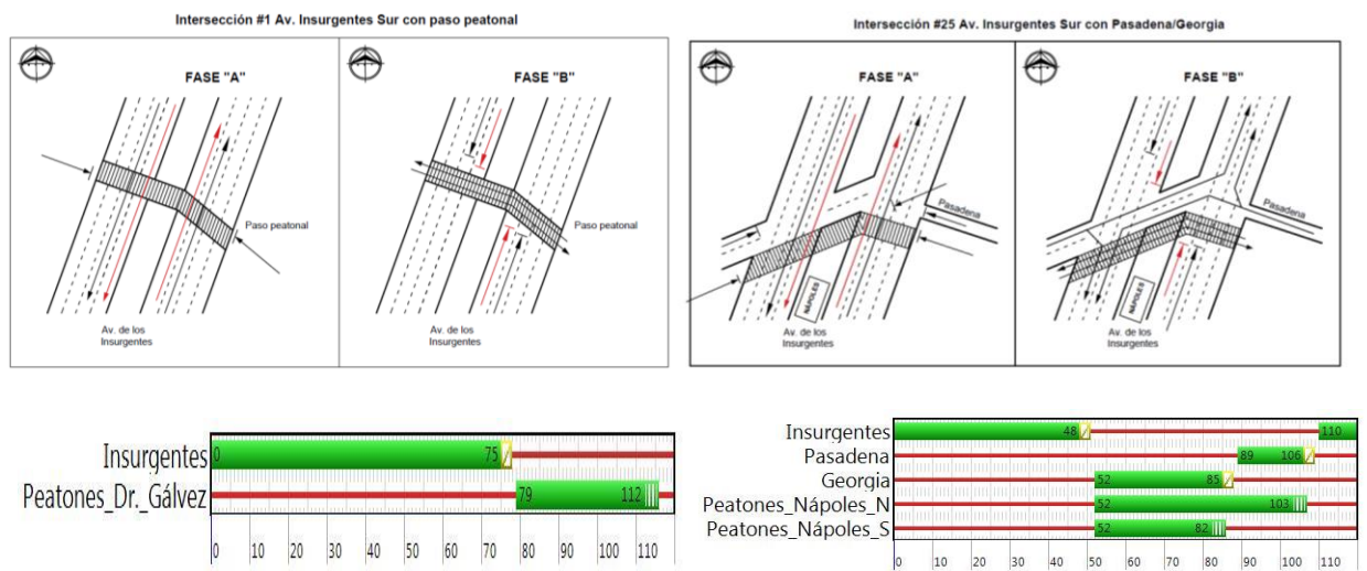
Figura 8.10: Tiempos y fases de 2 de las 44 intersecciones del tramo en estudio.
