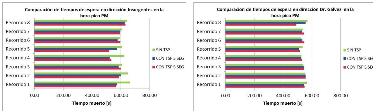
Figura 8.26: Comparación de tiempos de espera en ambas direcciones en la hora pico vespertina. Fuente: Elaboración propia.
