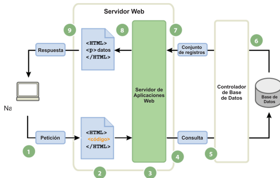
Figura 2.2: Componentes y funcionamiento de las aplicaciones web. Extraída y traducida de [1]
