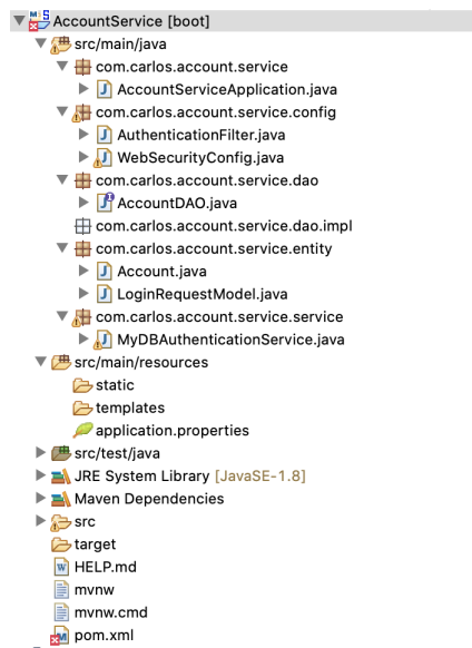
Figura 6.4: Estructura del nuevo proyecto Spring Boot conteniendo el subdominio account
