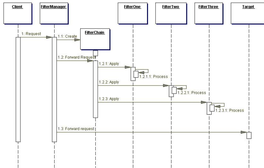
Figura 3.8: Diagrama de secuencia de Intercepting Filter. Extraído de [5]
