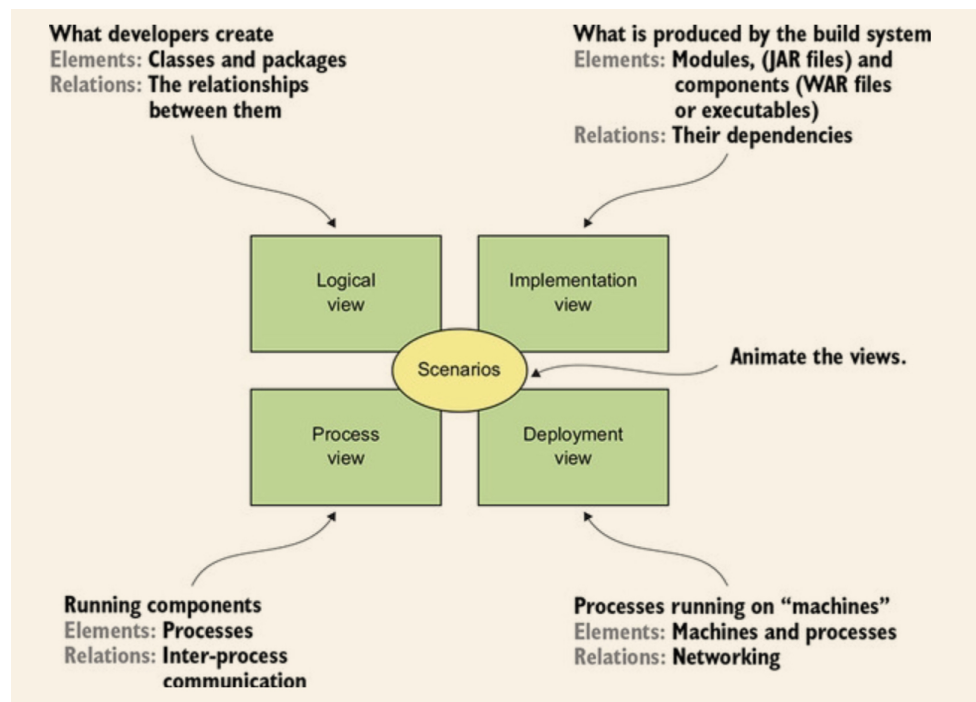
Figura 4.12: Modelo 4+1 de Arquitectura de Software. Extraído y traducido de [53]
