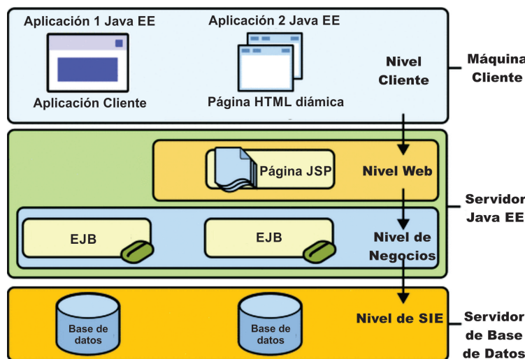
Figura 2.8: Arquitectura de Java EE. Extraída y traducida de [20]
