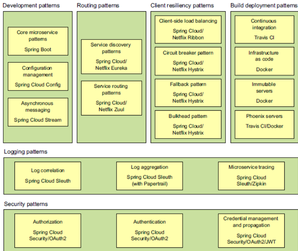
Figura 4.11: Patrones de diseño en Spring Cloud. Extraído de [71]
