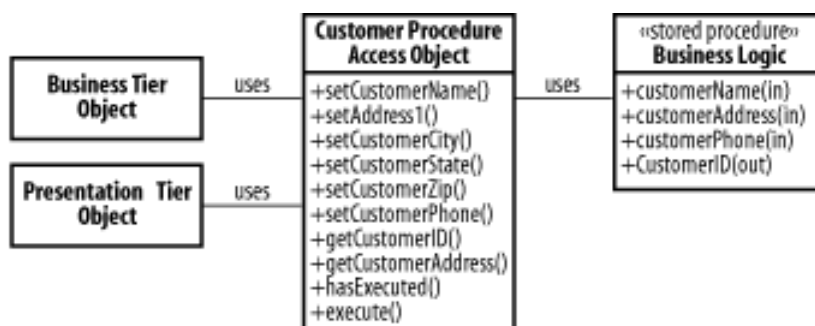
Figura 3.15: Diagrama de clases del Patrón Procedure Access Object. Extraído de [39]
