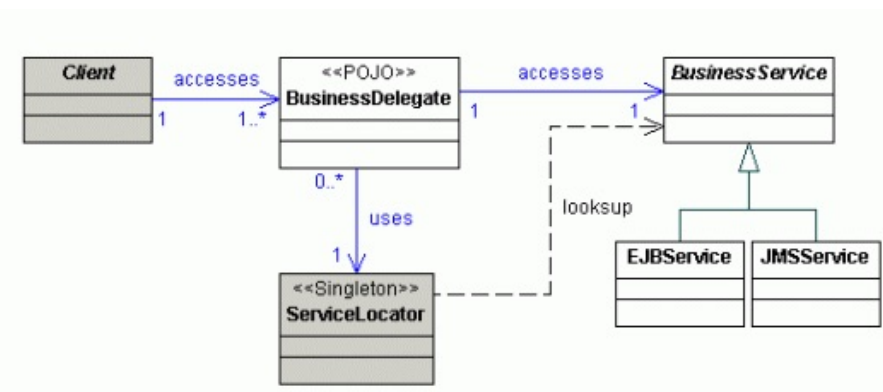
Figura 3.10: Diagrama de clases del Patrón Business Delegate. Extraído de [22]
