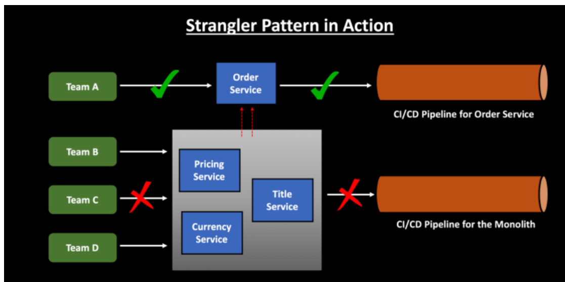
Figura 4.14: Patrón Strangler. Extraído de [36]
