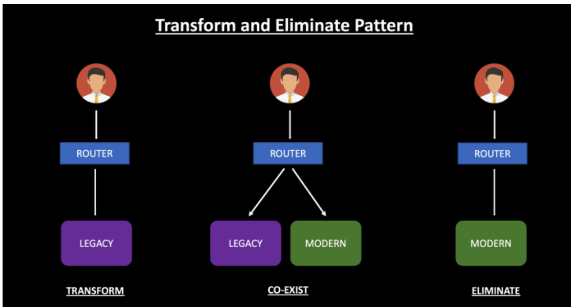
Figura 4.15: Implementación del patrón strangler. Extraído de [36]
