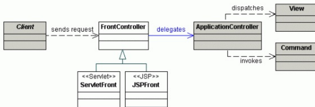
Figura 3.4: Estructura del Front Controller. Extraída de [50]
