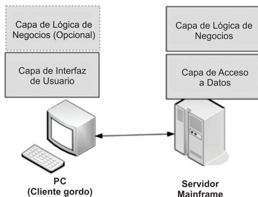
Figura 2.5: Arquitectura de dos niveles de tipo cliente pesado. Extraída y traducida de [50]
