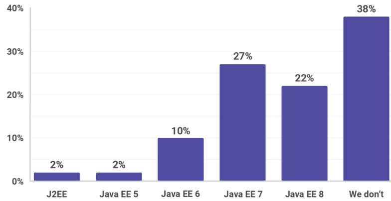
Figura 4.3: Versiones de Java EE utilizados en producción. Extraída de [56]
