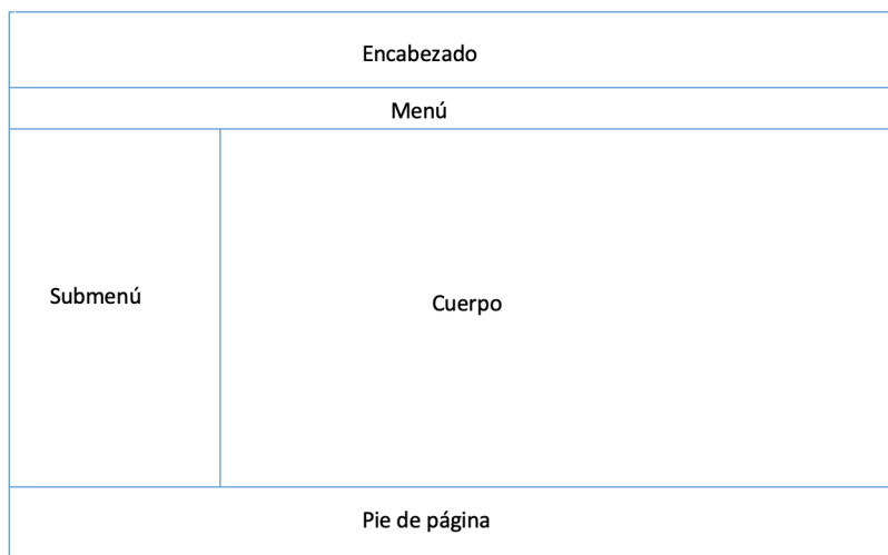
Figura 3.3: Patrón Composite View.
