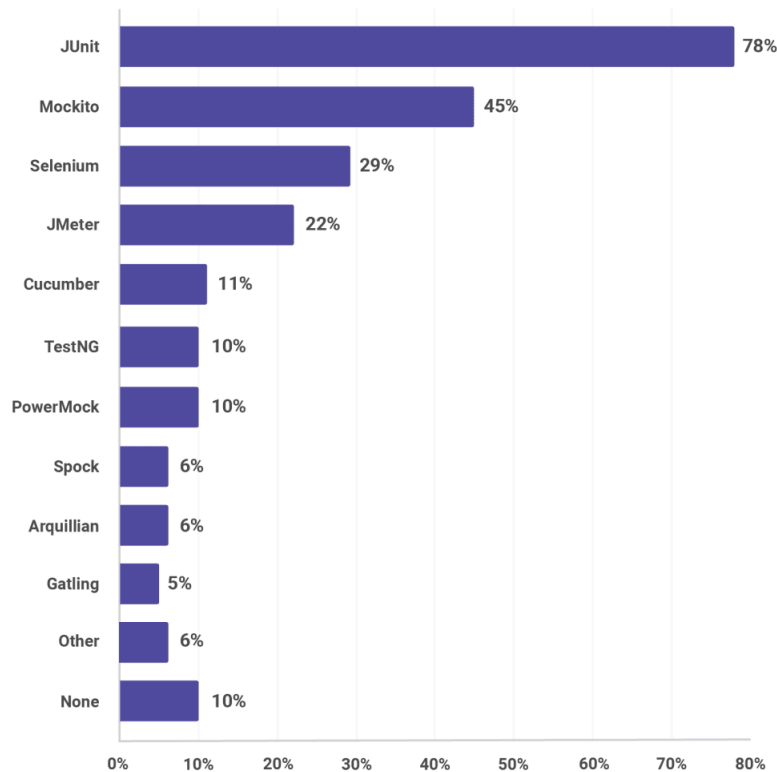
Figura 4.5: Herramientas de pruebas usadas. Extraída de [56]
