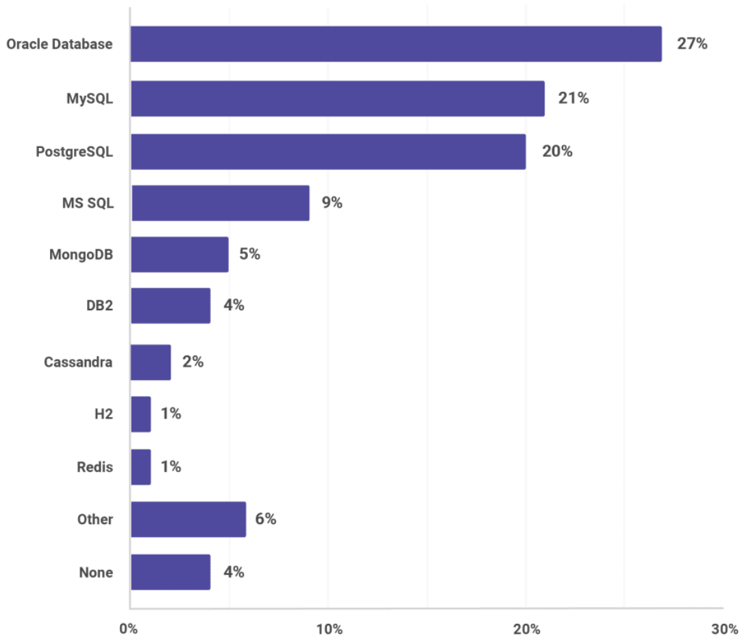
Figura 4.9: Bases de datos usadas. Extraída de [56]
