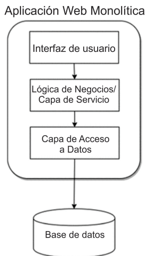
Figura 2.1: Aplicación web de arquitectura monolítica. Extraída y traducida de [48]
