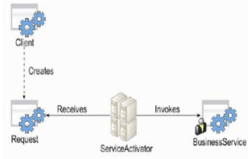
Figura 3.16: Patrón Service Activator. Extraído de [24]
