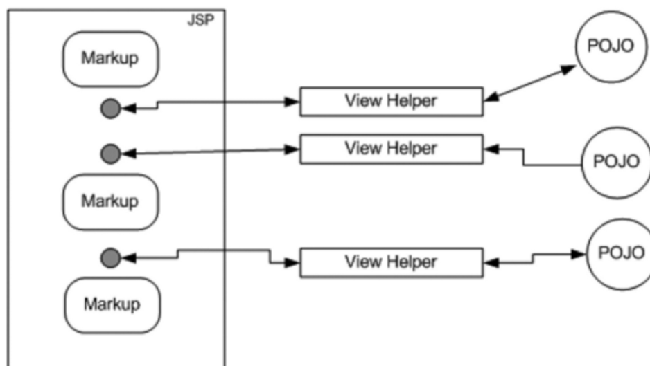
Figura 3.2: Patrón View Helper. Extraído de [50]
