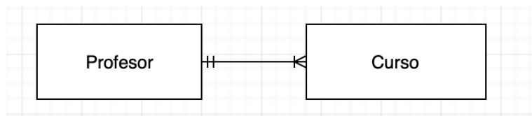
Figura 3.21: UML
