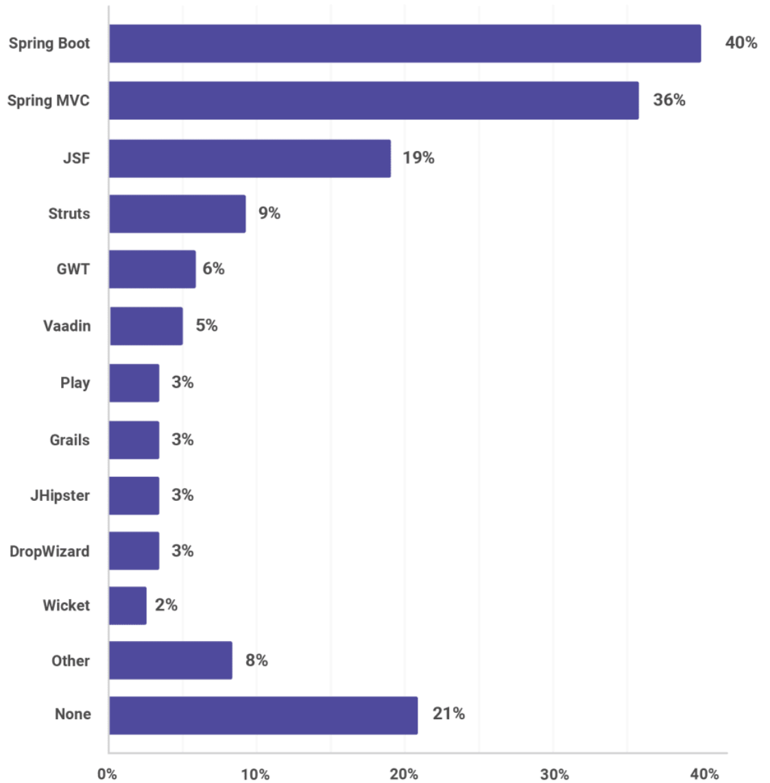
Figura 4.8: Frameworks web más usados. Extraída de [56]
