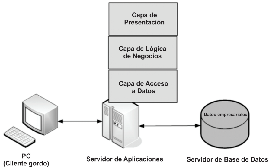
Figura 2.6: Arquitectura de tres niveles. Extraída y traducida de [50]
