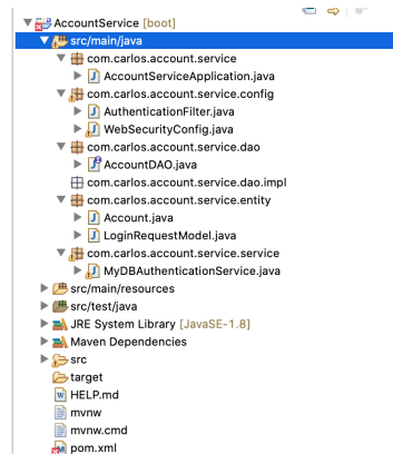
Figura B.1: Estructura del proyecto
