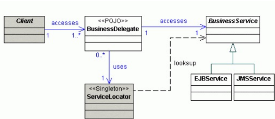
Figura 3.11: Diagrama de clases del Patrón Session Facade. Extraído de [25]
