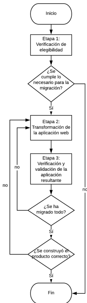
Figura 5.1: Diagrama de flujo general del método de migración.
