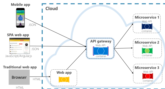
Figura 3.17: Patrón API Gateway. Extraído de [64]
