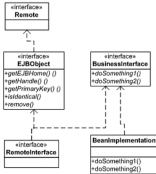
Figura 3.13: Diagrama de clases del Patrón Business Interface. Extraído de [50]
