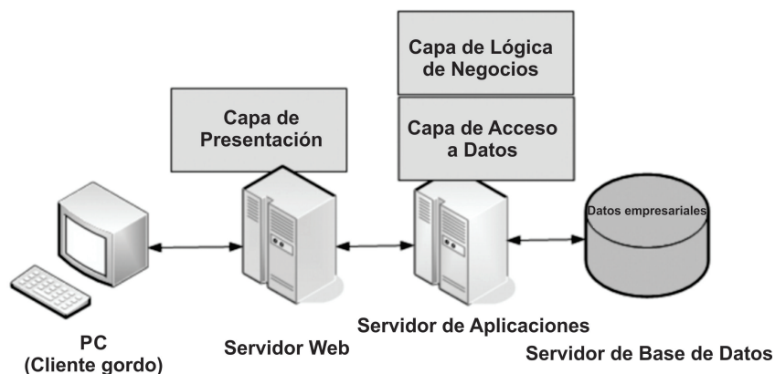
Figura 2.7: Aplicación de n niveles. Extraída y traducida de [50]
