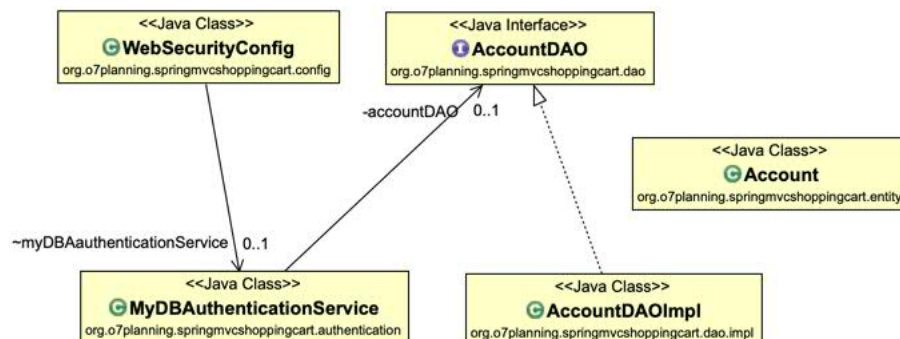
Figura 6.2: Parte del modelo Bounded Context diseñado correspondiente al subdominio account
