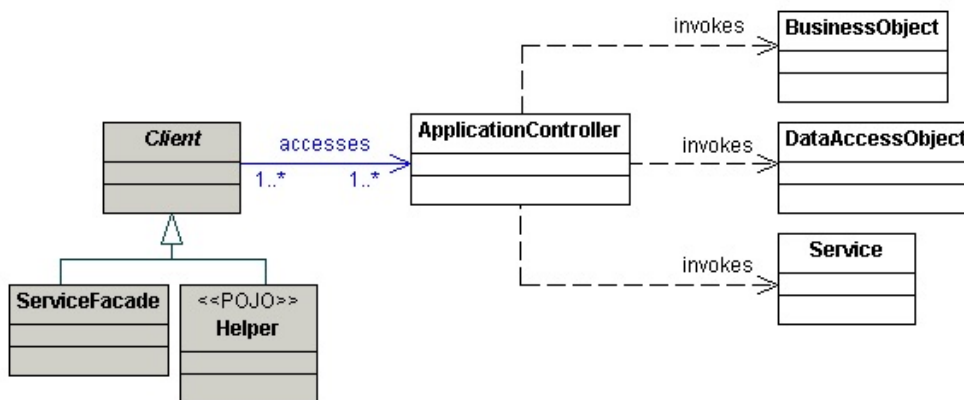
Figura 3.12: Diagrama de clases del Patrón Application Service. Extraído de [31]
