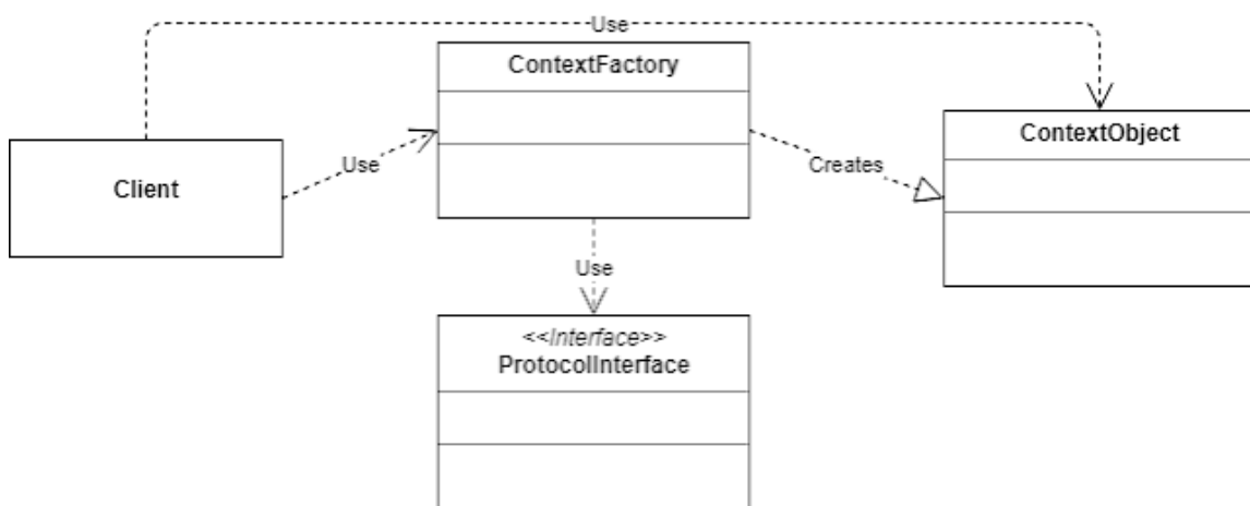
Figura 3.9: Diagrama de clases del Patrón Context Object. Extraído de [45]
