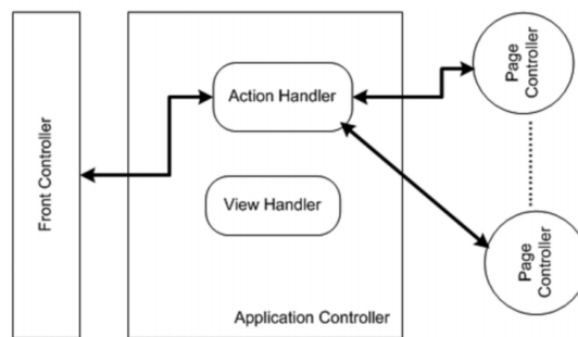
Figura 3.5: Flujo de trabajo del Action Handler. Extraído de [50]
