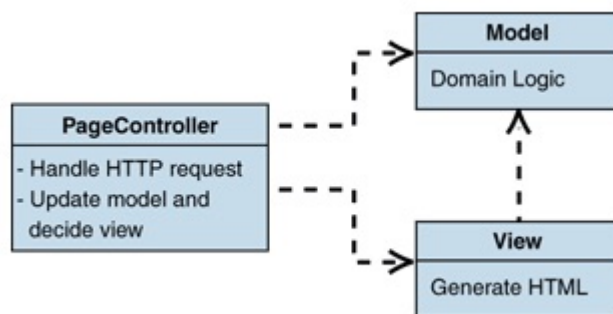
Figura 3.7: Estructura del Page Controller. Extraído de [32]
