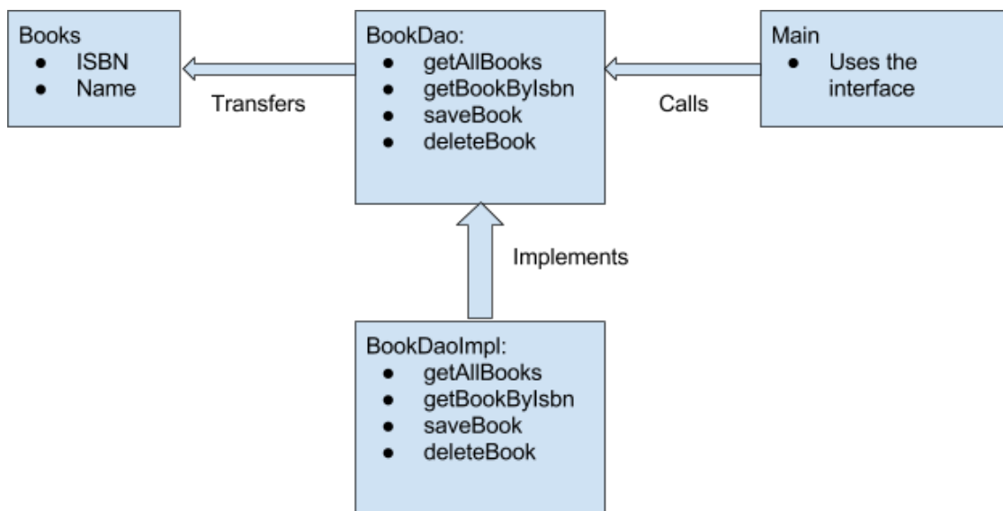
Figura 3.14: Ejemplo del Patrón DAO. Extraído de [57]
