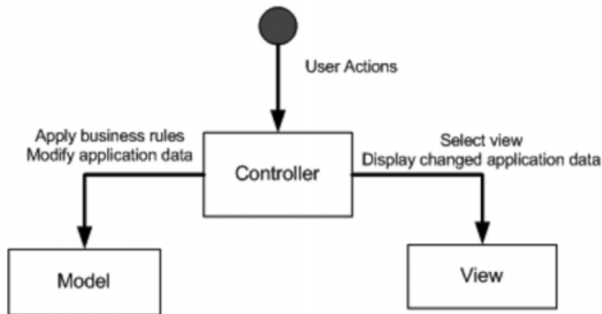
Figura 3.1: Modelo Vista Controlador. Extraído de [50]
