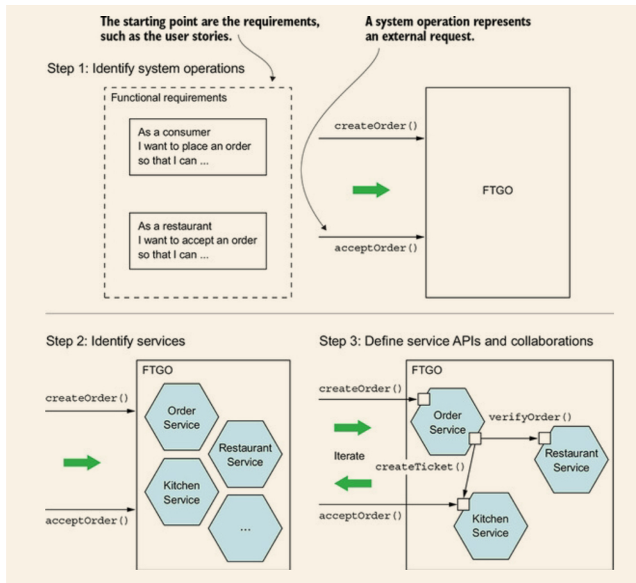
Figura 4.13: Pasos descritos para la identificación y definición de microservicios. Extraído de [63]
