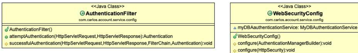
Figura B.3: UML de com.carlos.account.service.config
