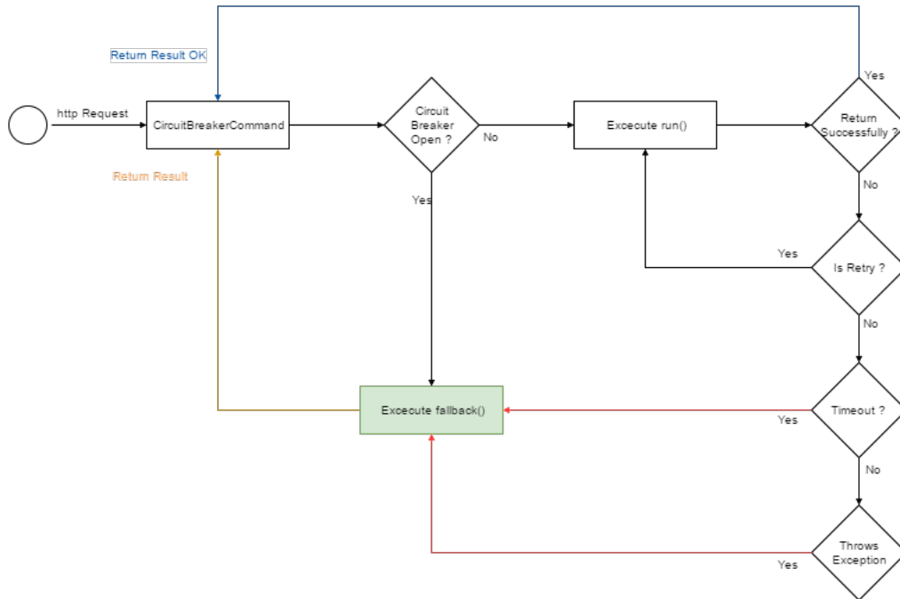
Figura 3.19: Interacción de Fallback con Circuit Breaker. Extraído de [51]
