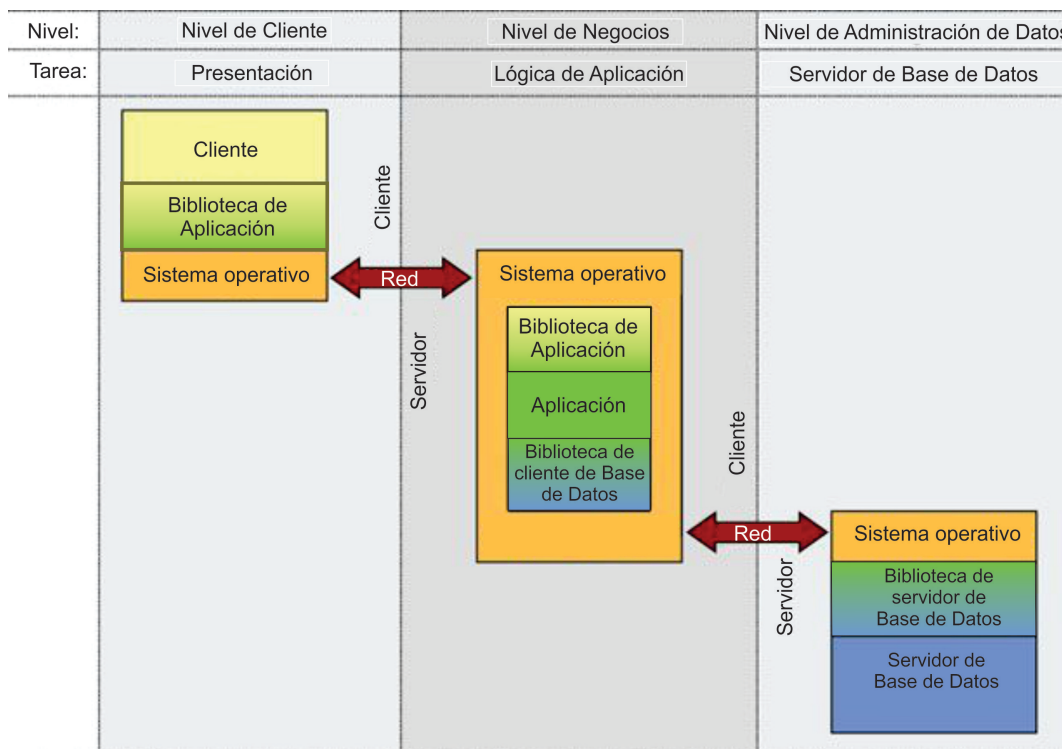
Figura 2.3: Arquitectura de 3-niveles. Extraída y traducida de [65]
