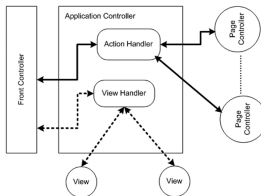
Figura 3.6: Flujo de trabajo del View Handler. Extraído de [50]
