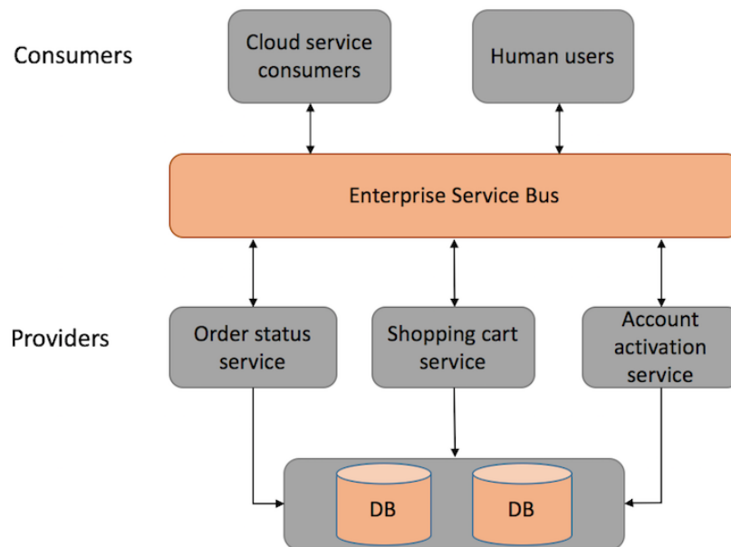
Figura 2.10: Arquitectura SOA. Extraído de [59]
