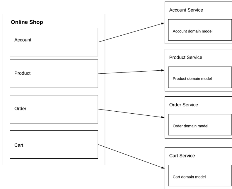
Figura 6.1: De subdominios a microservicios
