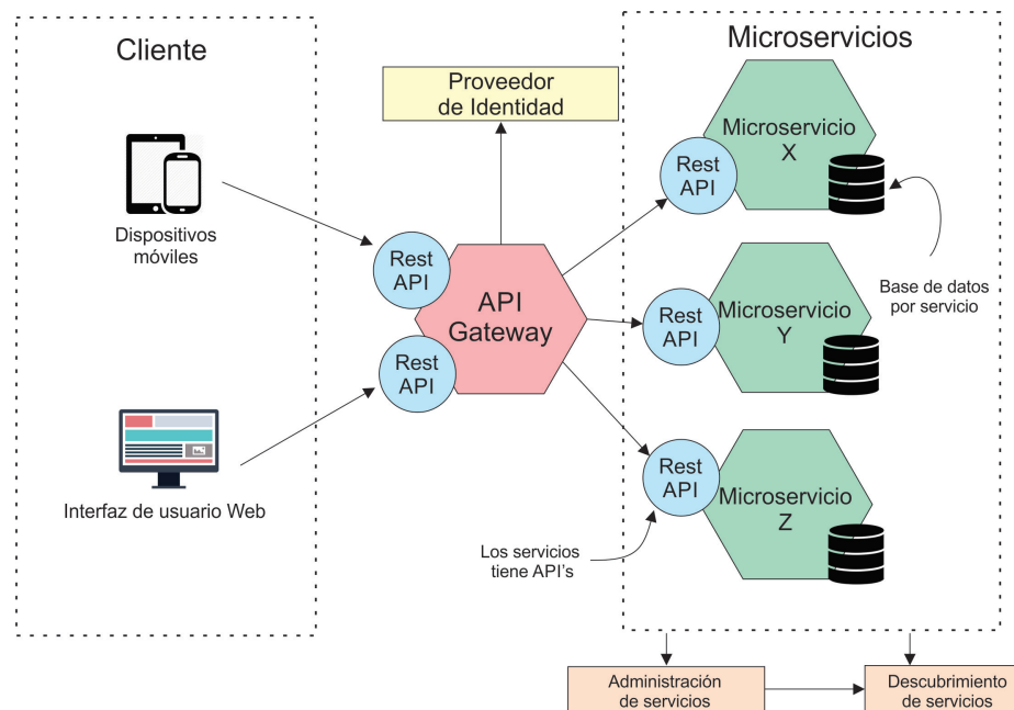
Figura 2.9: Arquitectura de los Microservicios. Basado en [49, 63]
