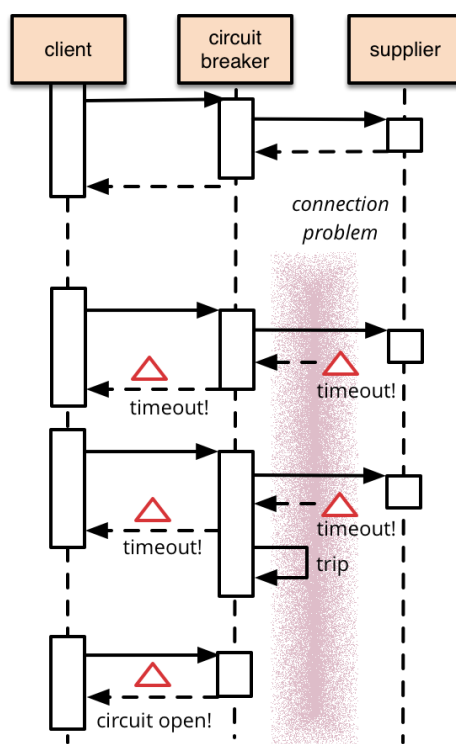
Figura 3.18: Diagrama de secuencias del Patrón Circuit Braker. Extraído de [2]
