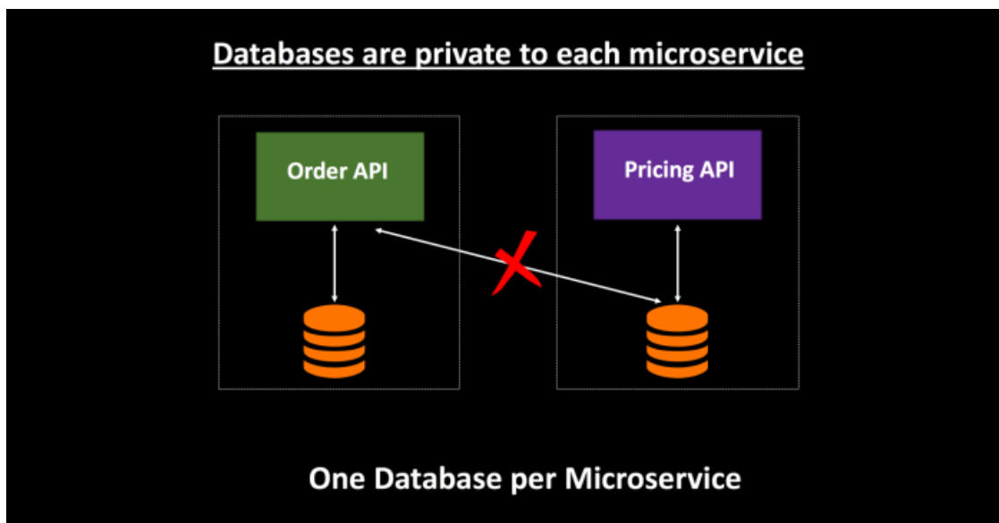
Figura 3.20: Database per service. Extraído de [37]
