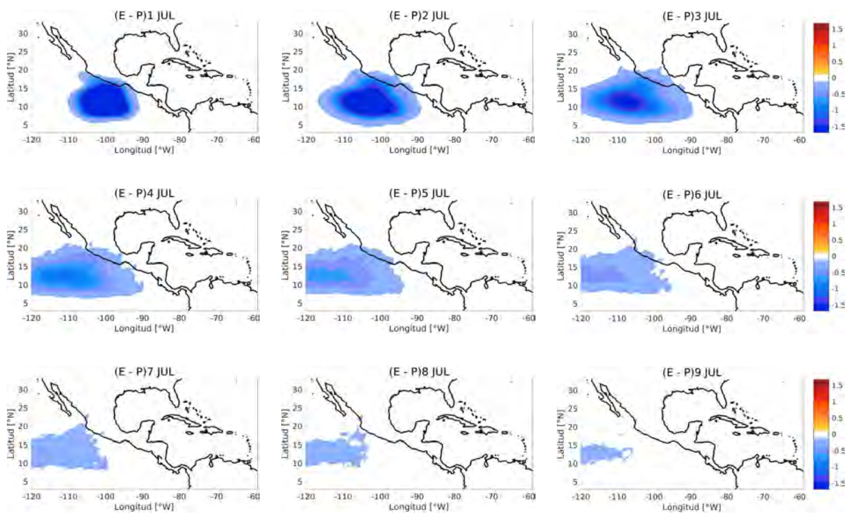
FIGURA 5.15: Climatologías mensuales de (E - P) ( \text{mm día}^{-1} ) del día 1 al día 9 desde que las partículas de aire abandonan la región evaporativa del NETP, para el mes de julio. Período: 1979-2017.
