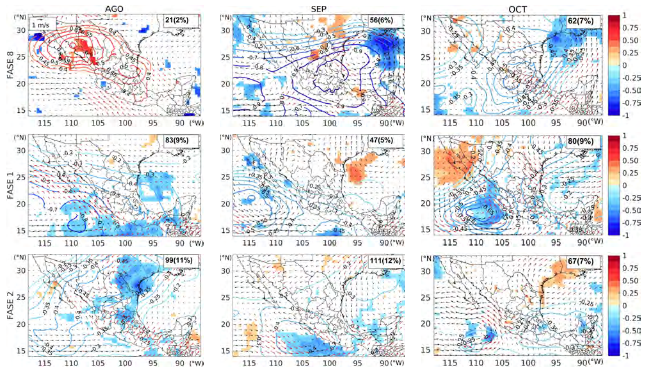
FIGURA 3.12: Compuestos de anomalías estandarizadas de la altura geopotencial en 500 hPa (contornos; anomalías negativas en azul), del viento en 850 hPa (los vectores rojos indican anomalías significativas a un nivel de confianza del 95 %) y de la velocidad vertical omega en 300 hPa (áreas sombreadas; anomalías negativas en azul indican movimientos ascendentes), para las fases húmedas de la MJO (8, 1, 2) de agosto a octubre (meses del MAX2). Solo se grafican las anomalías estadísticamente significativas a un nivel de confianza del 95 %. El número de días considerado en cada compuesto y sus porcentajes con respecto al total de días de cada mes en el periodo, se indican en la esquina superior derecha. Periodo: 1981–2010.
