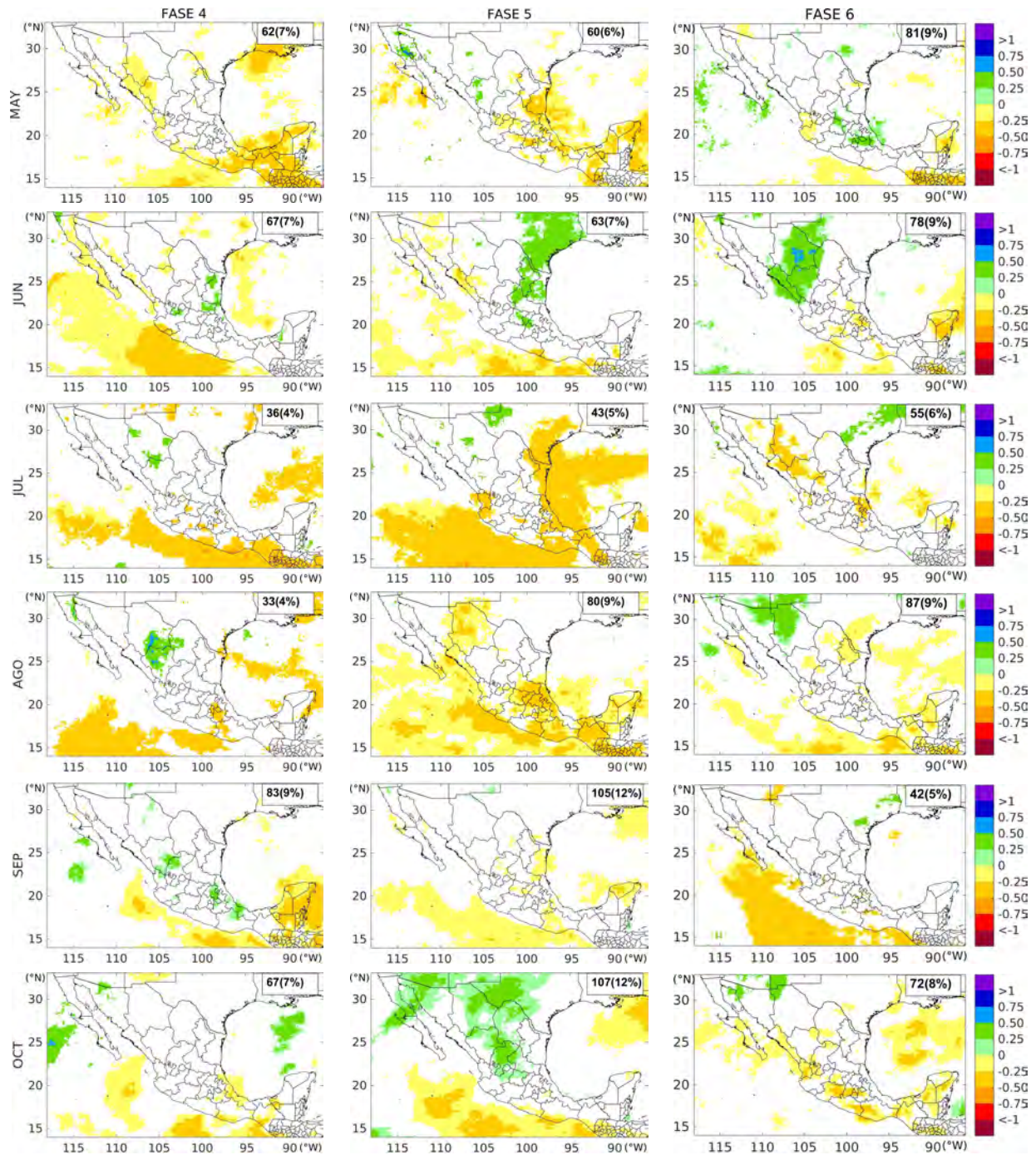
FIGURA 3.8: Compuestos de anomalías estandarizadas de precipitación para las fases secas de la MJO (4, 5, 6), para cada mes de la temporada de lluvias (de mayo a octubre). Solo se grafican las anomalías estadísticamente significativas a un nivel de confianza del 95%. El número de días considerado en cada compuesto y sus porcentajes con respecto al total de días de cada mes en el período, se indican en la esquina superior derecha. Período: 1981–2010.
