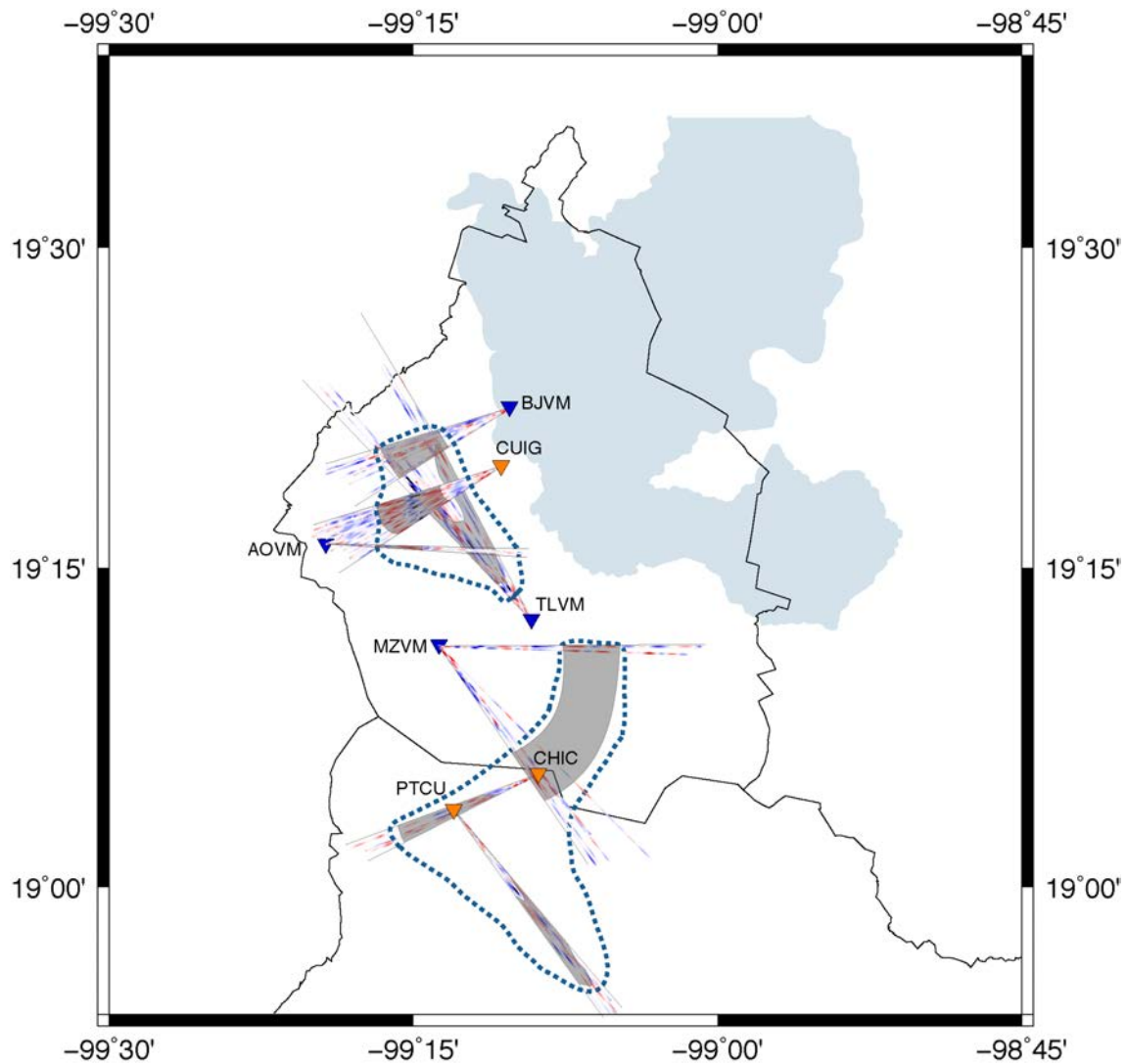
Figura 4.9 Proyección en superficie de los rayos que representan la trayectoria de los terremotos. En gris se sombreadon los pulsos correspondientes a las discontinuidades en la base de la corteza. Con líneas azules punteadas se propone la delimitación espacial de las discontinuidades observadas.
