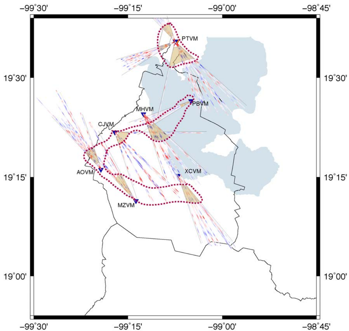
Figura 4.7 Proyección en superficie de los rayos que representan la trayectoria de los telesismos. Con café claro se sombrearon los pulsos correspondientes a las discontinuidades someras. Con líneas rojas punteadas se propone la delimitación espacial de las discontinuidades someras.
