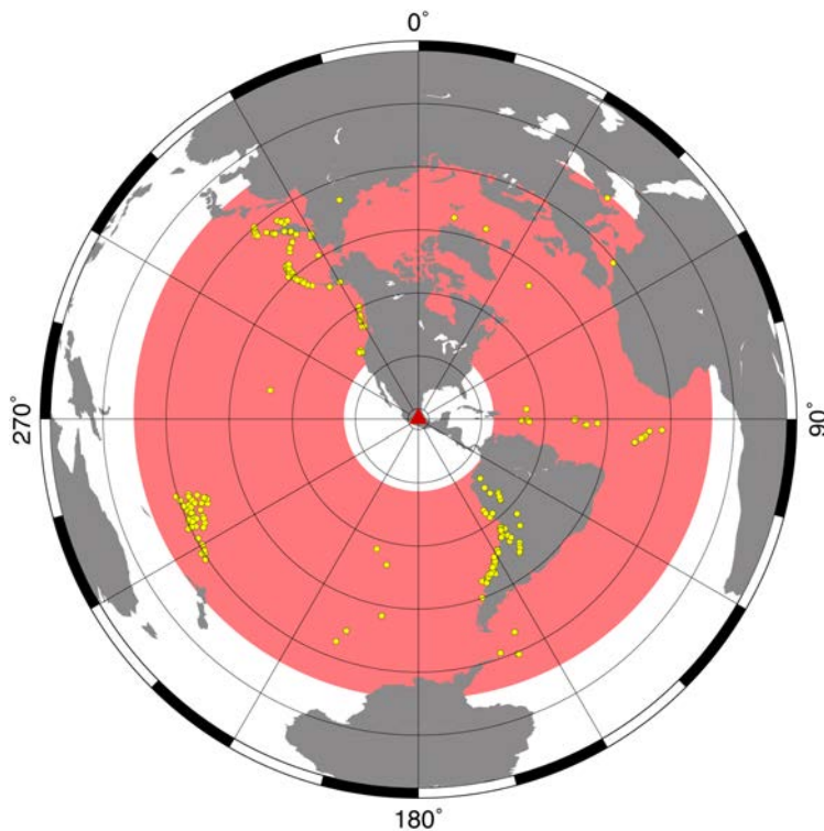
Figura 4.1 Epicentros de los telesismos usados para obtener funciones de receptor. Únicamente se utilizaron sismos a una distancia angular entre 30° y 90° de la estación.
