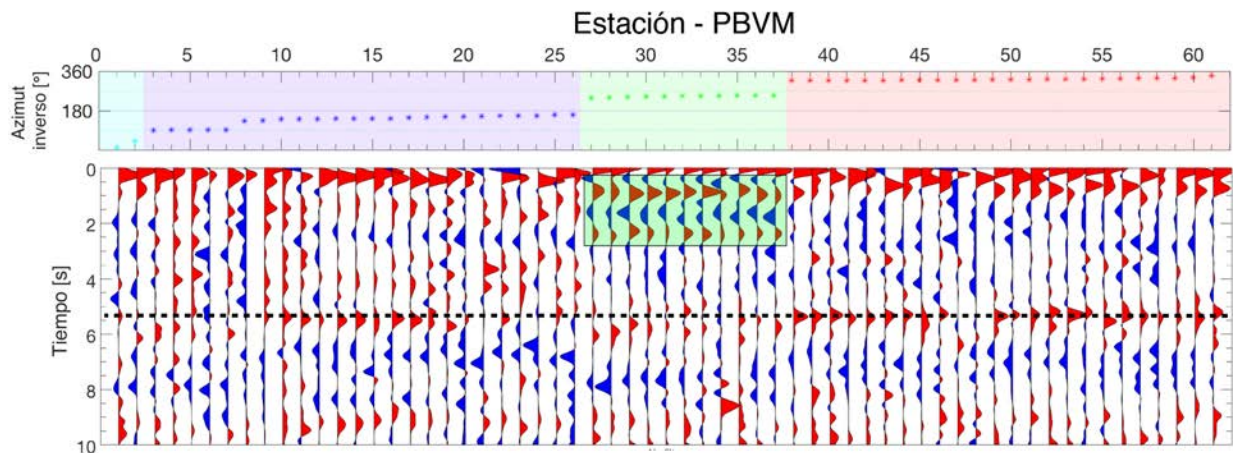
Figura 4.5 Funciones de receptor para la estación PBVM, ubicada en Peñón de los Baños, ordenadas por azimuth inverso. El panel superior muestra el valor de azimuth inverso correspondiente a cada traza y los colores representan los cuadrantes de azimuth inverso: turquesa: 0^{\circ} - 90^{\circ} ; azul fuerte: 90^{\circ} - 180^{\circ} ; verde: 180^{\circ} - 270^{\circ} ; rojo: 270^{\circ} - 360^{\circ} . Con una línea punteada se indican los pulsos correspondientes al Moho y en rectángulo sombreado se indican los pulsos exclusivos de ese azimuth.
