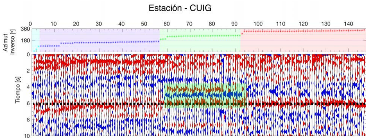
Figura 4.8 Funciones de receptor para la estación CUIG, ubicada en Ciudad Universitaria, ordenadas por azimut inverso. El panel superior muestra el valor de azimut inverso correspondiente a cada traza y los colores representan los cuadrantes de azimut inverso: turquesa: 0°-90°; azul fuerte: 90°-180°; verde: 180°-270°; rojo: 270°-360°. Con una línea punteada se indican los pulsos correspondientes al Moho y en rectángulo sombreado se indican los pulsos identificados en la base de la corteza, exclusivos de ese azimut.
