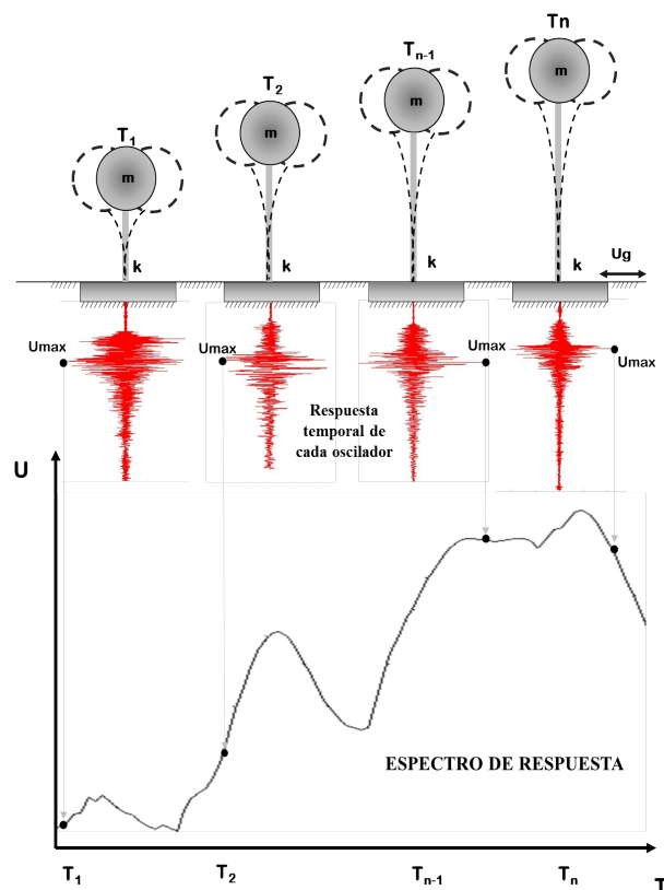
Figura 3.7: Construcción del espectro de respuesta.
