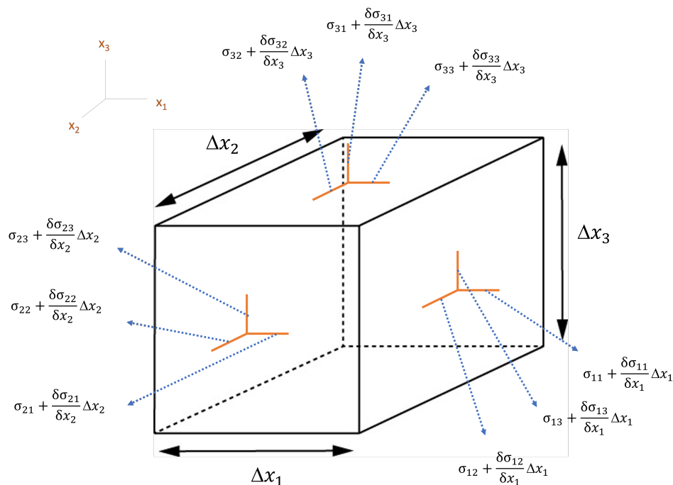
Figura 3.3: Estados de esfuerzos de un elemento \delta x . Modificado de Stein y Wysesession (2003).
