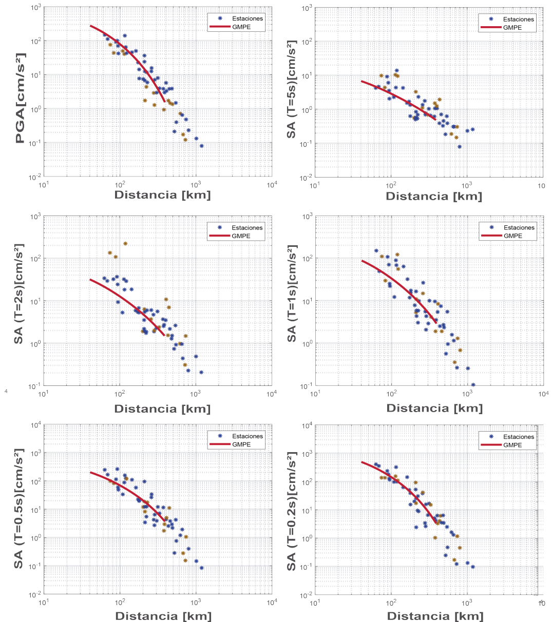
Figura 5.5: Comparación entre el espectro de respuesta de los datos y la estimación utilizando la ecuación de predicción de movimiento. Los asteriscos cafés representan las estaciones que se encuentran sobre la FVTM.
