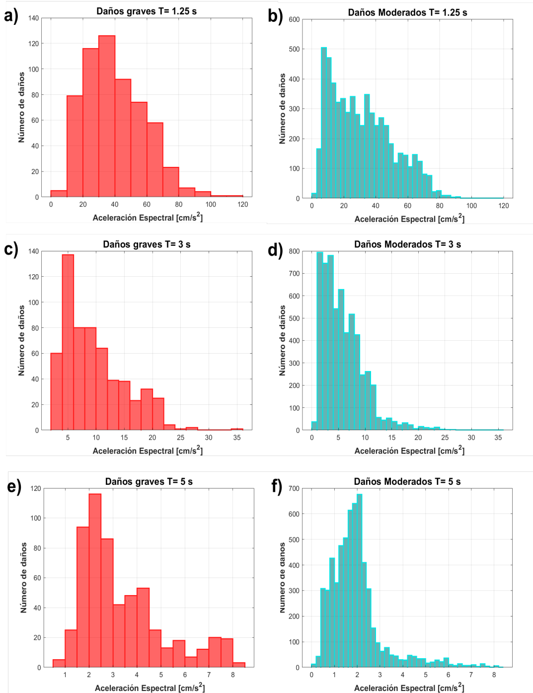
Figura 5.13: Pseudoaceleraciones espectrales para periodos de T = 1.25, 3 y 5 segundos asociadas con daños
