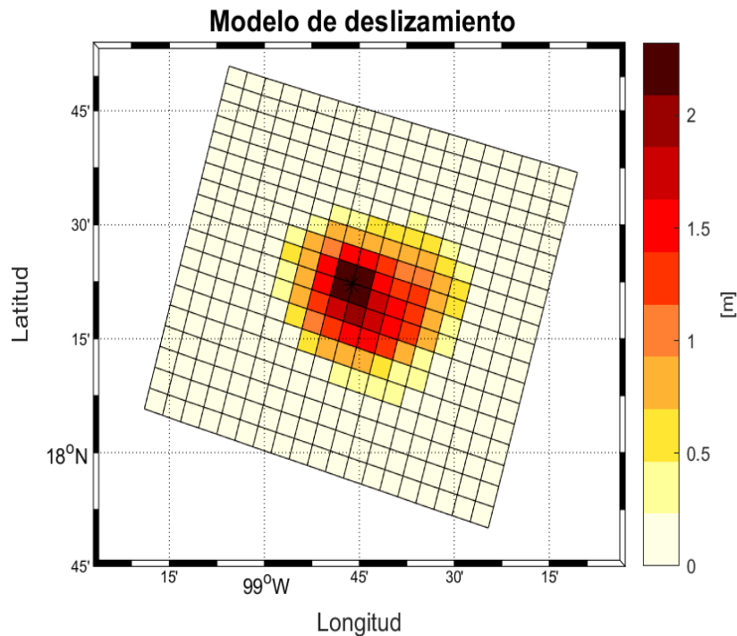
Figura 4.7: Modelo de deslizamiento en m.
