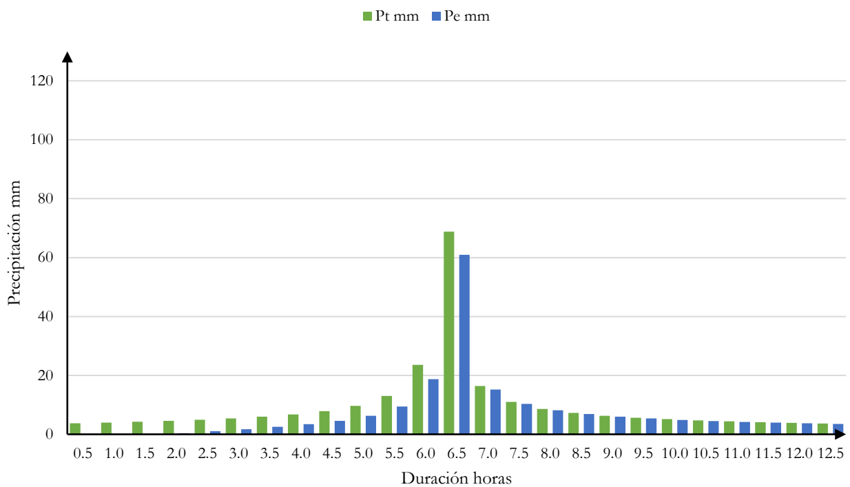
Ilustración 24. Hietograma de diseño de la estación Ayutla, para Tr=50 años.
