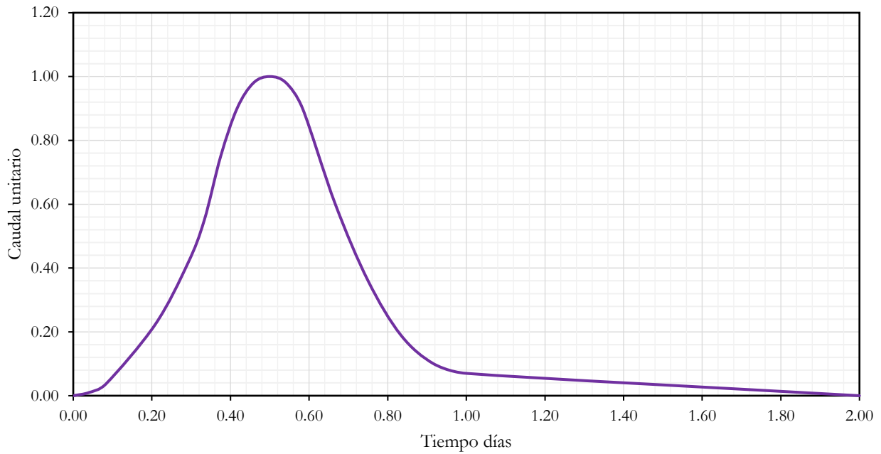
Ilustración 8. Hidrograma unitario para la estación 2018 Marquelia.
