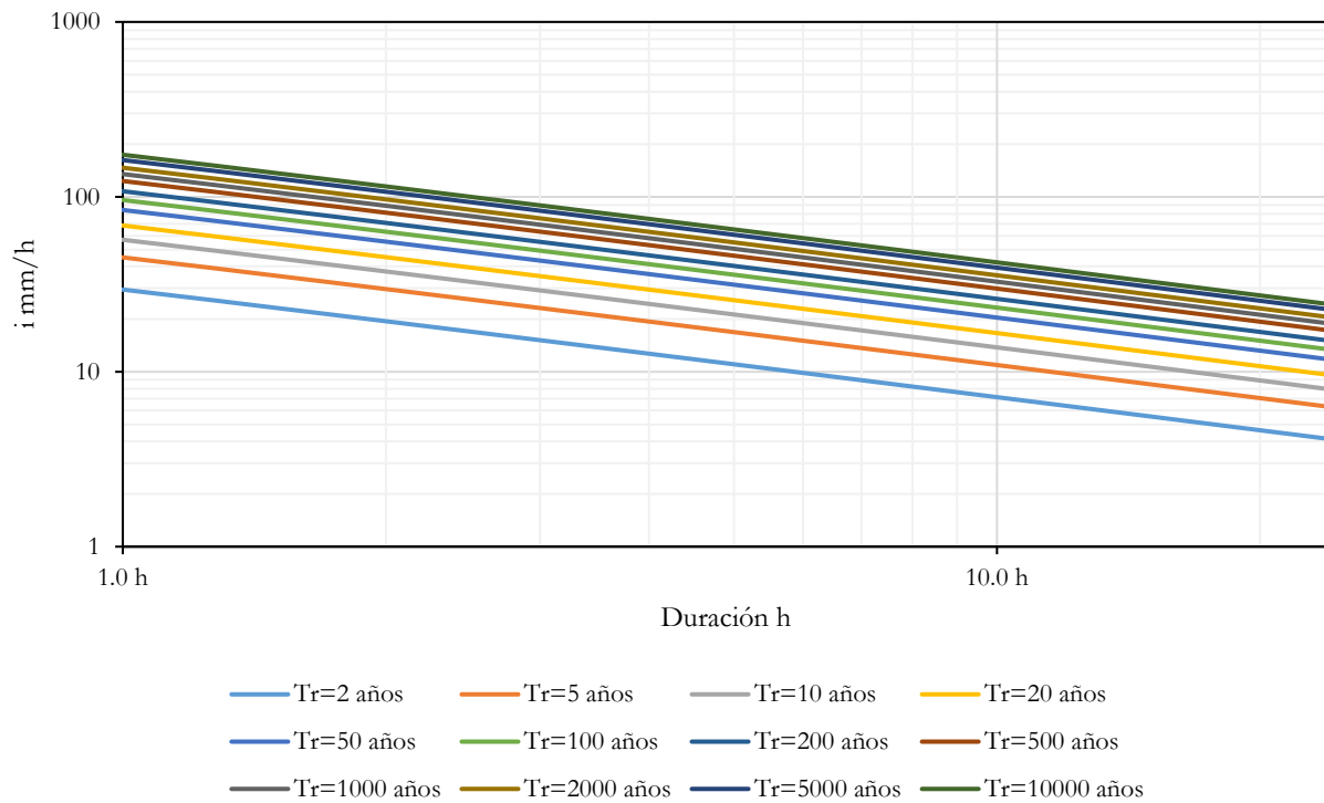
Ilustración 20. Curvas i-d-t para la estación 12068 San Luis Acatlán.
