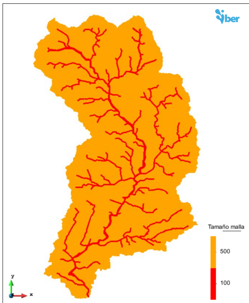
Ilustración 45. Tamaños de malla.
