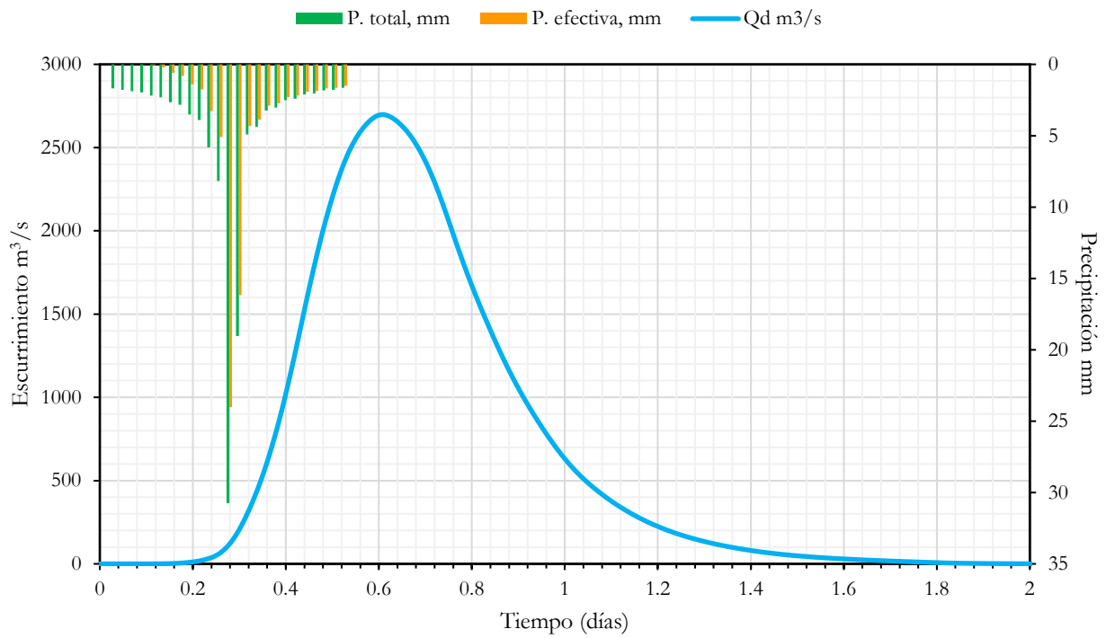
Ilustración 35. Hidrograma de escurrimiento directo, Tr= 20 años.
