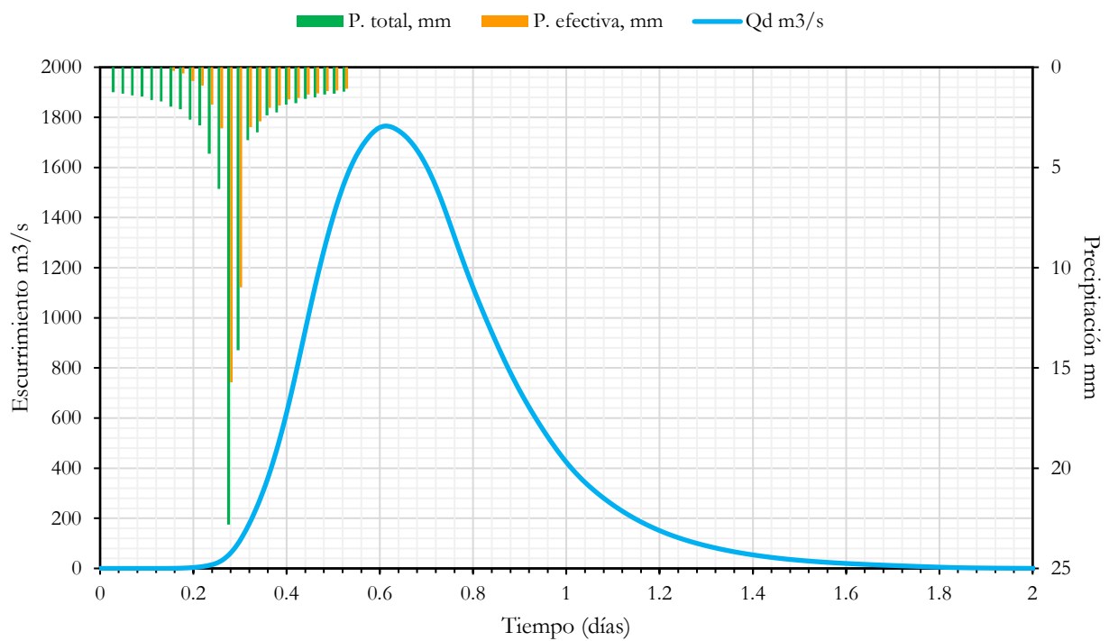
Ilustración 33. Hidrograma de escurrimiento directo, T_r=5 años.
