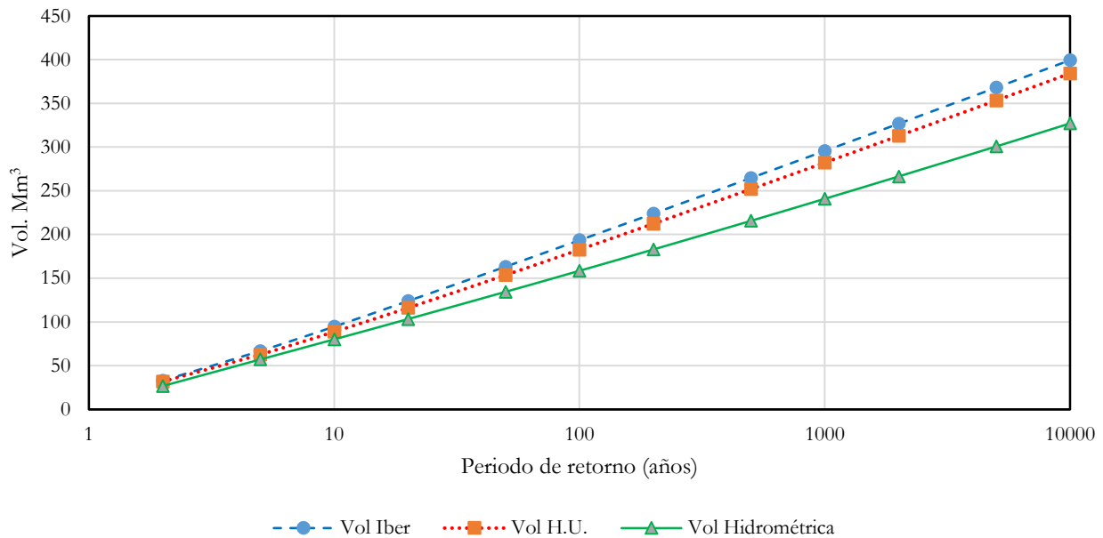
Ilustración 83. Comparación de volumen de escurrimiento directo, Cuenca del río Marquelia.
