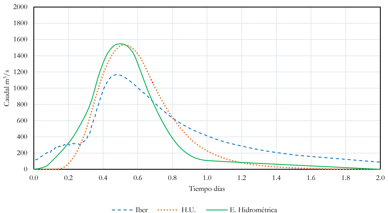
Ilustración 71. Comparación de hidrogramas, T_r=5 años.
