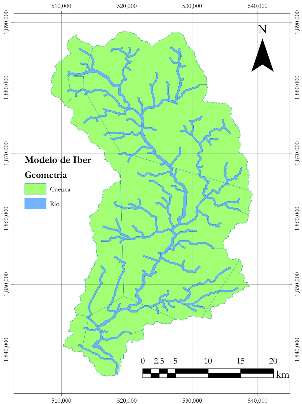
Ilustración 44. Geometría del modelo Iber: cauce principal, cauces secundarios y polígonos de Thiessen.
