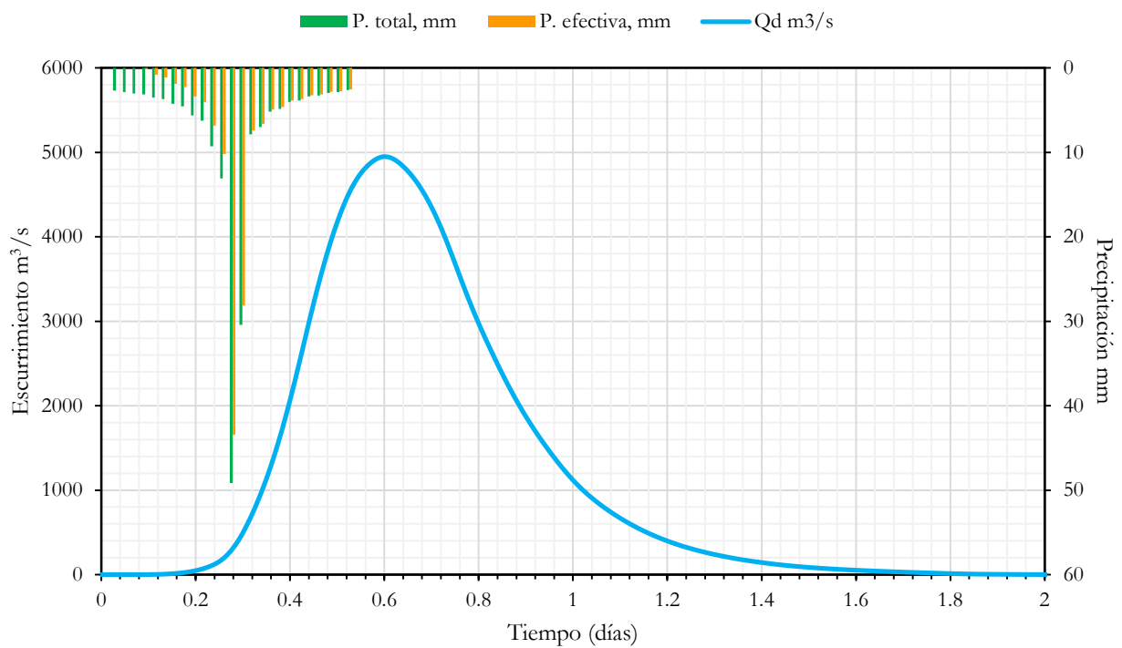
Ilustración 39. Hidrograma de escurrimiento directo, T_r = 500 años.
