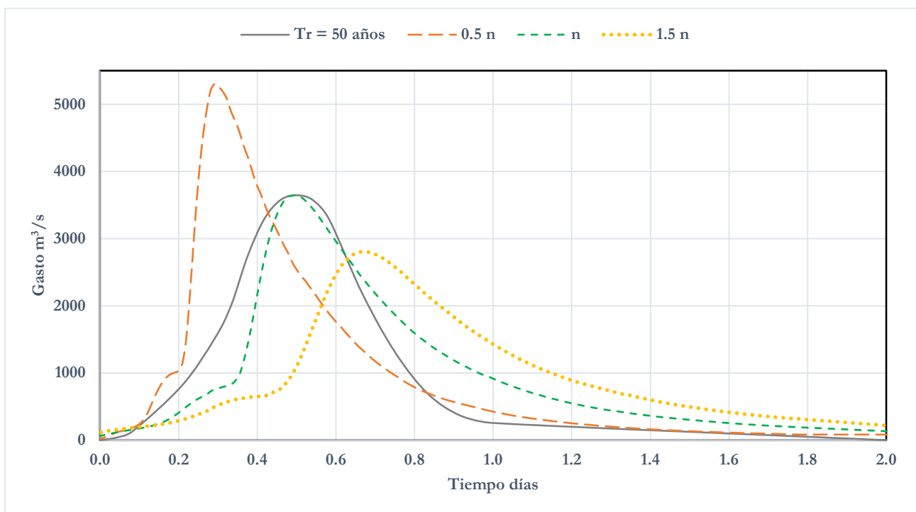
Ilustración 85. Hidrogramas para Tr= 50 años, calculados con diferentes coeficientes de rugosidad.
