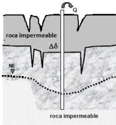
Figura 50. Mecanismo de subsidencia debido a la extracción de agua del subsuelo. Modificado de Manilla-Aceves et. al. , 2001.
