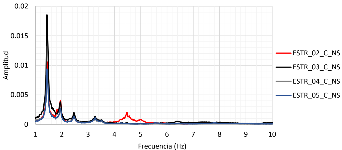
Figura 5.7 Valores promediados de FFT de las estaciones 2 al 5 en dirección norte-sur edificio C
