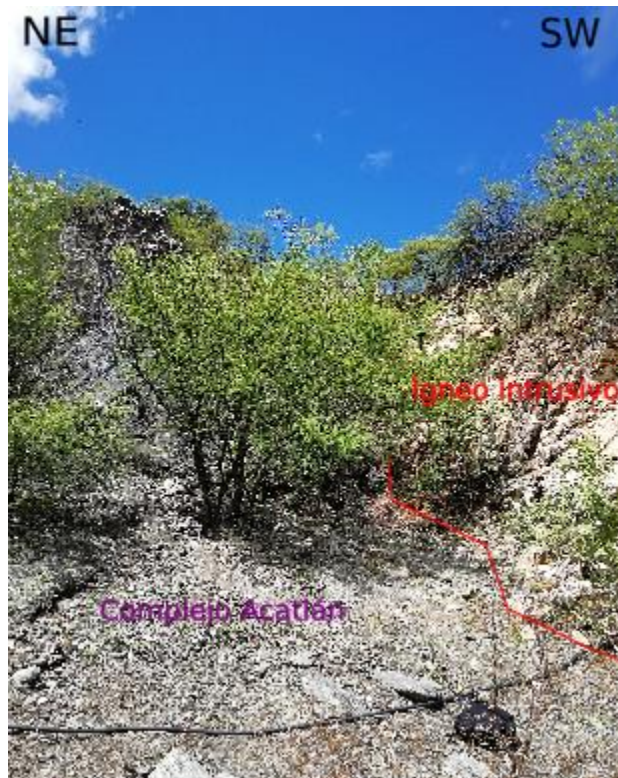
Ilustración V.3 Fotografía tomada en la barranca La Iguana con las coordenadas x= 628159 m, y= 2020781 m.
