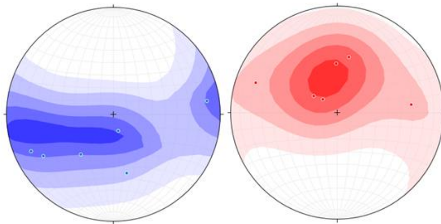
Ilustración IV.0.19 Concentraciones para el eje de acortamiento (a la izquierda) y para el eje de extensión (a la derecha).
