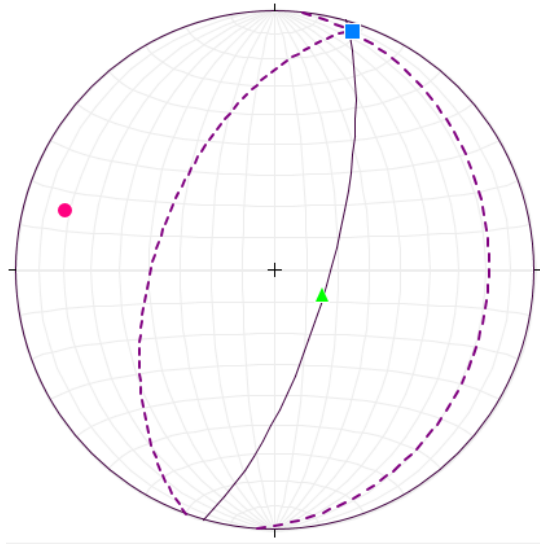
Ilustración IV.0.49 Proyección del pliegue y sus ejes de esfuerzo para el dominio I.
