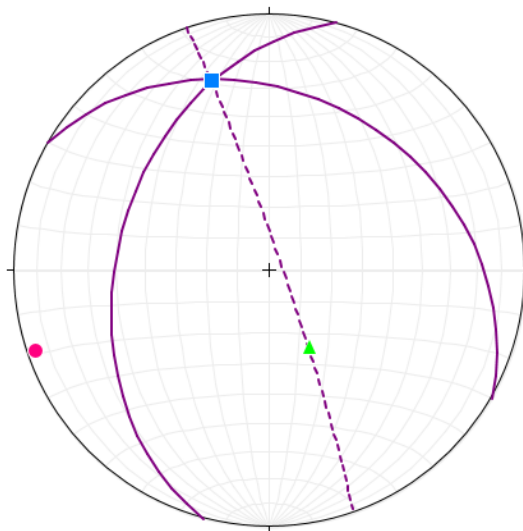
Ilustración IV.0.51 Proyecciones estereográficas para los esfuerzos pertenecientes al dominio III.
