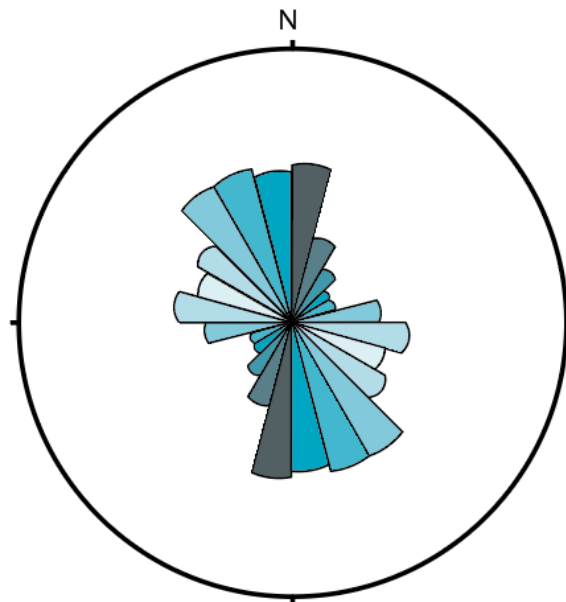
Ilustración IV.0.31 Roseta elaborada con datos de la formación Otlaltepec.
