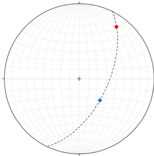
Ilustración IV.0.23 Proyección del eje de extensión (rojo) y el eje de acortamiento (azul).
