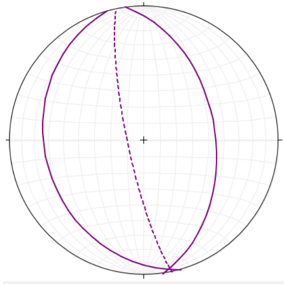
Ilustración IV.0.10 Proyección estereográfica del pliegue final obtenido del análisis hecho para los datos encontrados en el dominio IV. Marcadas por líneas continuas se representan los flancos, mientras que la línea punteada representa el plano axial del pliegue.
