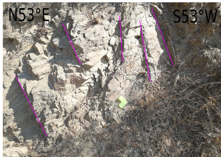
Ilustración IV.0.33 Foto del afloramiento en el que se obtuvieron los datos de fracturas en las afueras de Santo Tomás Otlaltepec. En rosa se encuentran marcadas algunas fracturas pertenecientes a la familia principal presente en la roseta.
