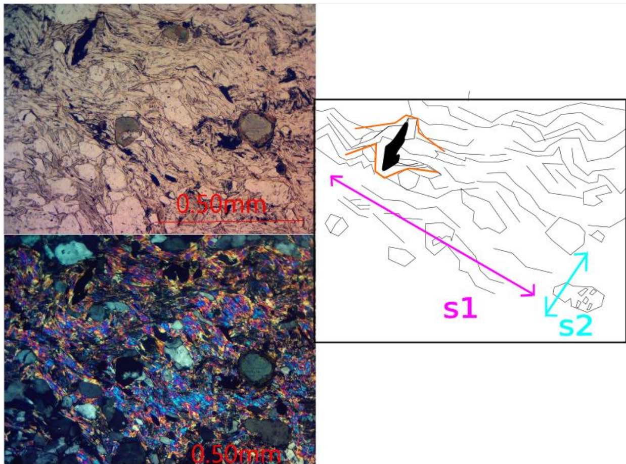
Ilustración IV.0.14 Del lado se encuentran fotografías de una sección en lámina delgada de la muestra M2, mientras que a lado derecho hay un diagrama del acomodo de las discontinuidades. En las fotos de la muestra se observa mica y fenocristales de cuarzo.
