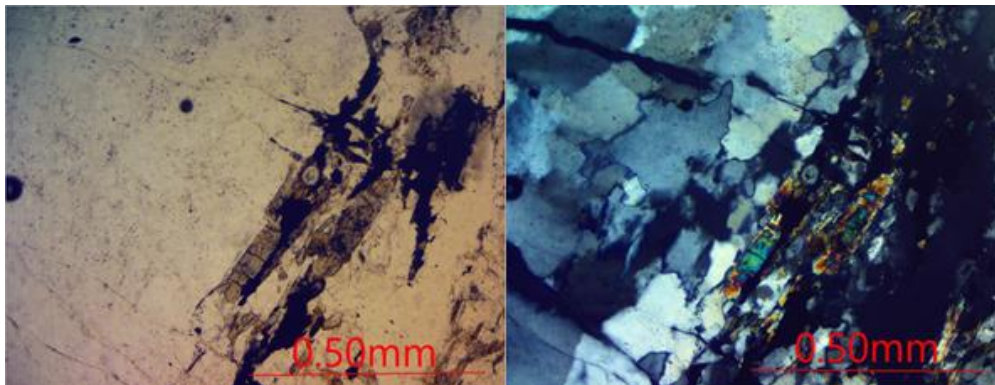
Ilustración III.2 Fotos (a la izquierda lp y a la derecha nx) tomada con el objetivo de 10x de la muestra F1 (tomada en la barranca La Iguana, en la zona de contacto entre el Complejo Acatlán y el Plutón Totoltepec), en la que se muestra un cristal de epidota y en el que se nota la deformación en fenoclastos de cuarzo a la izquierda.
