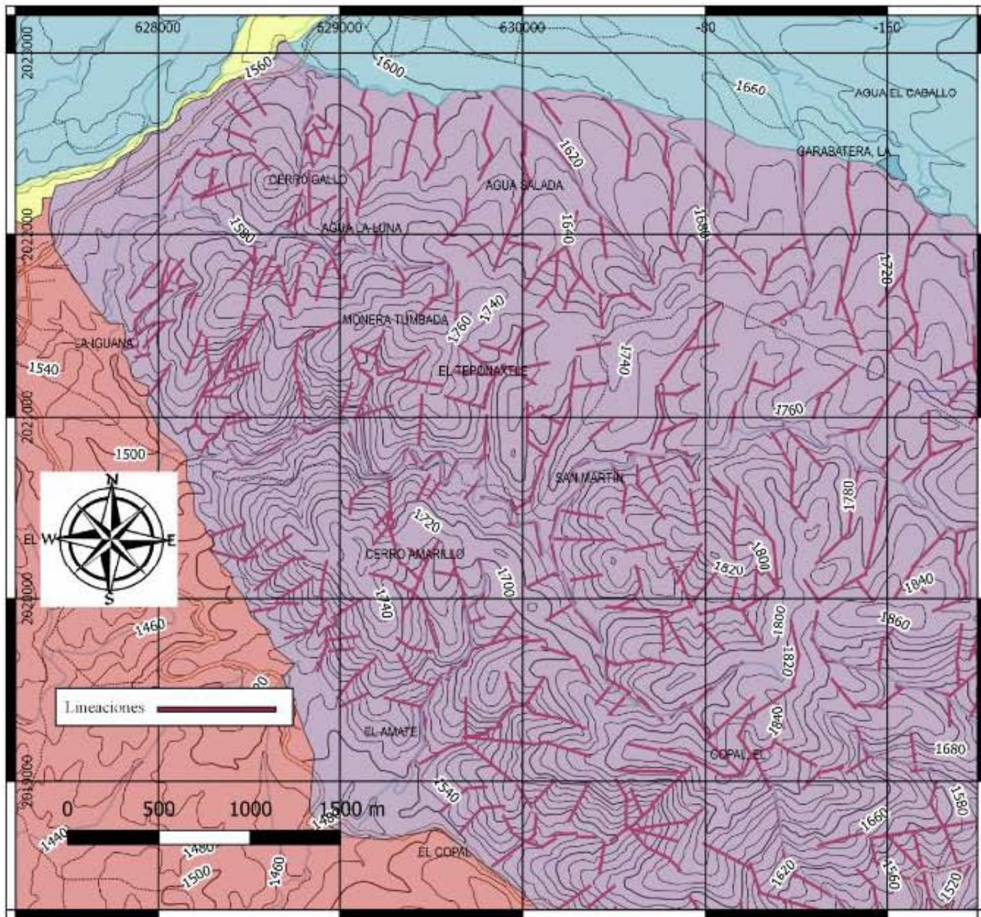
Ilustración VII.6 Mapa de la zona de estudio con las lineaciones marcadas en rosa.
