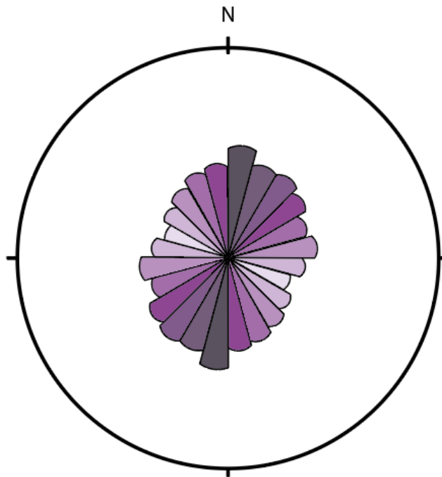
Ilustración IV.0.44 Roseta de lineaciones.
