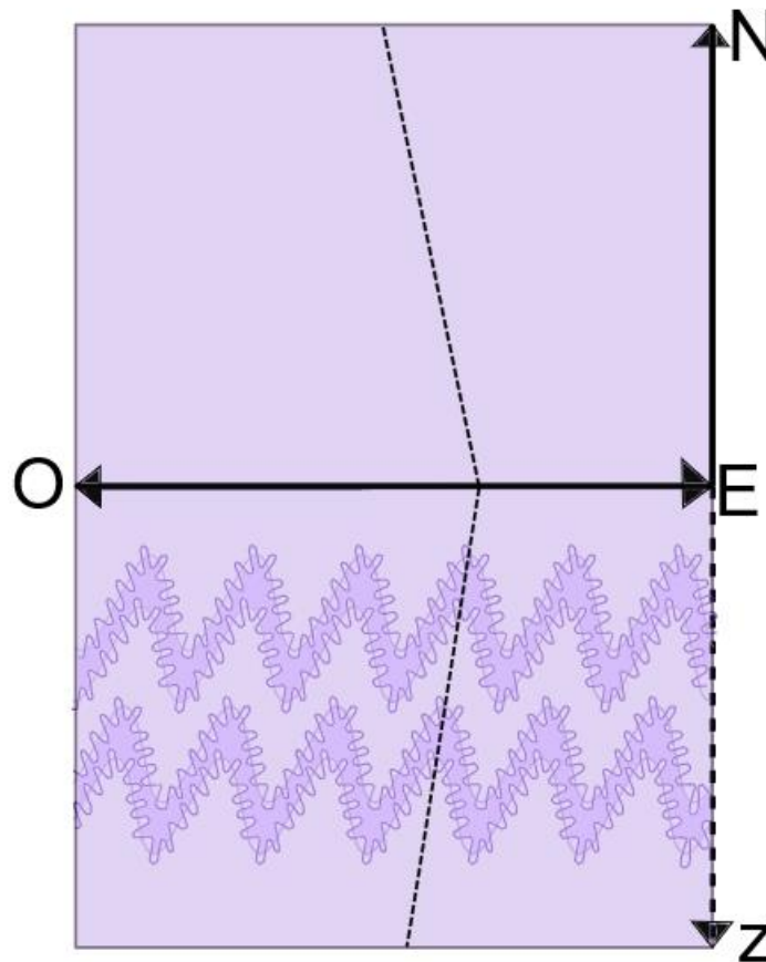
Ilustración VI.3 Forma y comportamiento del pliegue perteneciente al dominio IV.
