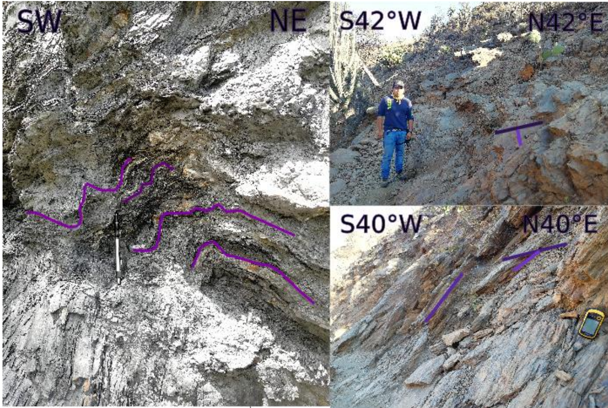
Ilustración IV.0.9 Fotos tomadas en la barranca La Iguana, la primera al E, cerca de la zona de contacto entre el esquistos y el granito, mientras que las siguientes dos fueron tomadas más al W, en los límites del cerro Teponaxtli.
