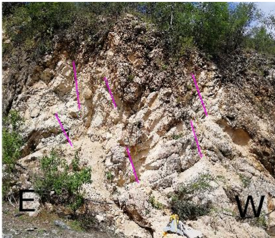
Ilustración IV.0.37 Fotografía del granito en la barranca La Iguana con algunas fracturas de la familia principal marcada en color rosa.
