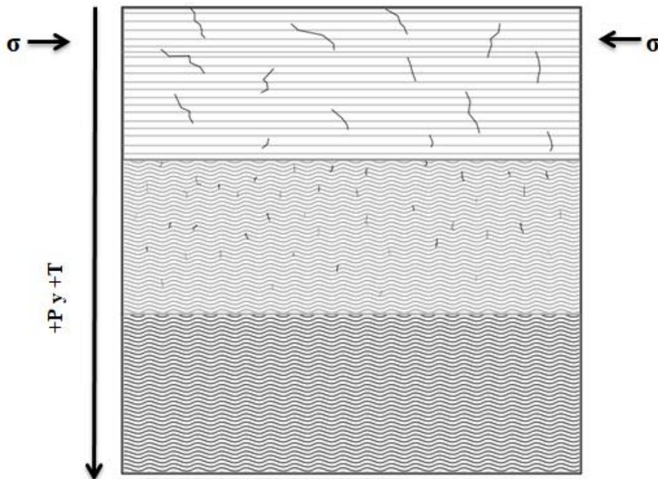
Ilustración VI.9 Comportamiento de un cuerpo de roca al presentarse P y T, además de un esfuerzo de contracción.
