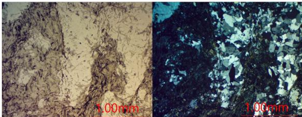
Ilustración III.3 Fotos (a la izquierda lp y a la derecha nx) tomadas con el objetivo de 4x de la muestra M1 (tomada en la barranca La Iguana, en los límites entre el cerro Teponaxtli y cerro Amarillo), en la que se observa la presencia de clorita que es muy abundante en esta muestra.
