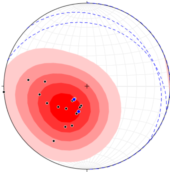
Ilustración VII.4 Concentración de los polos de los datos en la tabla VII.7. En azul se encuentran los polos utilizados para obtener los flancos utilizados para el análisis.
