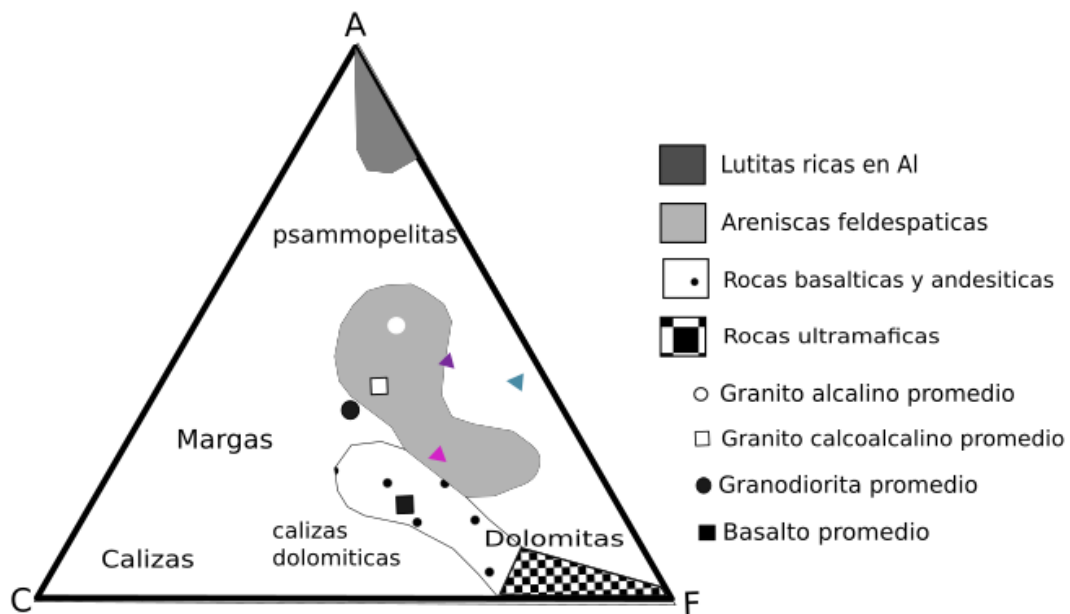
Ilustración III.4 Diagrama ACF (Winkler 1979) en el que se grafican las muestras M1 (color azul), M3 (color morado) y M3 (color rosa).
