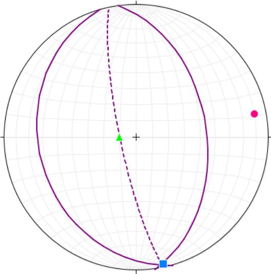
Ilustración IV.0.52 Proyecciones estereográficas de los esfuerzos que pertenecen al dominio IV.
