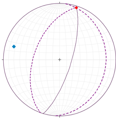
Ilustración IV.0.27 Proyección del pliegue del Dominio I con su dominio de extensión en rojo y eje de acortamiento en azul.
