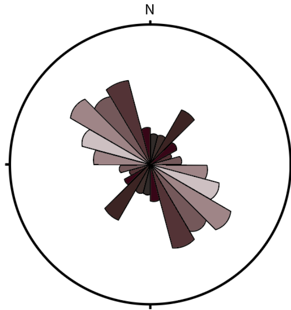
Ilustración IV.0.38 Roseta de fracturas obtenida de datos en la barranca La Iguana en el Complejo Acatlán.
