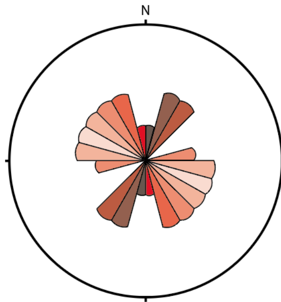
Ilustración IV.0.40 Roseta obtenida por datos en el Plutón Totoltepec (contacto entre gabro y granito).
