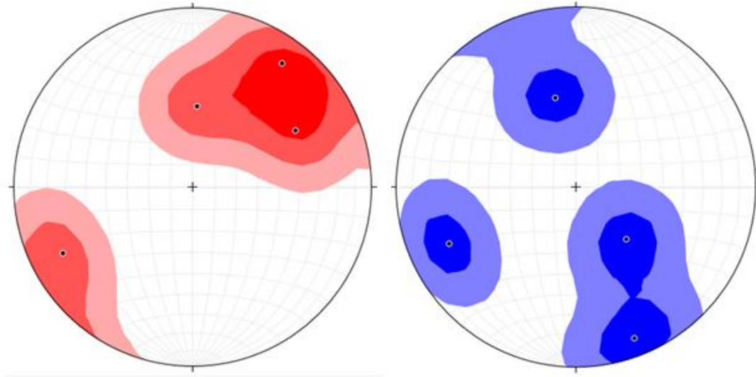
Ilustración VI.6 Conteo de puntos para los ejes de extensión y de acortamiento obtenido en las fallas. A la izquierda, en rojo, se encuentran los ejes de extensión y a la derecha, los de acortamiento.
