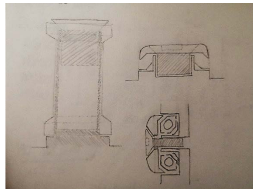
Figura 3.20.- Tornillería
