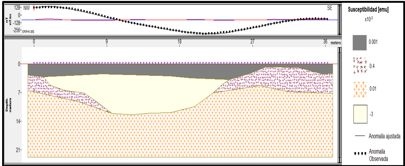
Figura 23. Modelo A bidimensional de la anomalía observada para el perfil A.
