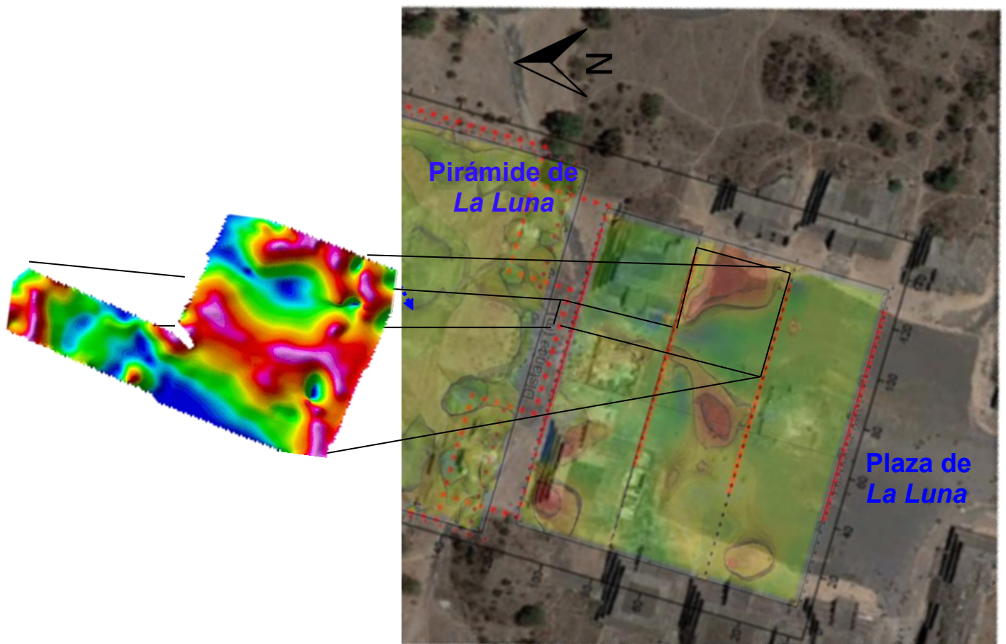
Figura 36. Localización de las estructuras en la Plaza de la Luna de acuerdo al estudio de TRE-3D y magnetometría (Modificada de Chávez et. al, 2018).
