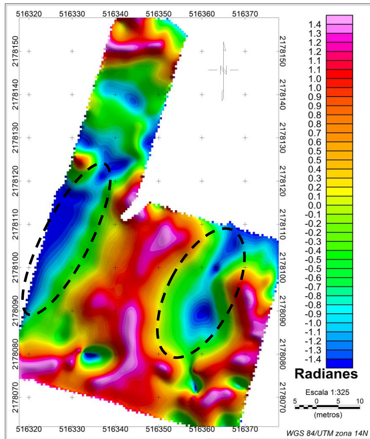
Figura 22. Tilt derivative de la PL del Campo Anómalo Total reducido al polo del levantamiento magnético en la PL.
