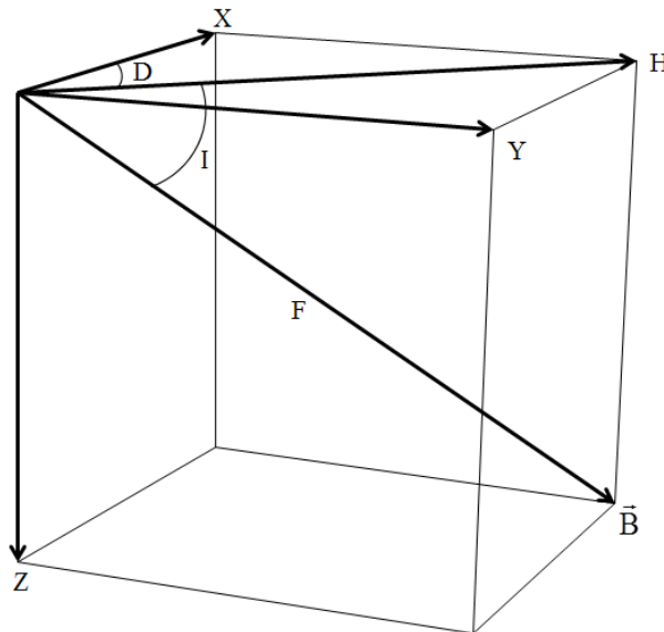
Figura 6. Representación del vector del campo magnético.
