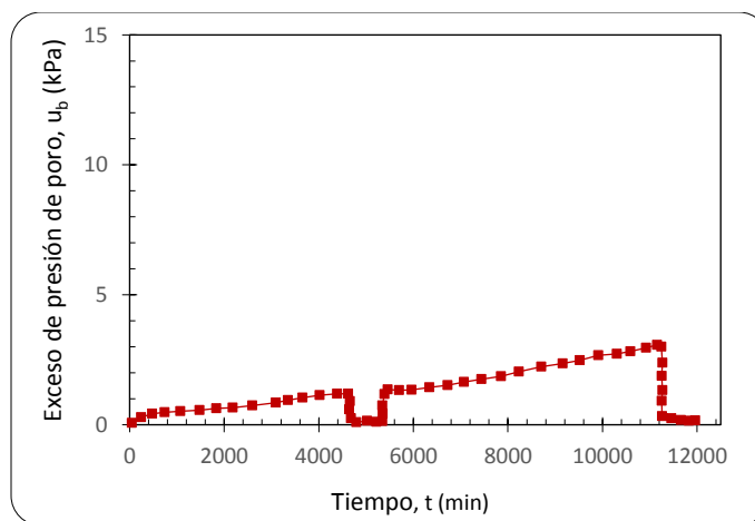
Figura 3.9 Registro de presión de poro en la prueba CRS
