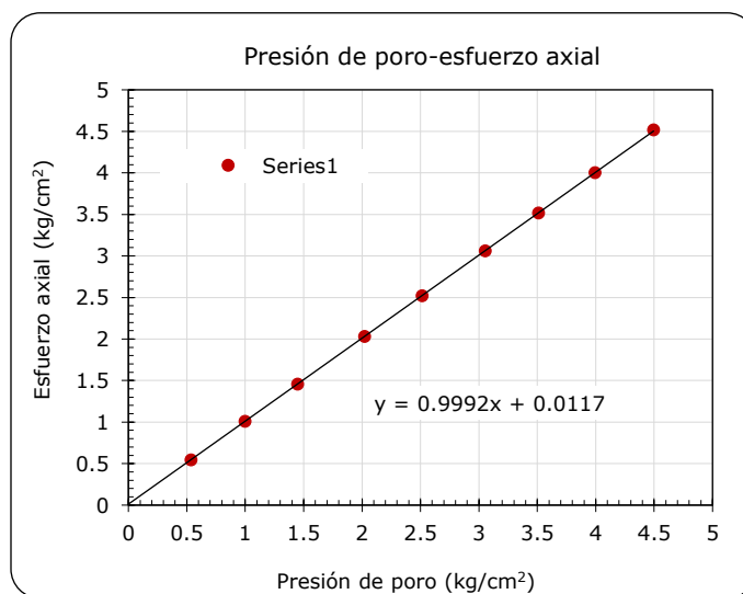
Figura 2.36 Verificación cruzada de presión de poro vs esfuerzo axial
