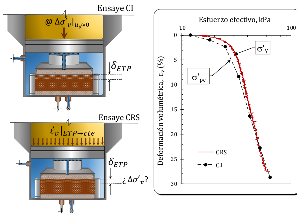
Figura 4.1 Esquema de prueba de CI y CRS
