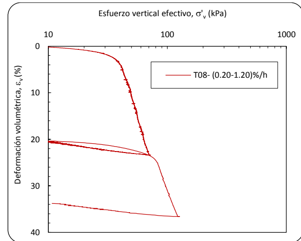
Figura B.43 Curva de compresibilidad, prueba T08
