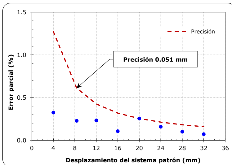
Figura 2.30 Curva de precisión del sensor de desplazamiento
