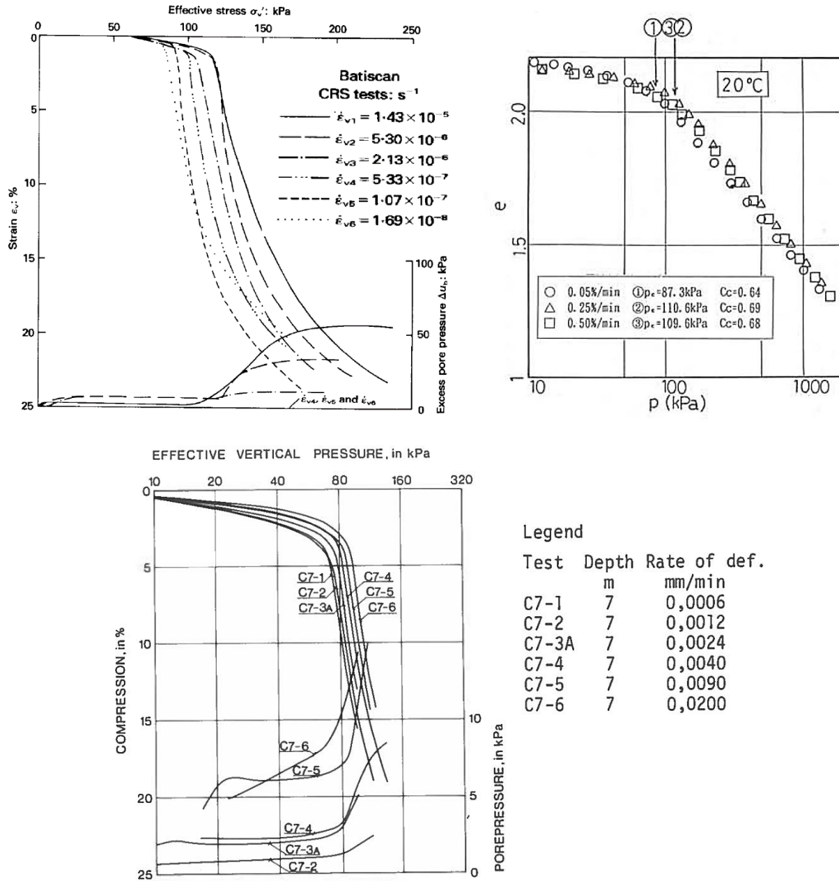
Figura 4.20 Curvas esfuerzo-deformación en pruebas CRS a diferentes velocidades para Leroueil et al. , 1985 (izquierda superior), Akagi et al. , 1995 (derecha superior) y Sällfors, 1975 (inferior).
