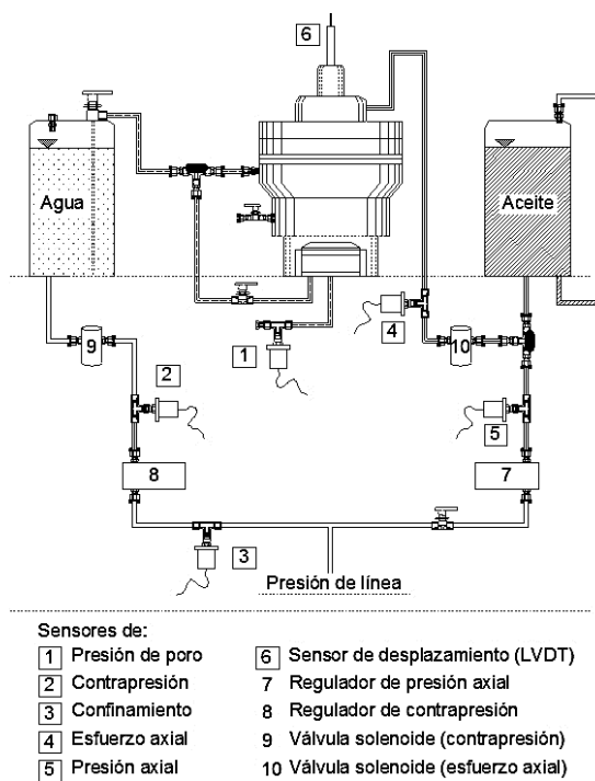
Figura 3.1 Esquema resumido de distribución de sensores del consolidómetro
