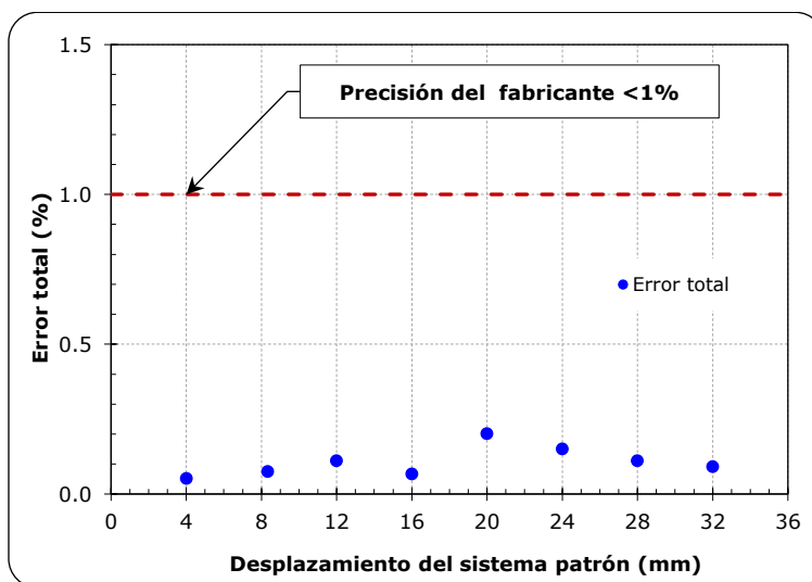
Figura 2.31 Curva de precisión del sensor de desplazamiento
