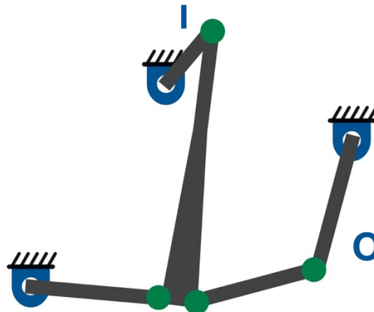
Figura 3.5. Mecanismo manivela-oscilador de seis barras.
