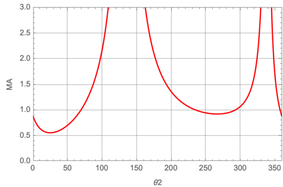
Figura 3.52. Ventaja mecánica MO4.
