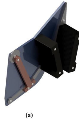
Figura 16 – Modelo en CAD de la configuración mecánica propuesta.
