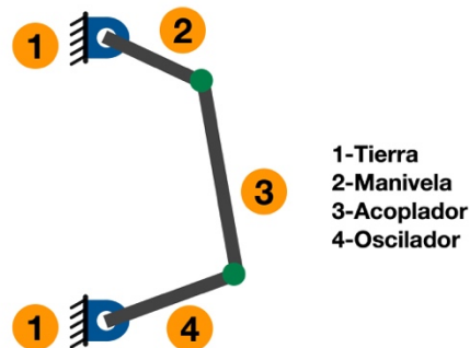
Figura 3.16. Números asignados a los eslabones para el análisis MO4-2.
