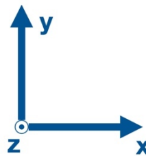
Figura. 2.6. Sistema coordenado rectangular derecho \hat{x}, \hat{y}, \hat{z}
