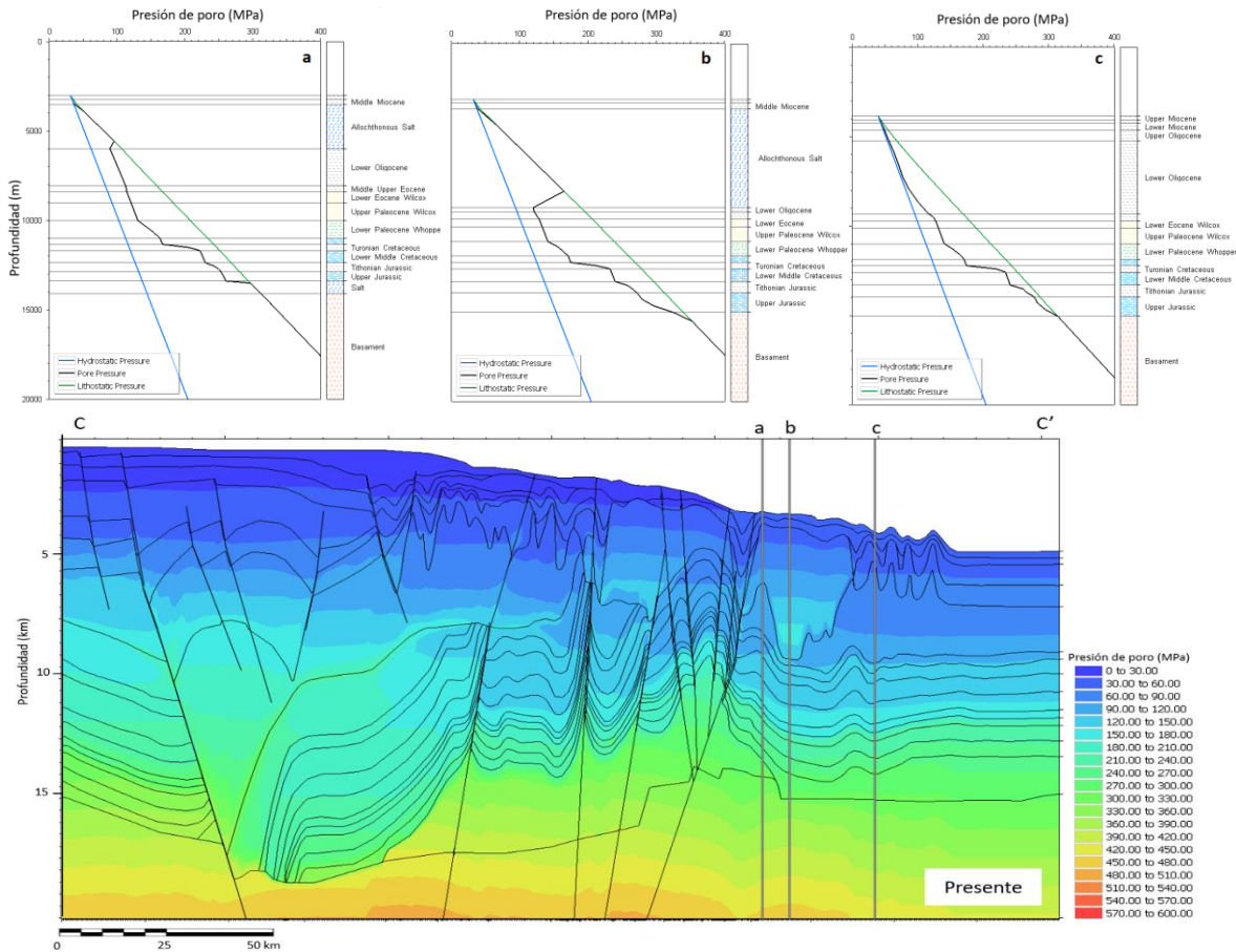
Figura 5.18 Extracciones 1D: a, b y c de presión de poro a lo largo de la sección C-C'. Las extracciones a y b atraviesan la sal, mientras que la c, no, esto con el objetivo de visualizar como es la tendencia de presión de poro con y sin presencia de sal.
