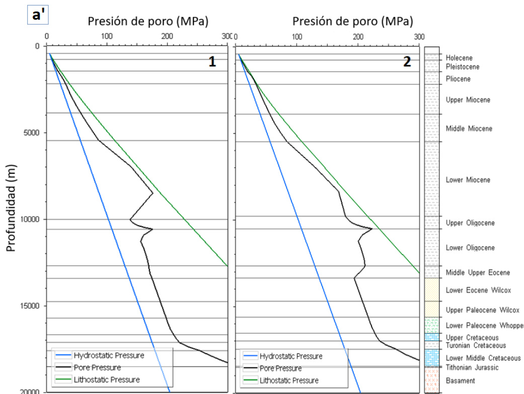
Figura 5.15 Escenario 1 y 2, extracción a', la tendencia de presión de poro es muy similar, sin embargo, algunos valores cambian significativamente debido al tipo de fallas.
