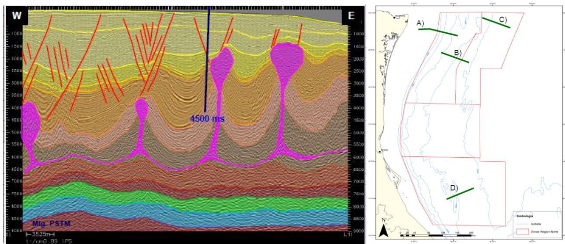
Figura 2.5 Sección A-A', que cruza perpendicularmente al Cinturón subsalino, a la derecha un mapa del Golfo de México oeste y secciones (Tomada de CNH, 2015).
