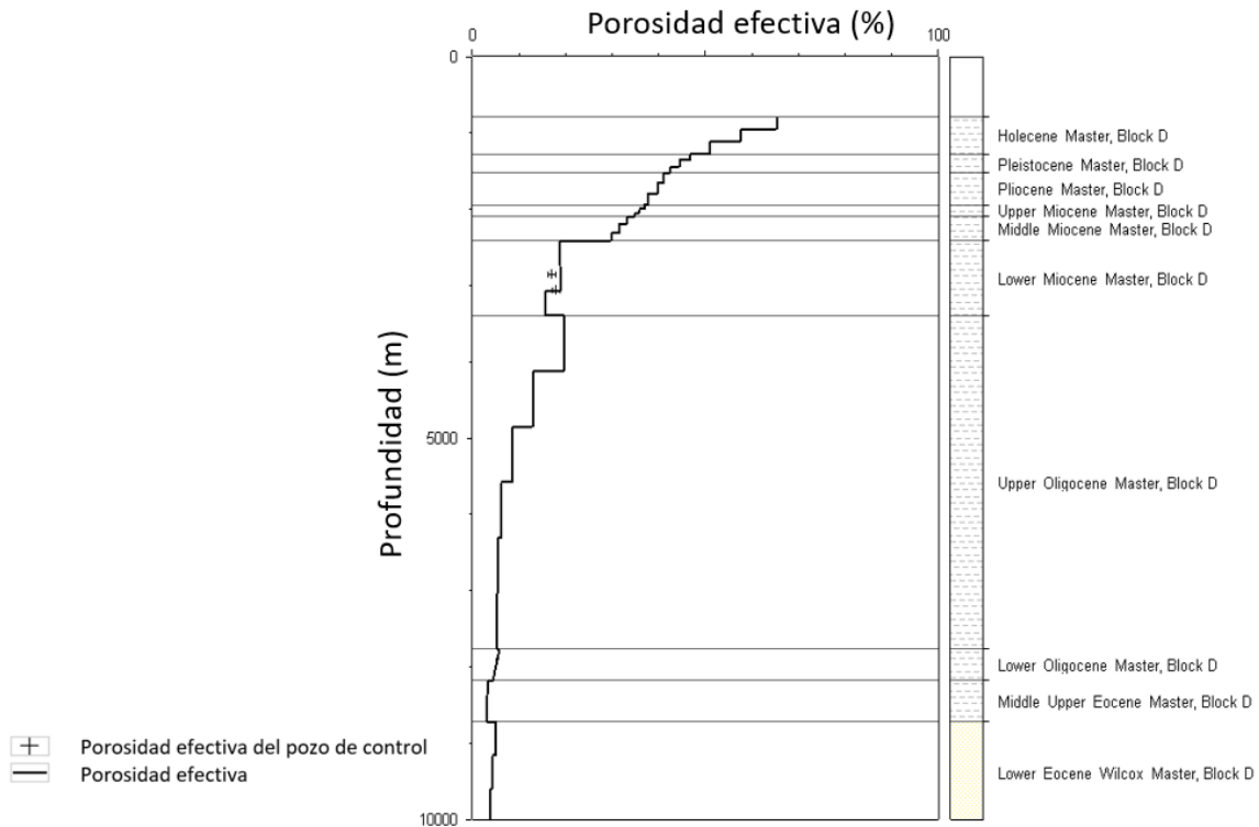
Figura 4.20 Resultado de la calibración de porosidad efectiva.
