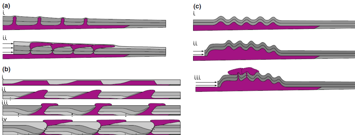
Figura 2.6 Diagramas esquemáticos de diferentes conceptos sobre la evolución para un canopie (a) mecanismo de diapiro exprimido (b) mecanismo rollover expulsión (c) mecanismo de anticlinal roto. El acotamiento es esencial para las tres primeras etapas. Los puntos negros marcan los puntos de inicio de la sal (Tomada de Gradmann y Beaumont, 2016).
