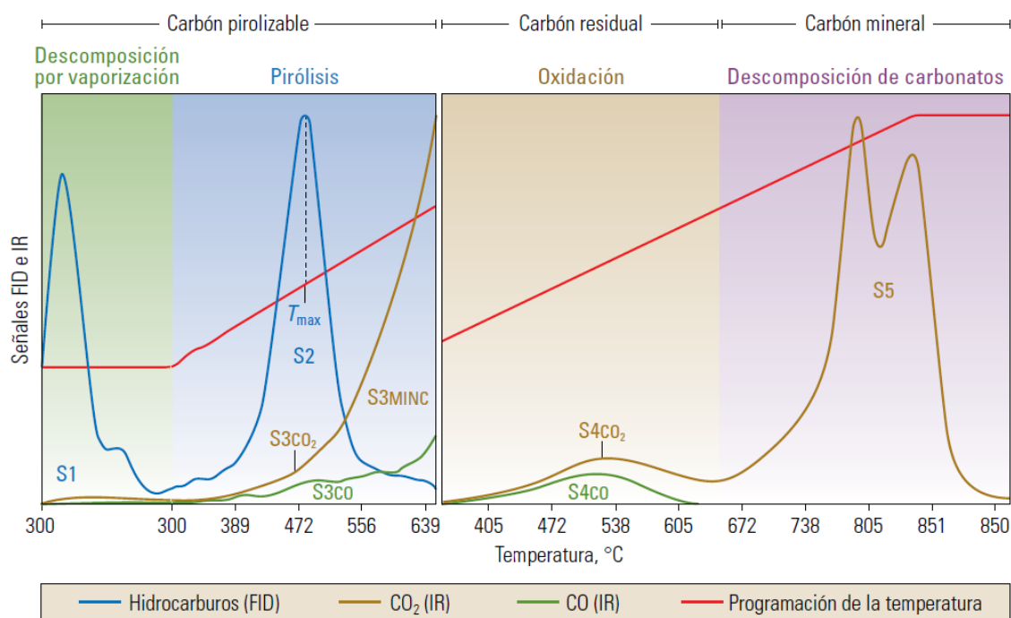
Figura 3.2. Resultado del proceso programado de pirólisis, en el cual es posible observar los picos S1, S2, S3, S4, S5 y T_{max} , los resultados del proceso de pirólisis se computan para determinar los volúmenes de carbón pirolizable, carbón residual, carbón mineral y COT (Tomada de McCarthy et al., 2011).
