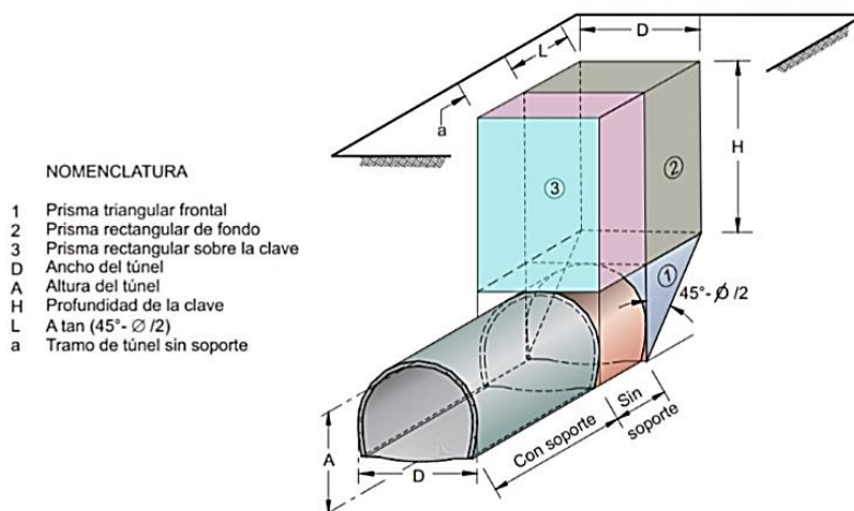
Figura 38. Tamez et al. (1997). Mecanismo de falla simplificado. [Figura]. Recuperado de Sistemas de Presostenimiento para Túneles en Terreno Dificiles.
