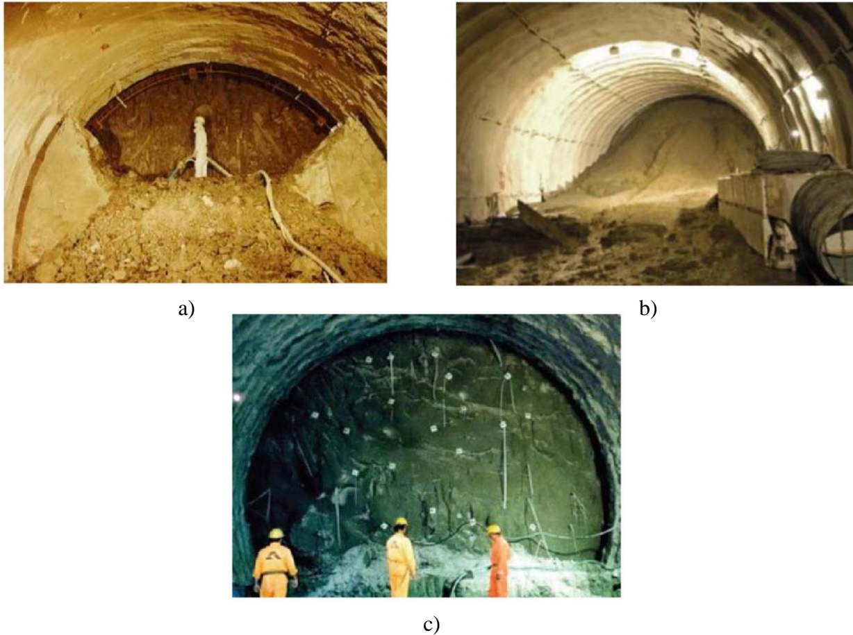
Figura 10. Anagnostou et al. (2018). (a) Frente de excavación en suelo con baja permeabilidad, (b) falla de frente en túnel y (c) sistema de soporte implementado. Recuperadas de ETH Zürich De acuerdo con el método de construcción empleado, las secuencias de excavación y el soporte temporal de un túnel, existen otros mecanismos de falla por influencia del agua que deben considerarse durante el diseño de un túnel, según los trabajos de Anagnostou (2006), son; falla por frente expuesto; subsidencia en superficie; sobreesfuerzos en zona de falla; presión de squeezing o deformaciones y levantamiento de piso en el túnel. (Fig. 11).
