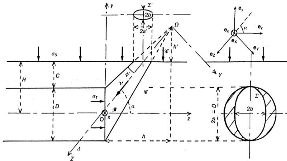
Figura 32. Villafuerte, D. (2013). Mecanismo de falla tipo MI de Leca & Dormieux, 1990. [Figura]. Recuperado de Estudio Analítico y Numérico del Fenómeno de Inestabilidad de Frente en Túneles.
