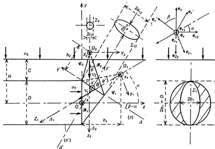
Figura 33. Leca (1990). Mecanismo de falla tipo MII. [Figura]. Recuperado de Estudio Analítico y Numérico del Fenómeno de Inestabilidad de Frente en Túneles.
