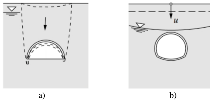
Figura 10. Anagnostou et al. (2018). (a) Frente de excavación en suelo con baja permeabilidad, (b) falla de frente en túnel y (c) sistema de soporte implementado. Recuperadas de ETH Zürich De acuerdo con el método de construcción empleado, las secuencias de excavación y el soporte temporal de un túnel, existen otros mecanismos de falla por influencia del agua que deben considerarse durante el diseño de un túnel, según los trabajos de Anagnostou (2006), son; falla por frente expuesto; subsidencia en superficie; sobreesfuerzos en zona de falla; presión de squeezing o deformaciones y levantamiento de piso en el túnel. (Fig. 11).
