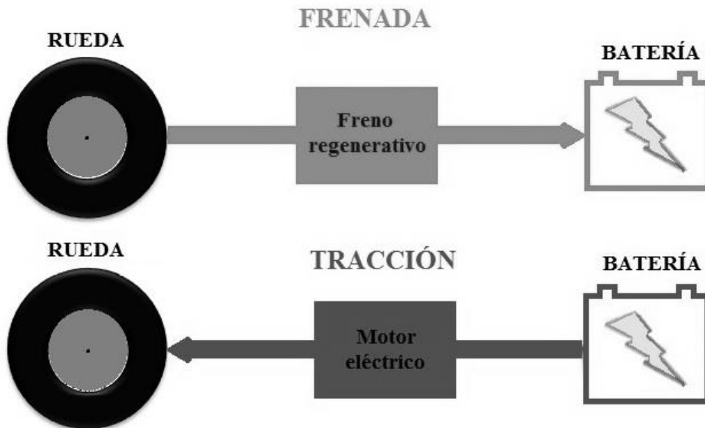
Figura 8.1c. Frenos regenerativos
