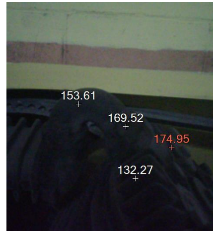
Figura 27. Distribución de temperaturas en la región más caliente del cabezal (Termografía)
