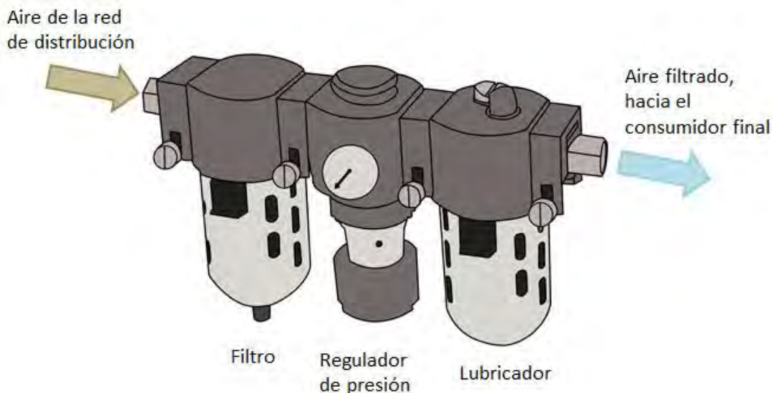
Figura 14. Unidad de mantenimiento con filtro, regulador y lubricador. Elaboración propia.
