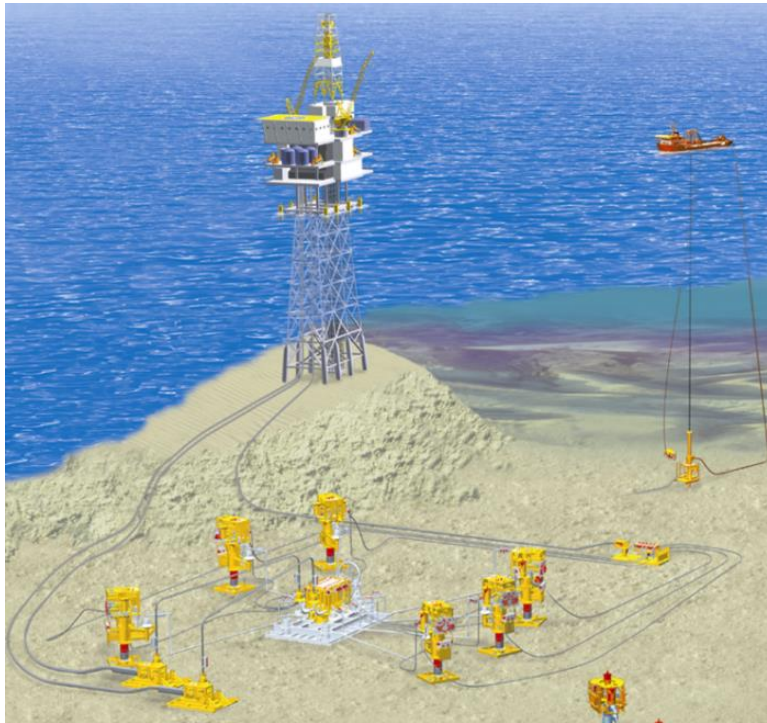
Fig. 3.5 Conexión de árboles submarinos (Schlumberger-Cameron) 43
