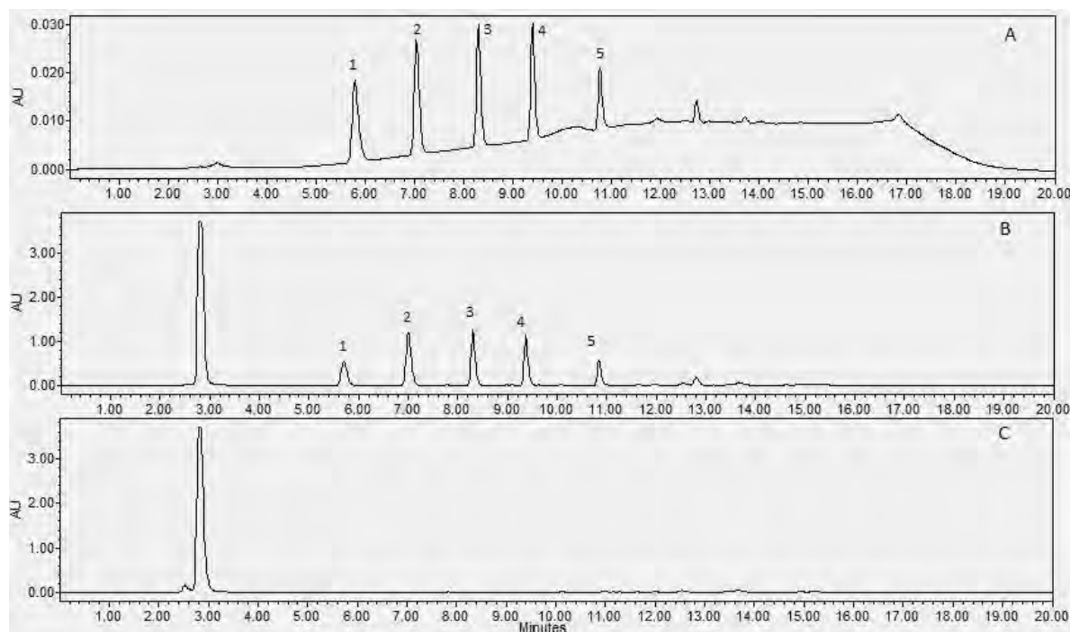
Figura 11. Cromatogramas obtenidos con las condiciones óptimas para el sistema EFS-HPLC-UV a 254 nm. (A) Disolución estándar a 4 \text{ ng mL}^{-1} (B) muestra fortificada a 100 \text{ ng g}^{-1} y (C) muestra blanco. 1. Metilparabeno, 2. Etilparabeno, 3. Propilparabeno, 4. Butilparabeno y 5. Oxibenzona.
