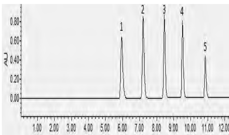
Figura 10. Cromatograma obtenido de una disolución estándar a una concentración de 200 ppb. Compuestos: 1. MP, 2. EP, 3. PP, 4. BP y 5. BP-3.
