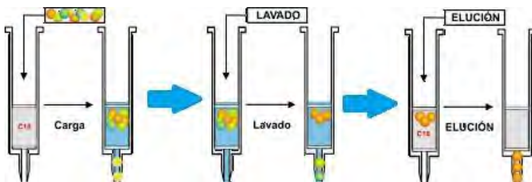
Figura 4. Procedimiento general de la EFS. Esquema adaptado de CromLab S.L. [37].
